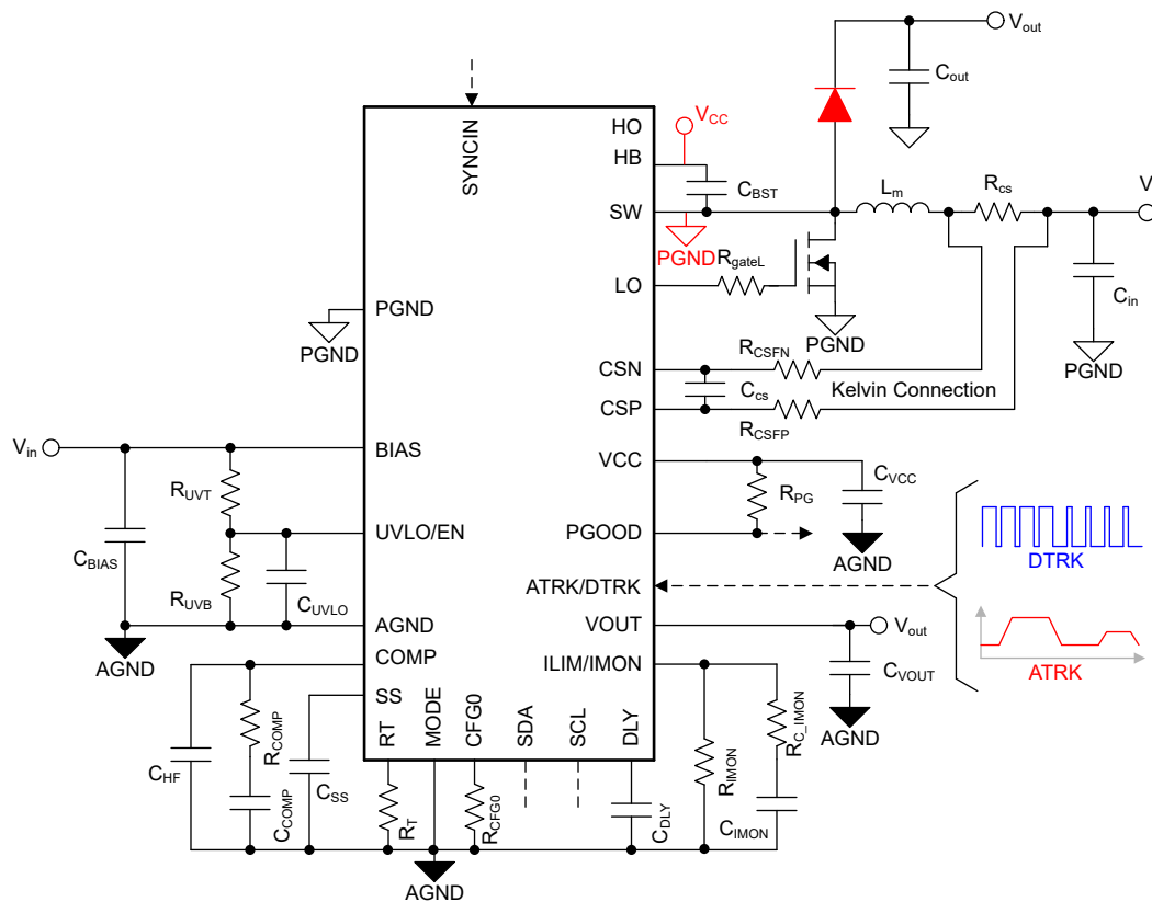
图 8-5. 非同步升压转换器的原理图
