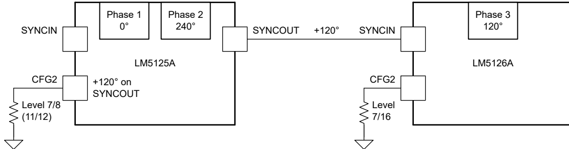
图 8-2. 三相交错式升压配置
