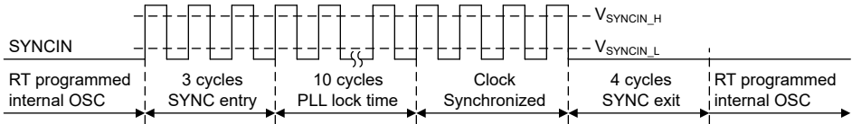
图 6-6. 时钟同步
