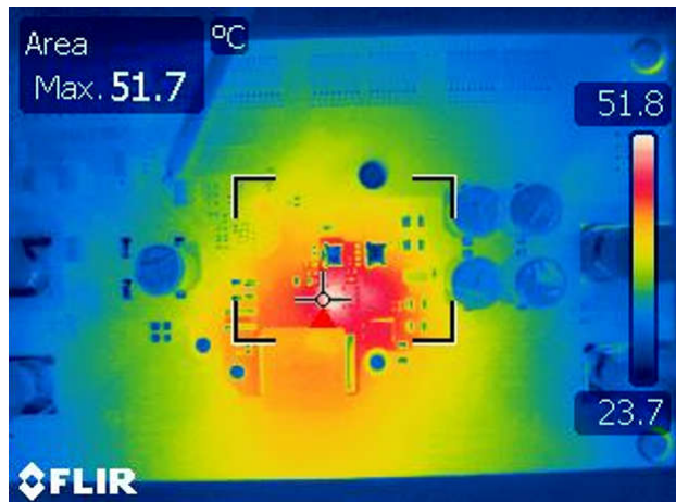
图 8-19. V_{in} = 14.4V , V_{out} = 24V , P_{OUT} = 150W , 自然对流
