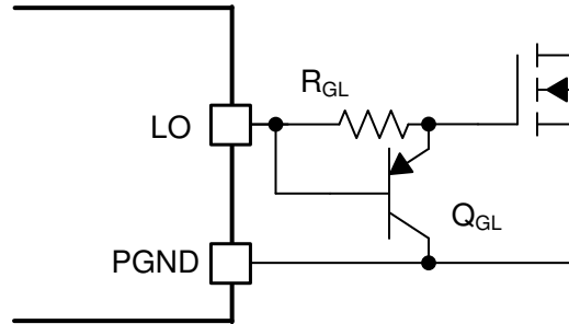
图 6-23. 压摆率控制
