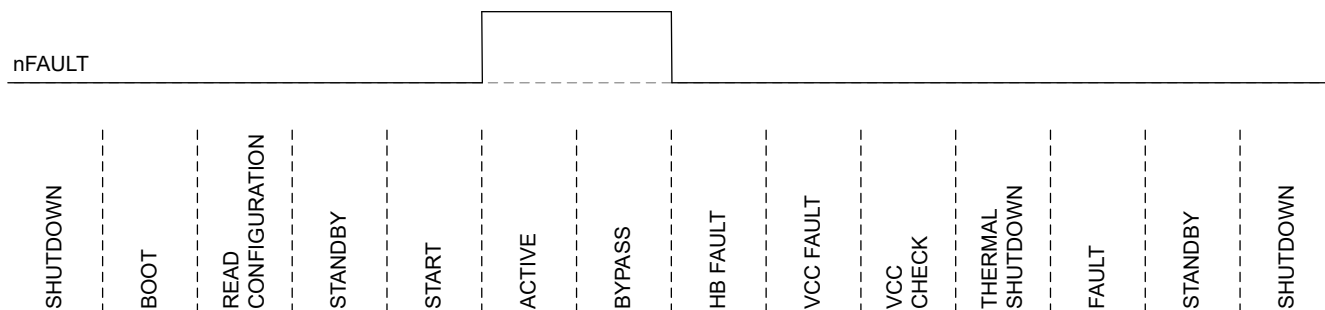
图 6-16. 所有器件状态的 nFAULT 状态
