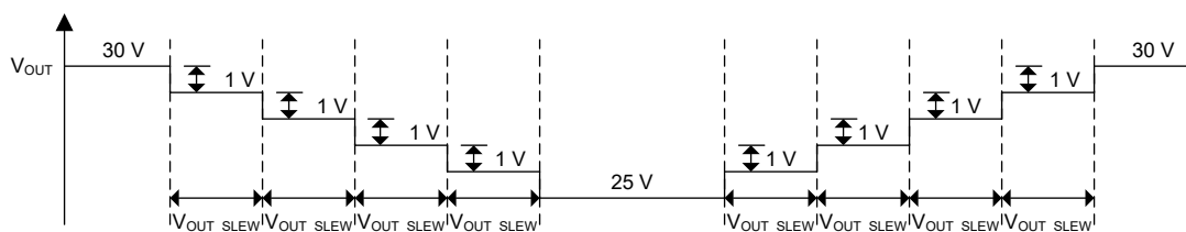
图 6-24. V_{OUT} 编程示例 30V 至 25V 至 30V
