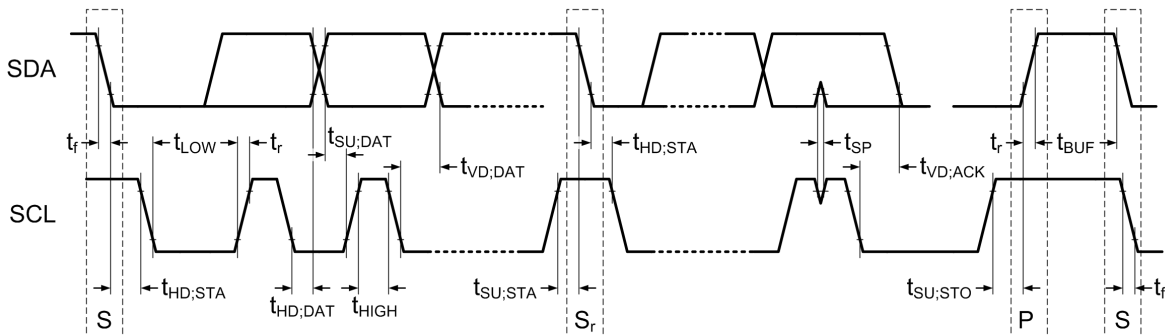
图 6-27. I 2 C 数据传输时序
