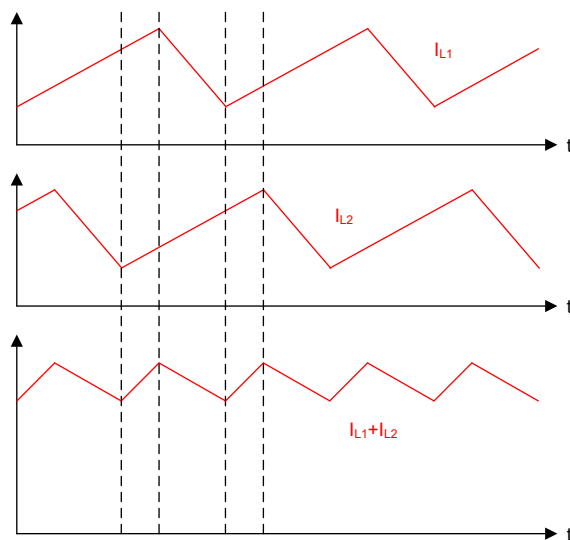
图 8-7. 通过双相交错降低输入电流纹波
