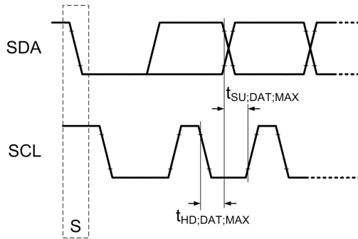
图 6-28. 最长上升/下降时间的 I 2 C 数据传输时序
