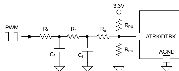
图 8-9. 两级 RC 滤波器连接到 ATRK/DTRK
