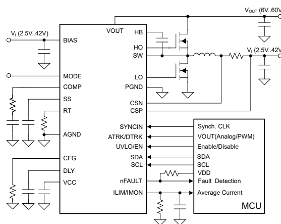
典型应用
