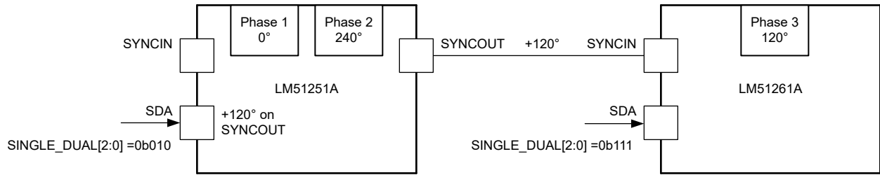
图 6-4. 三相配置
