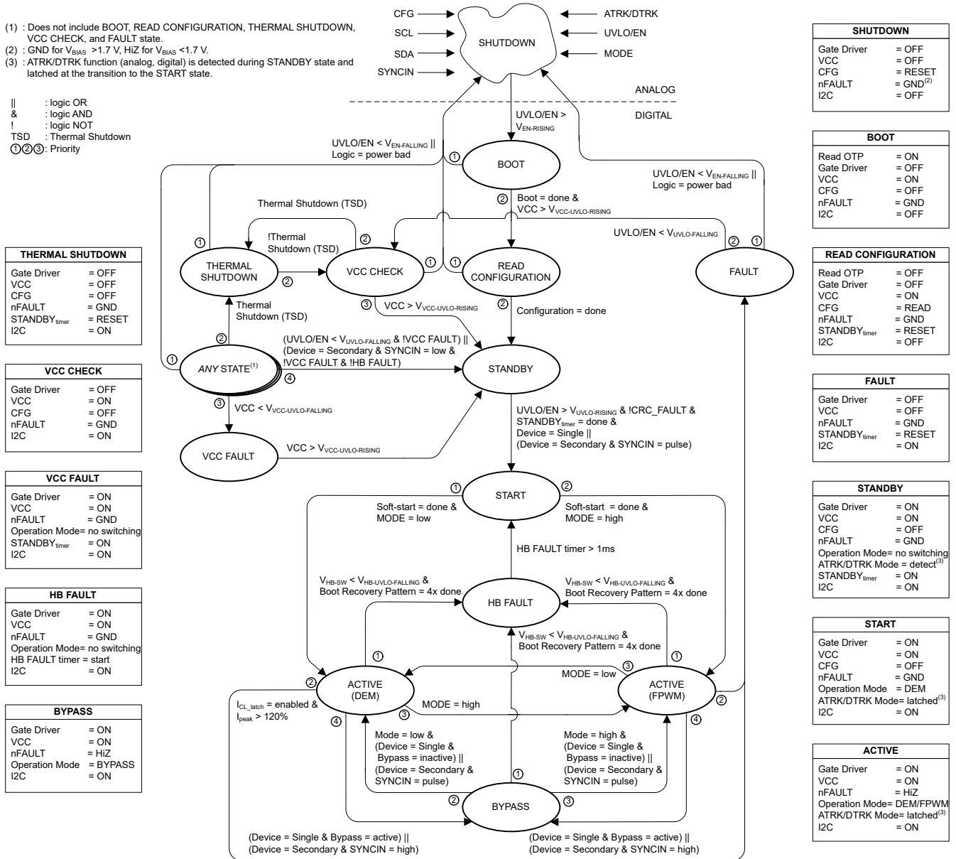
图 6-25. 功能状态图
