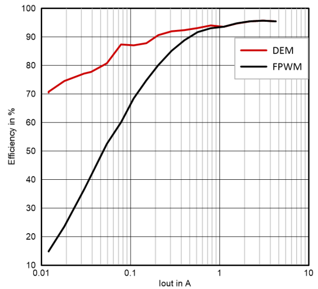
图 8-12. 效率与输出电流间的关系, V_{in} = 14.4V , V_{out} = 45V
