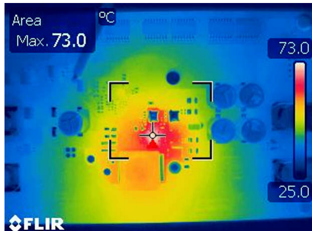
图 8-20. V_{in} = 14.4V , V_{out} = 45V , P_{OUT} = 150W , 自然对流
