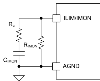
图 8-10. ILIM/IMON 引脚配置
