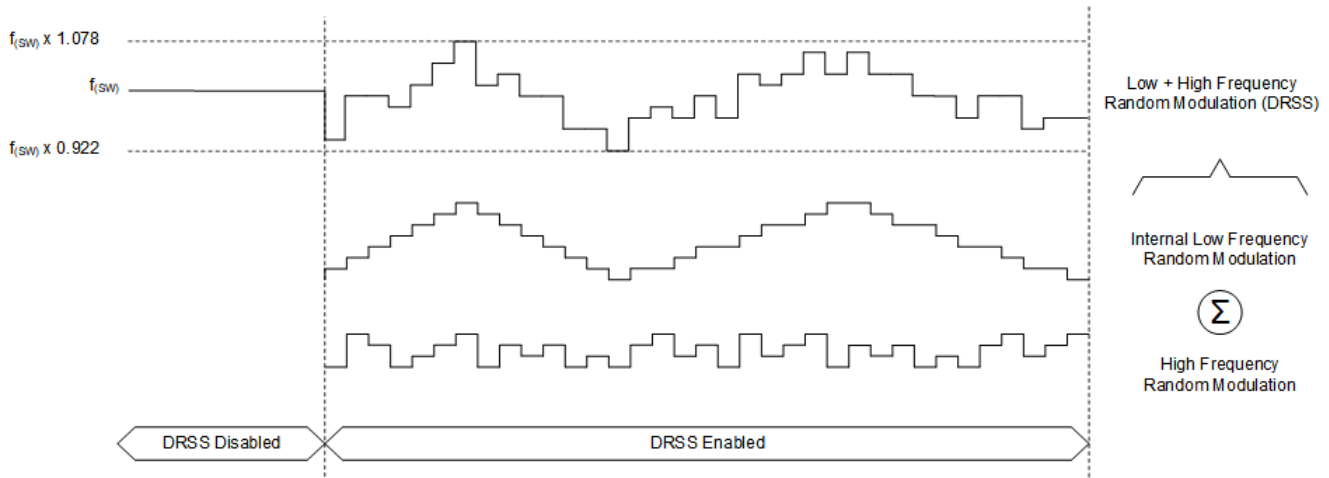
图 6-7. 双随机展频
