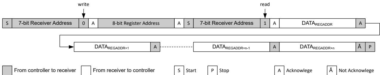
图 6-30. 从定义的寄存器地址开始进行顺序读取
