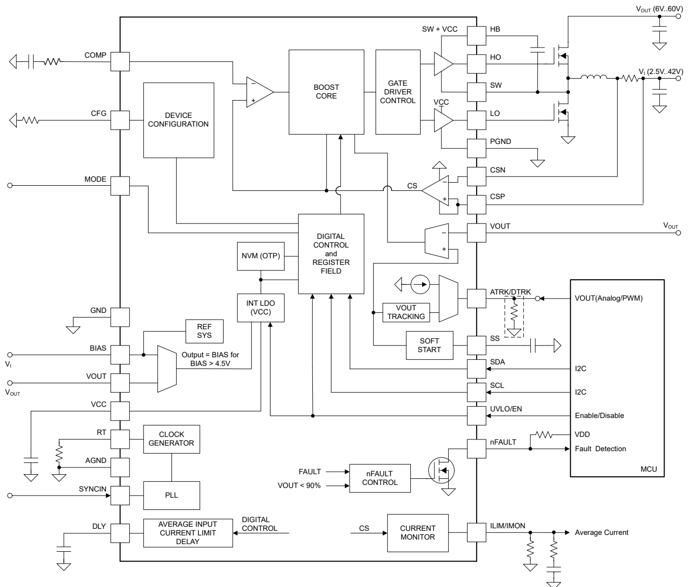
图 6-1. 功能方框图
