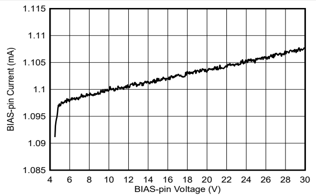
图 5-6. BIAS 引脚电流与 BIAS 引脚电压间的关系 ( 活动 , FPWM )
