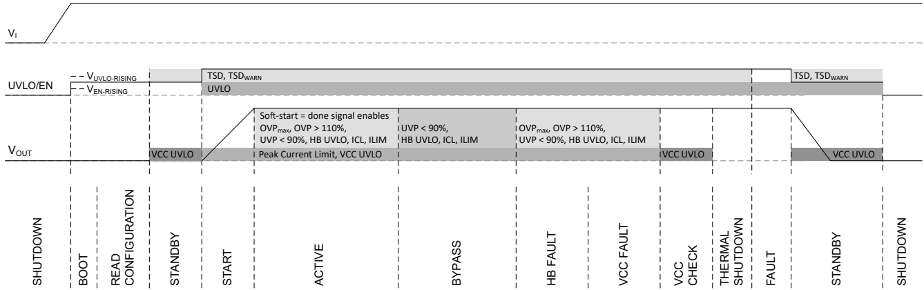
图 6-15. 保护功能
