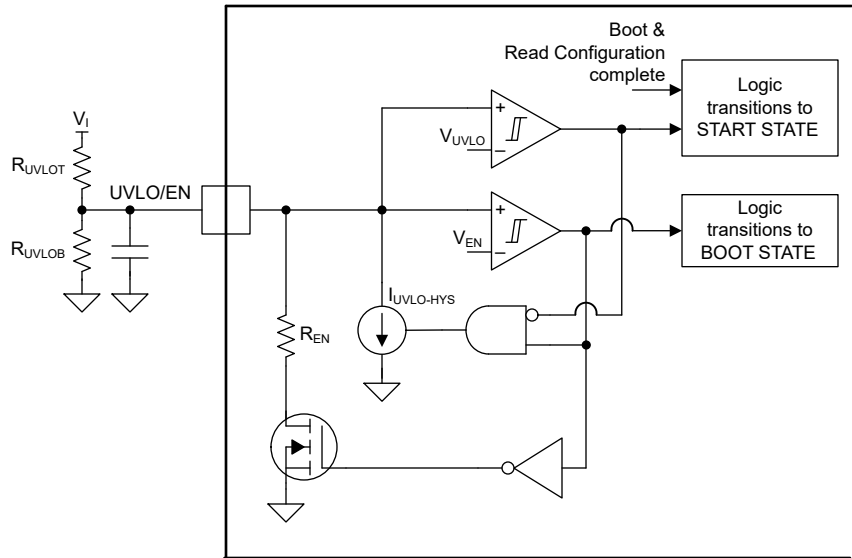
图 6-2. 功能方框图 UVLO 和 EN
