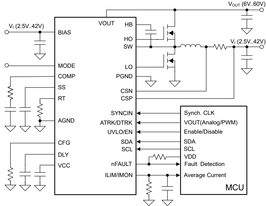
图 8-6. 典型应用
