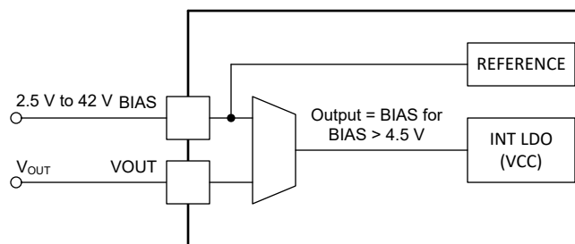
图 6-10. 动态 BIAS 电源选择
