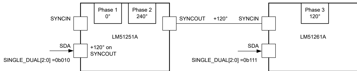
图 8-3. 三相交错式升压配置
