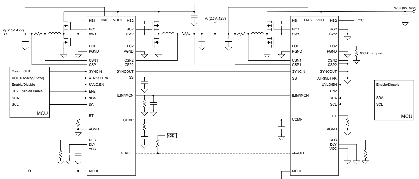
图 8-4. 三相典型应用原理图
