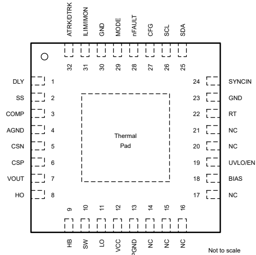
图 4-1. LM51261A-Q1 RHB 封装，32 引脚 VQFN ( 顶视图 )
