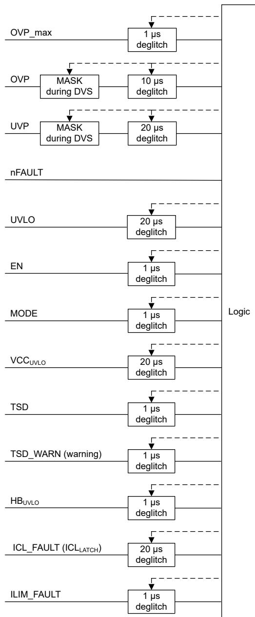
图 6-22. 信号抗尖峰脉冲
