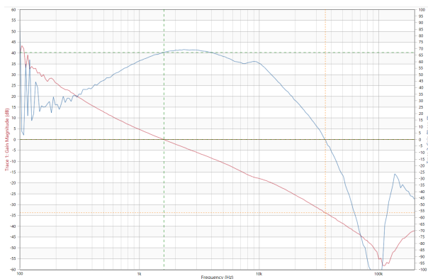
图 8-18. 波特图、 V_{in}=14.4V 、 V_{out}=45V 、 I_{out}=3.4A ( 平均电流环路已禁用 )
