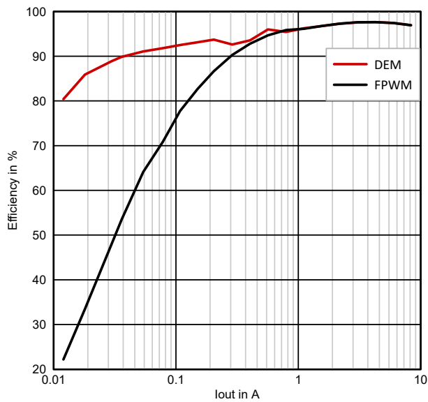
图 8-11. 效率与输出电流间的关系, V_{in} = 14.4V , V_{out} = 24V
