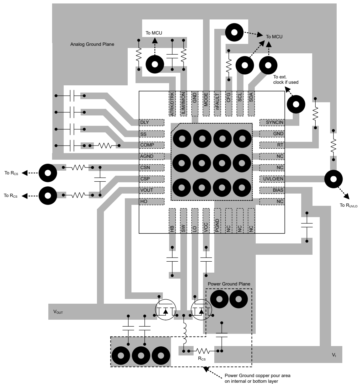
图 8-21. 布局示例
