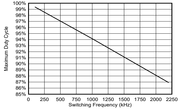
图 5-8. 最大占空比与开关频率间的关系
