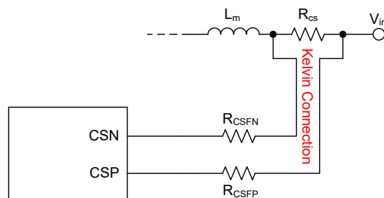
图 8-8. 电流检测滤波器
