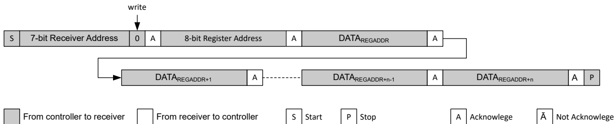
图 6-32. 在定义的寄存器地址开始进行顺序写入
