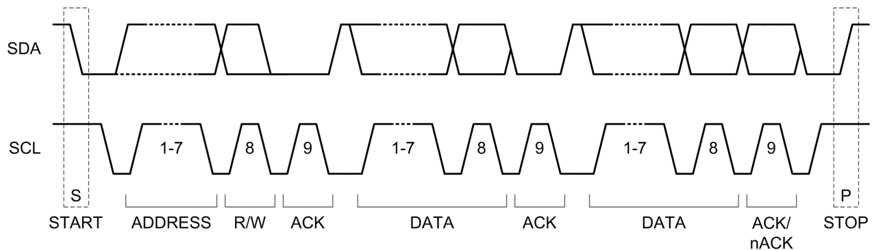
图 6-26. I 2 C 启动/停止/确认协议
