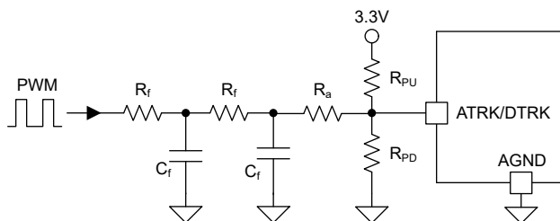
图 7-8. 两级 RC 滤波器连接到 ATRK/DTRK
