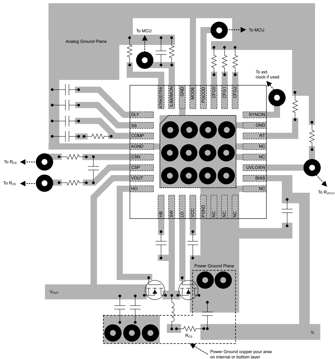
图 7-20. 布局示例
