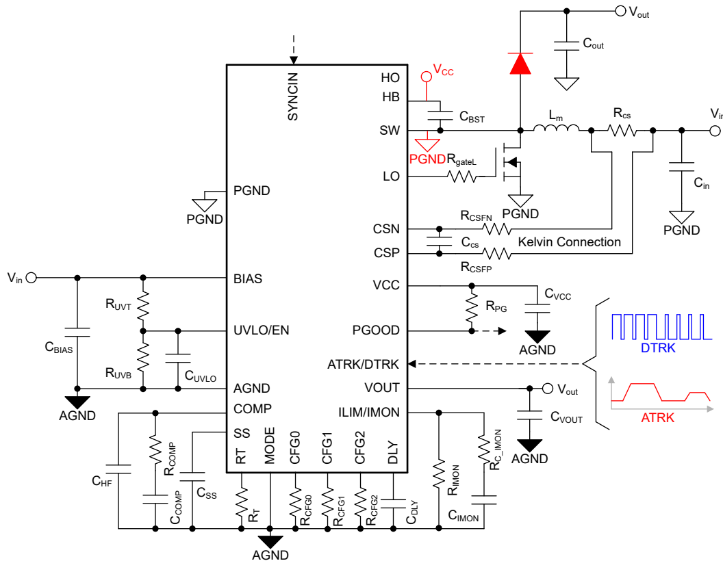
图 7-4. 非同步升压转换器的原理图
