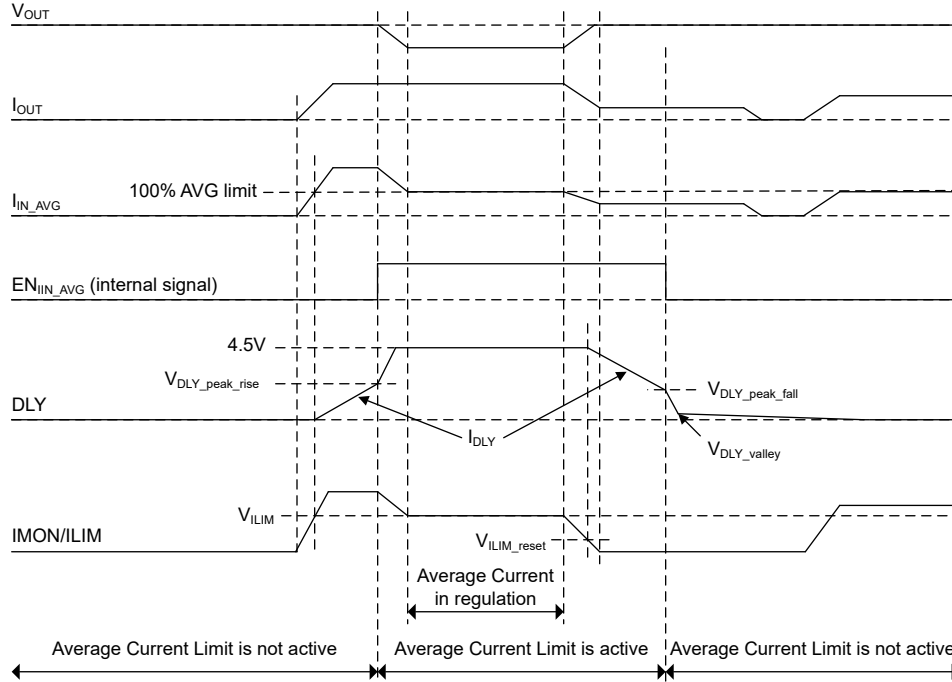
图 6-20. 平均电流限值
