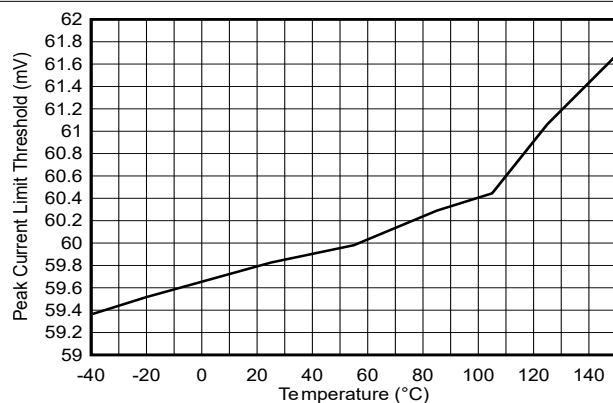
图 5-7. 峰值电流限制阈值 V_{\text{CLTH}} 与温度间的关系
