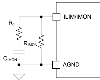
图 7-9. ILIM/IMON 引脚配置
