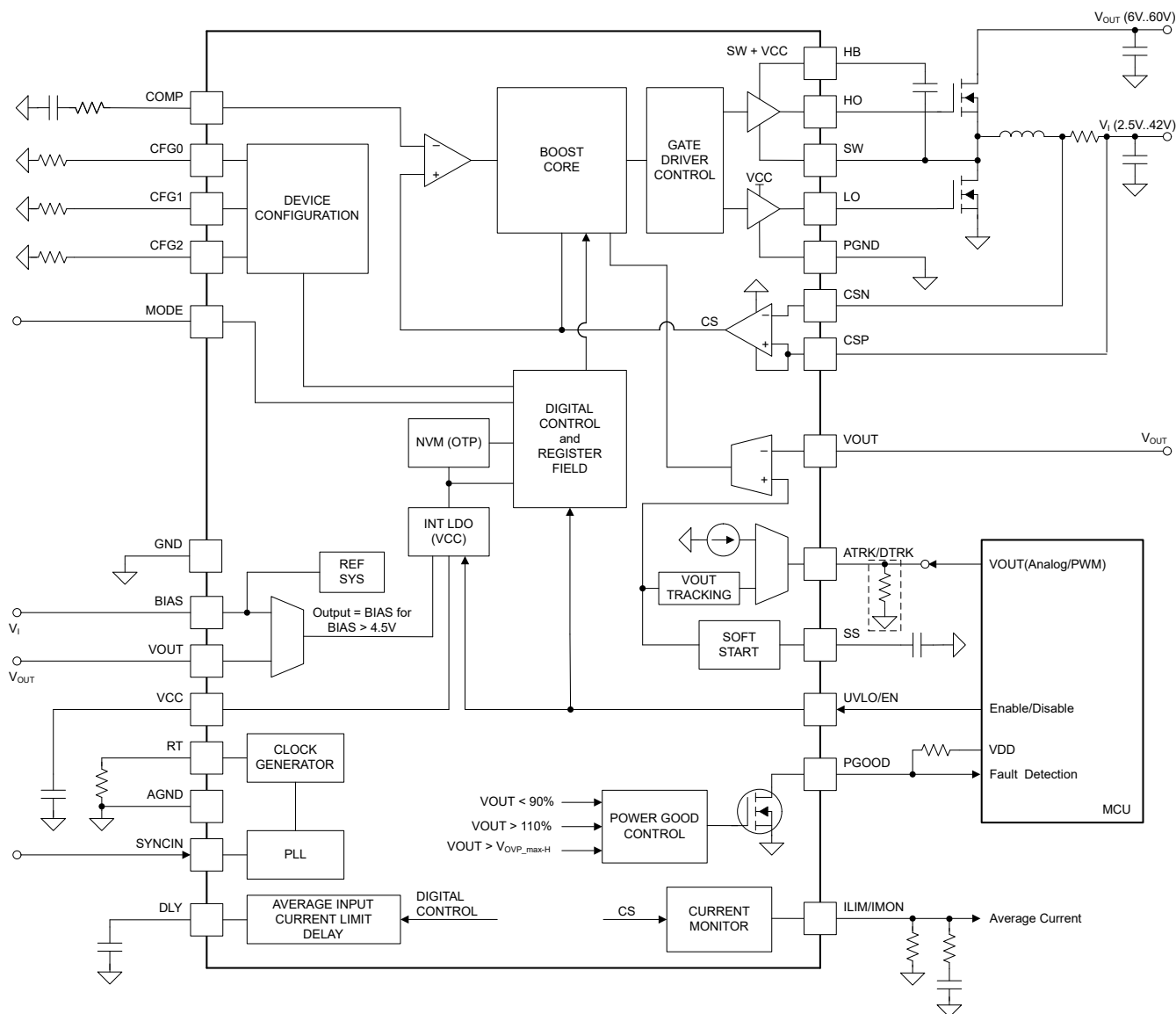
图 6-1. 功能方框图
