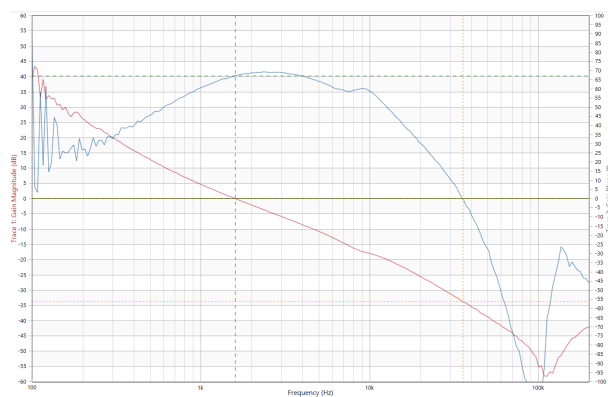
图 7-17. 波特图、 V_{in}=14.4V 、 V_{out}=45V 、 I_{out}=3.4A (平均电流环路已禁用)
