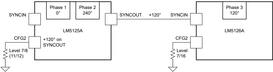
图 6-4. 三相配置
