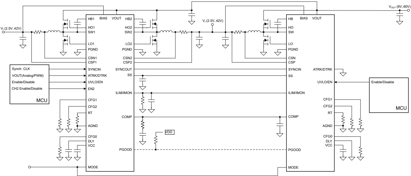
图 6-5. 典型应用 - 三相运行
