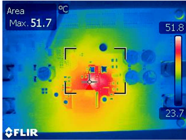
图 7-18. V_{in} = 14.4V , V_{out} = 24V , P_{OUT} = 150W , 自然对流
