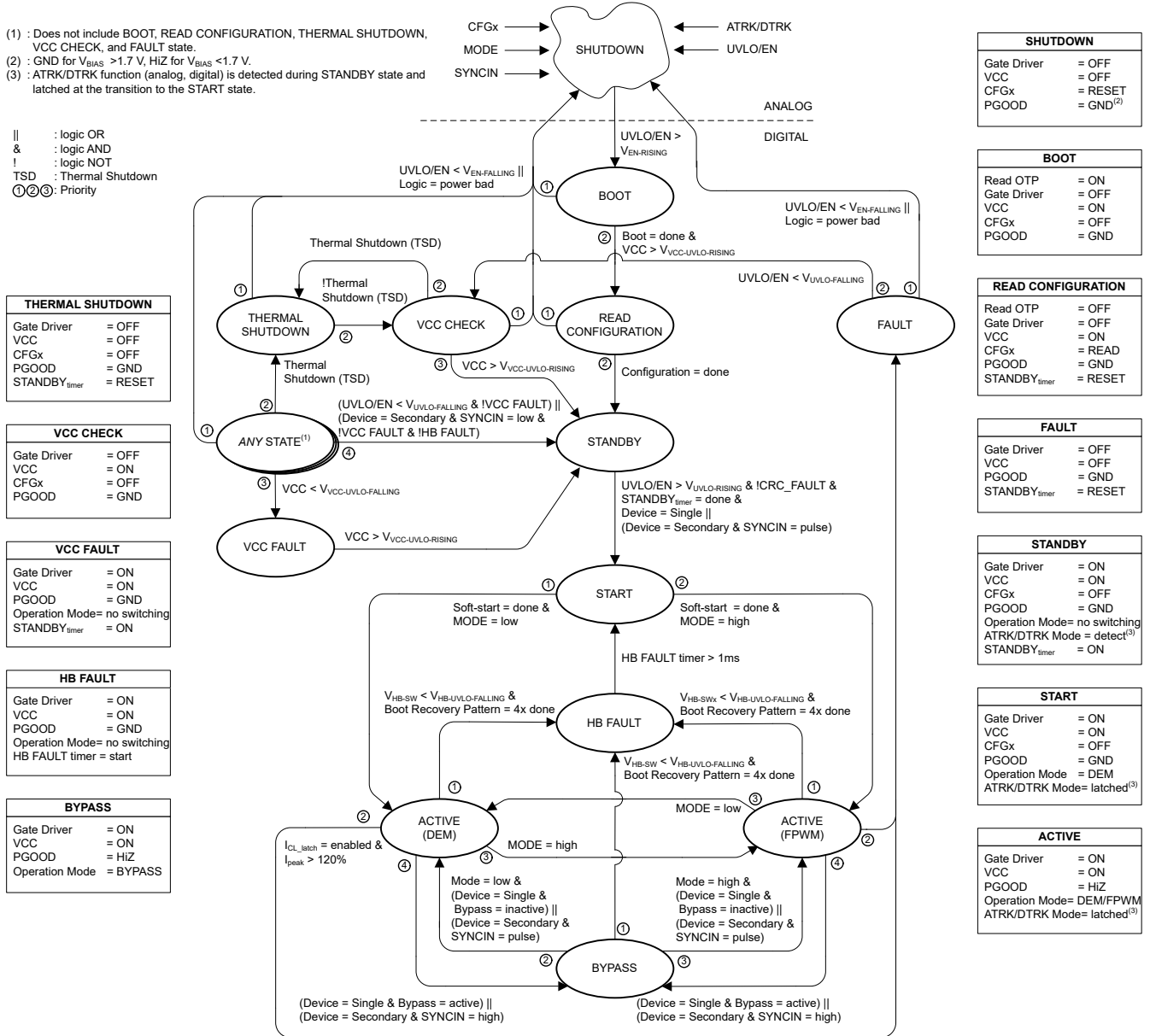
图 6-24. 功能状态图
