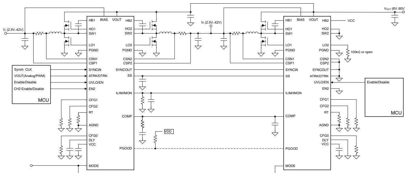
图 7-3. 三相典型应用原理图
