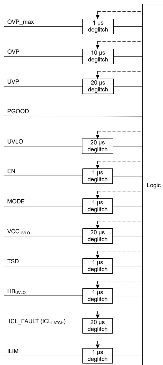
图 6-22. 信号抗尖峰脉冲
