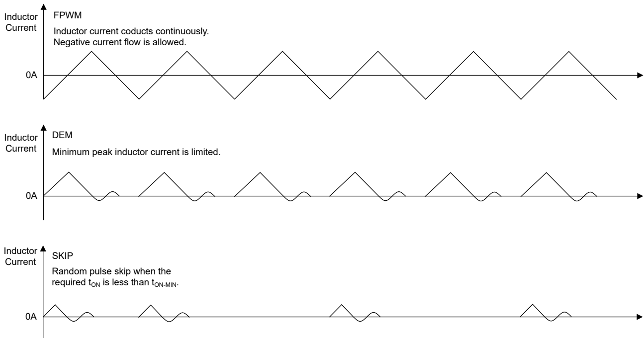
图 6-8. 不同工作模式下的电感器电流波形
