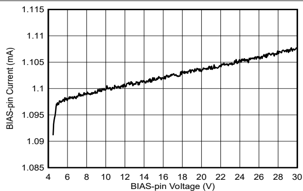
图 5-6. BIAS 引脚电流与 BIAS 引脚电压间的关系 ( 活动 , FPWM )
