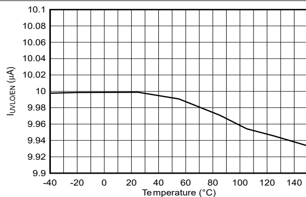
图 5-13. UVLO/EN 引脚电流与温度间的关系
