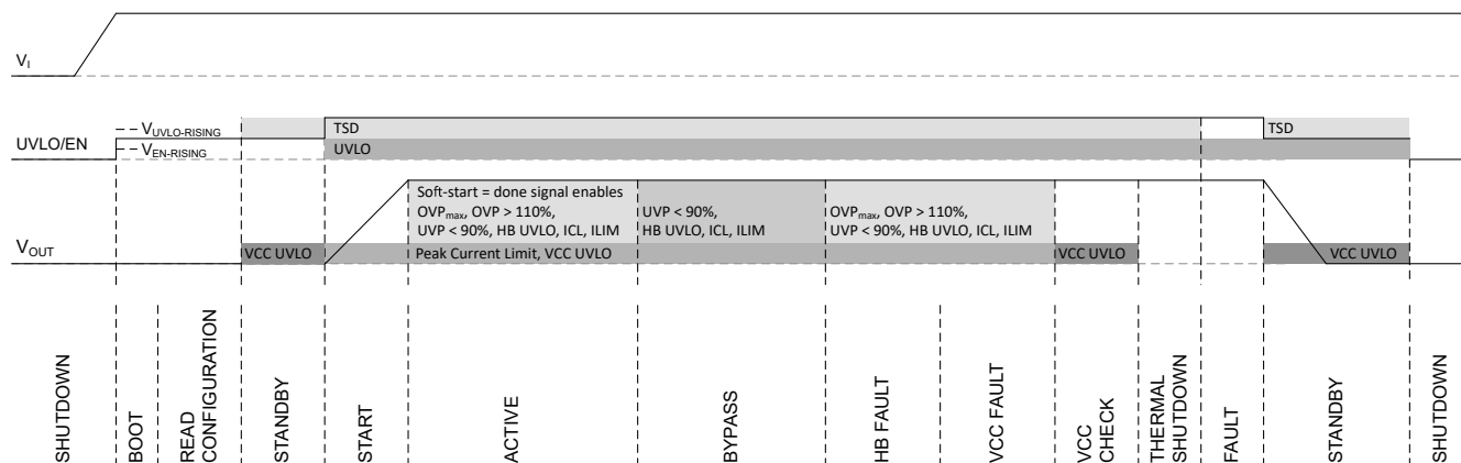
图 6-15. 保护功能
