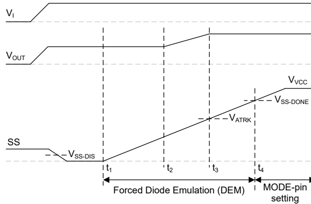
图 6-11. 软启动
