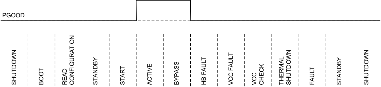
图 6-16. 所有器件状态的 PGOOD 状态
