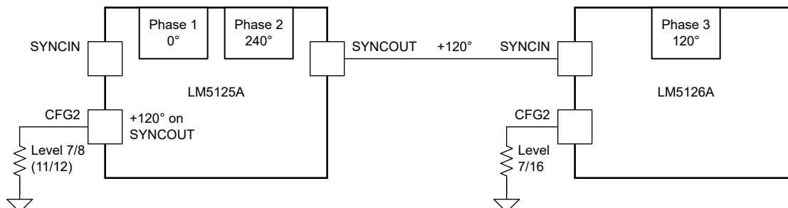
图 7-2. 三相交错式升压配置
