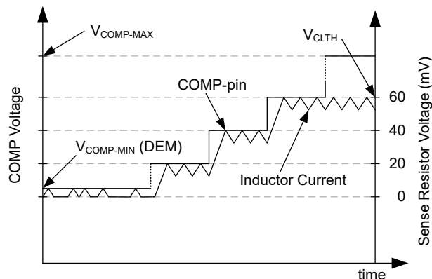
图 6-18. 通过 COMP 引脚电压和感测电阻电压限制开关电流 (DEM)
