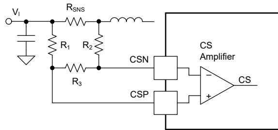
图 6-17. 通过添加电阻器进行峰值限制调整
