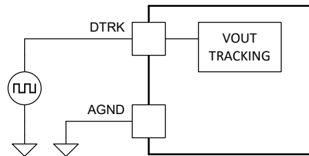
图 6-14. 通过数字信号进行 V_{OUT} 跟踪
