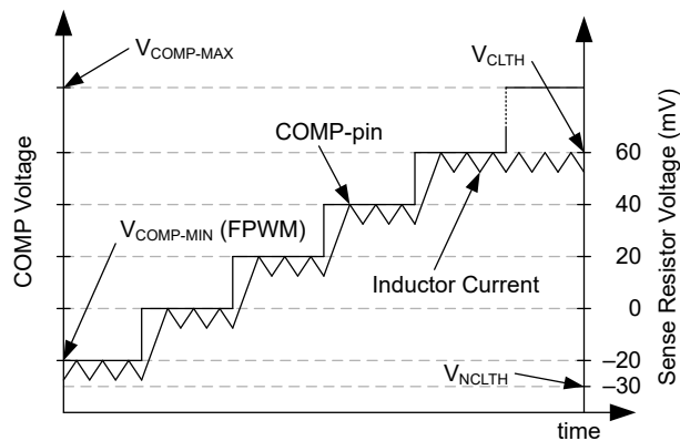
图 6-19. 通过 COMP 引脚电压和感测电阻电压限制开关电流 (FPWM)
