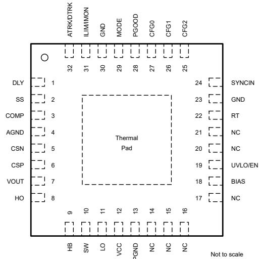
图 4-1. LM5126A-Q1 RHB 封装，32 引脚 VQFN (顶视图)
