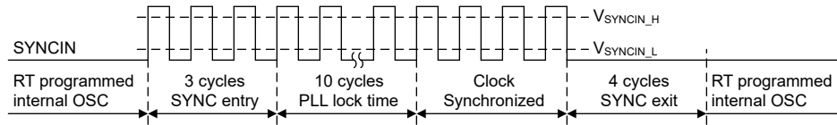
图 6-6. 时钟同步
