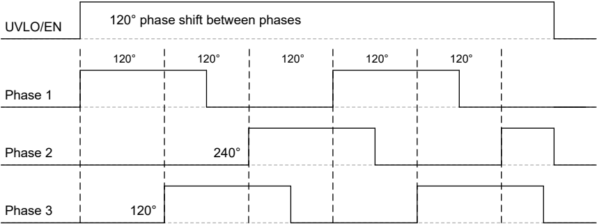
图 6-3. 双器件三相运行
