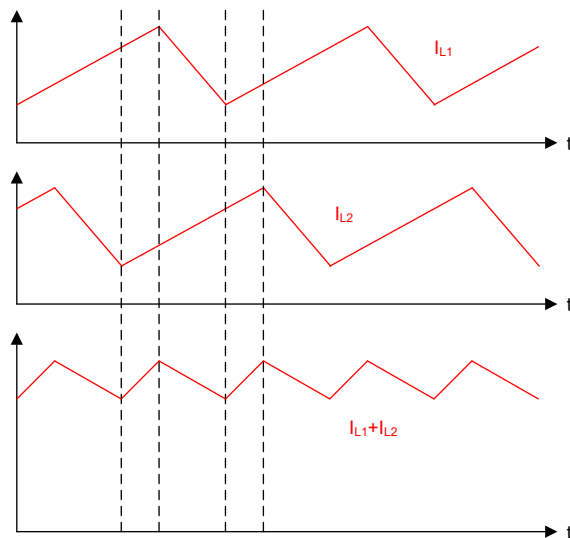
图 7-6. 通过双相交错降低输入电流纹波
