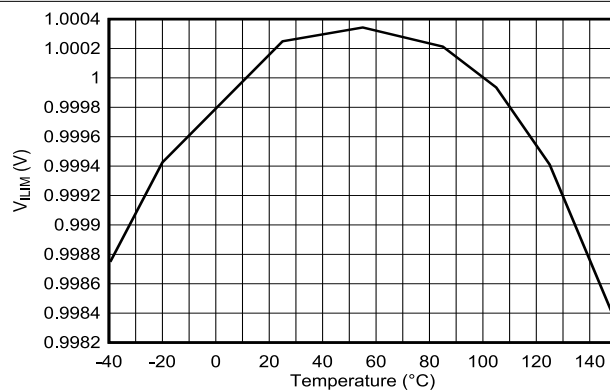
图 5-14. 平均电流限制调节电压与温度间的关系
