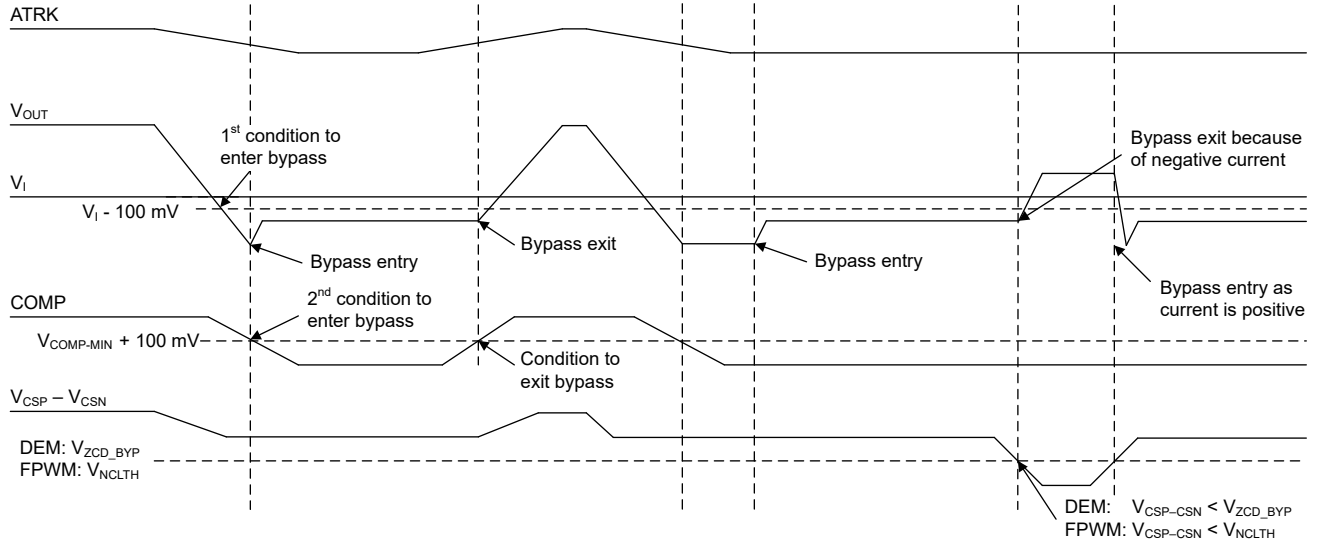
图 6-9. 进入、退出旁路模式
