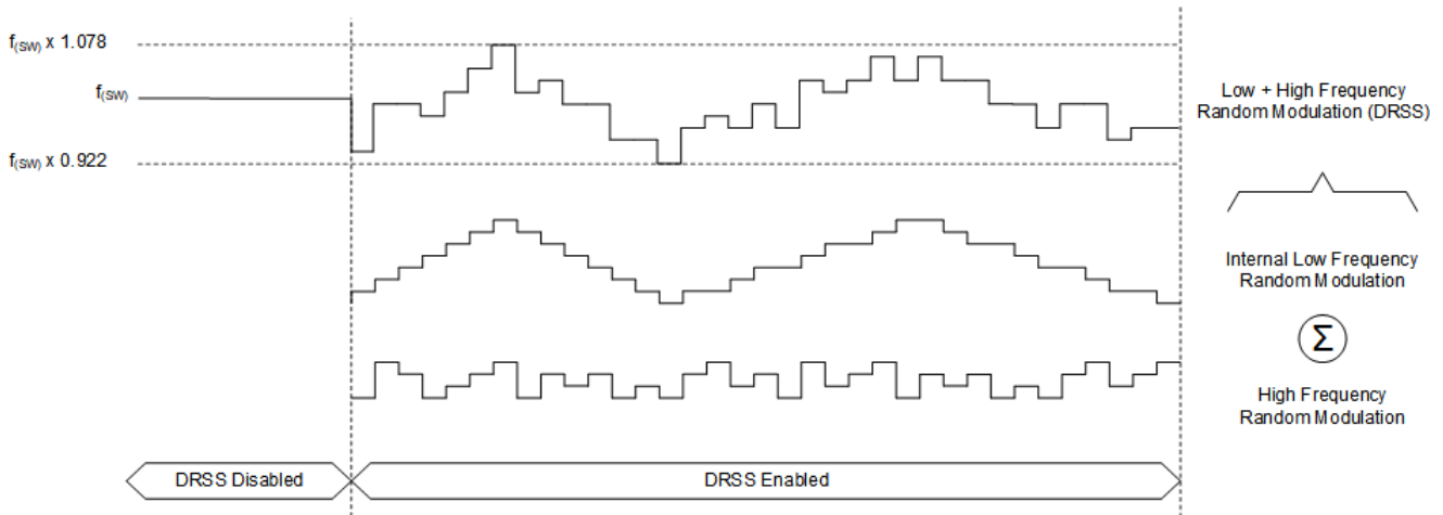
图 6-7. 双随机展频
