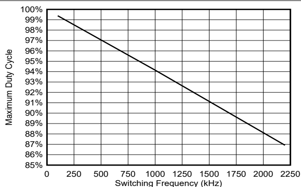
图 5-8. 最大占空比与开关频率间的关系
