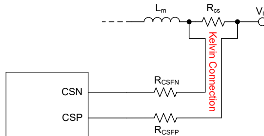
图 7-7. 电流检测滤波器
