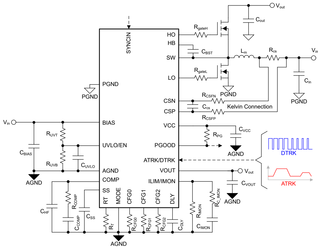
图 7-5. 典型应用
