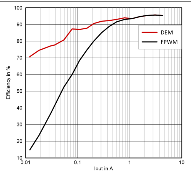
图 7-11. 效率与输出电流间的关系, V_{in} = 14.4V , V_{out} = 45V
