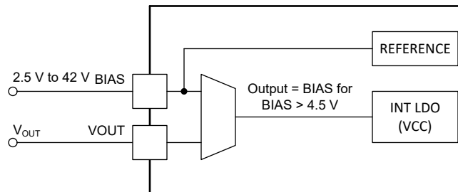
图 6-10. 动态 BIAS 电源选择
