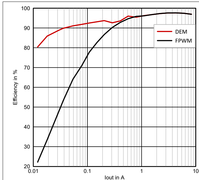
图 7-10. 效率与输出电流间的关系, V_{in} = 14.4V , V_{out} = 24V
