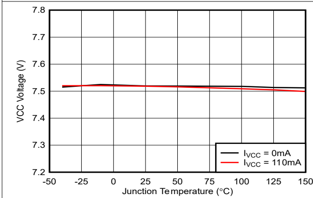
图 5-9. VCC 稳压电压与温度间的关系
