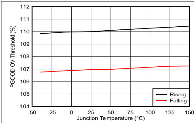
图 5-7. PG OV 阈值与温度间的关系
