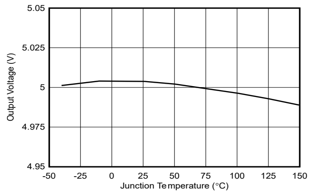
图 5-4. 固定 5V 输出电压与温度间的关系
