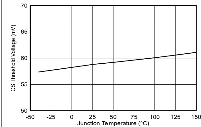
图 5-11. 电流检测 (CS) 阈值与温度间的关系
