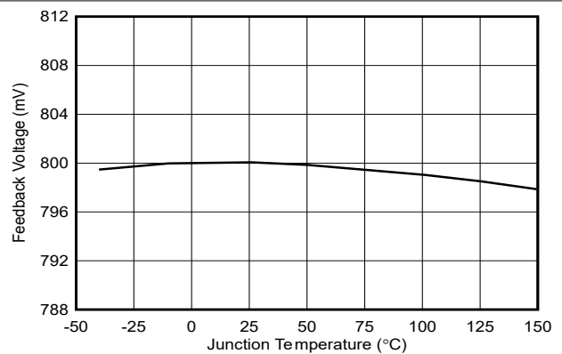
图 5-6. 反馈电压与温度之间的关系
