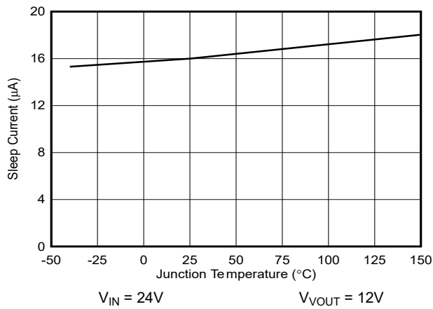
图 5-3. Sleep2 电流与温度间的关系
