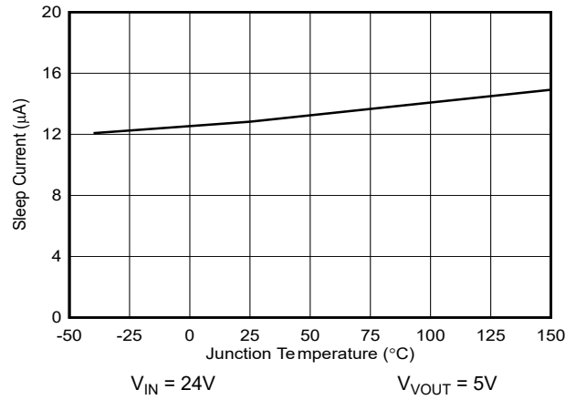
图 5-2. Sleep1 电流与温度间的关系
