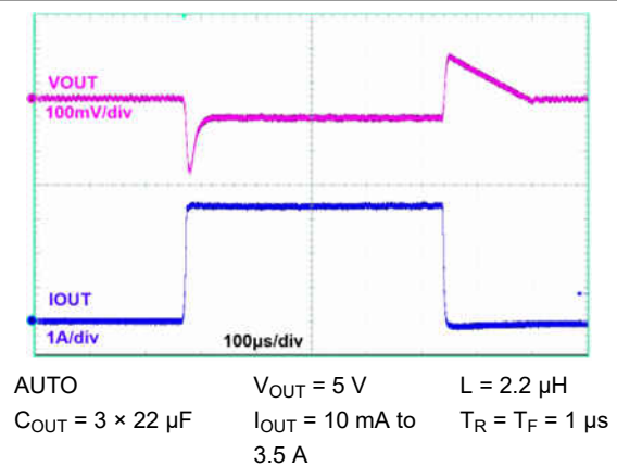
图 9-16. Load Transients
