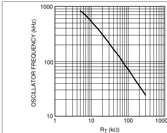
图 7-8. 振荡器频率与 R_T 间的关系
