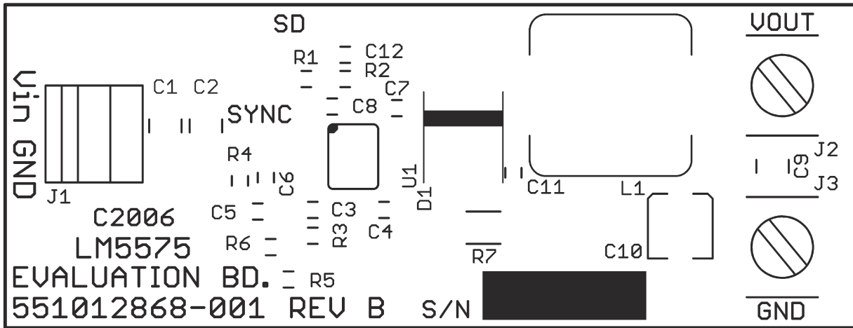
图 7-10. 丝印
