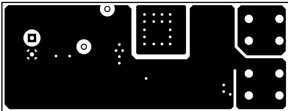
图 7-12. 焊接侧
