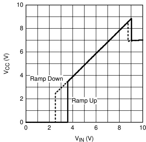
图 5-5. V_{CC} 与 V_{IN} 间的关系 R_L = 7k\Omega
