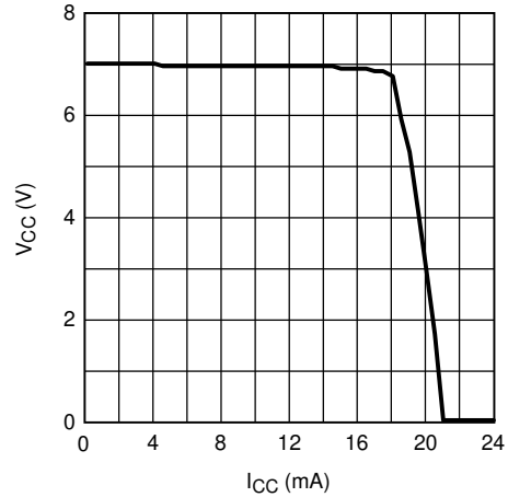
图 5-4. V_{CC} 与 I_{CC} 间的关系 V_{IN} = 12V
