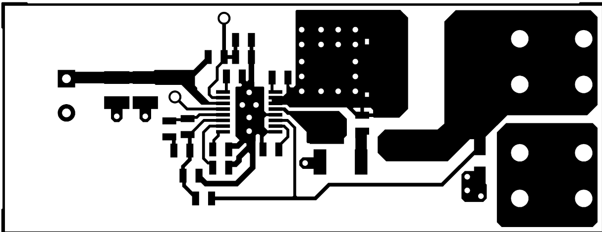
图 7-11. 组件侧
