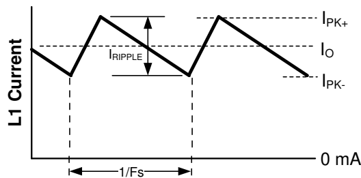
图 7-4. 电感器电流波形
