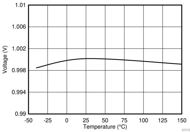
图 7-3. Feedback Voltage
