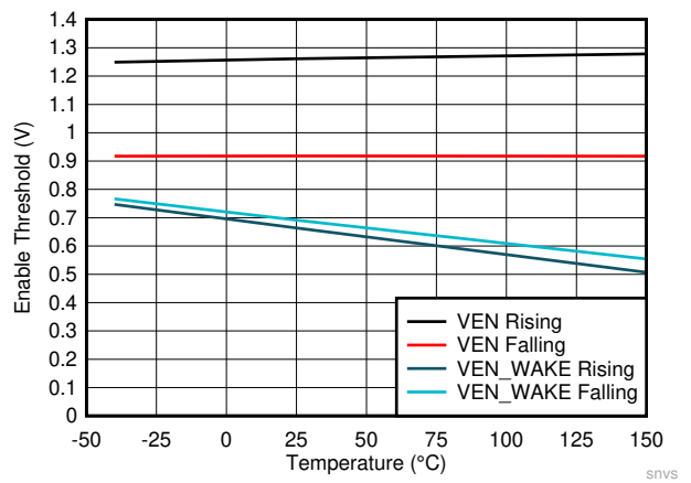
图 7-6. Enable Thresholds
