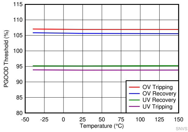
图 7-7. PGOOD Thresholds
