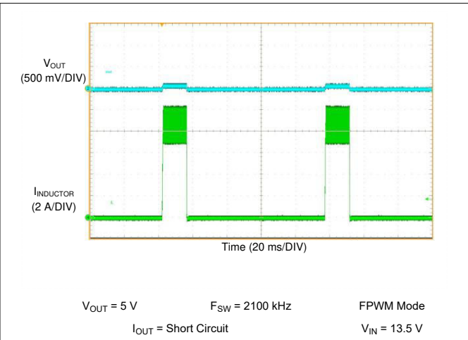
图 10-36. LM61460-Q1 Short Circuit Performance
