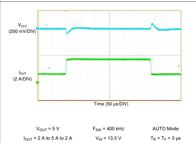
图 10-40. LM61460-Q1 Load Transient
