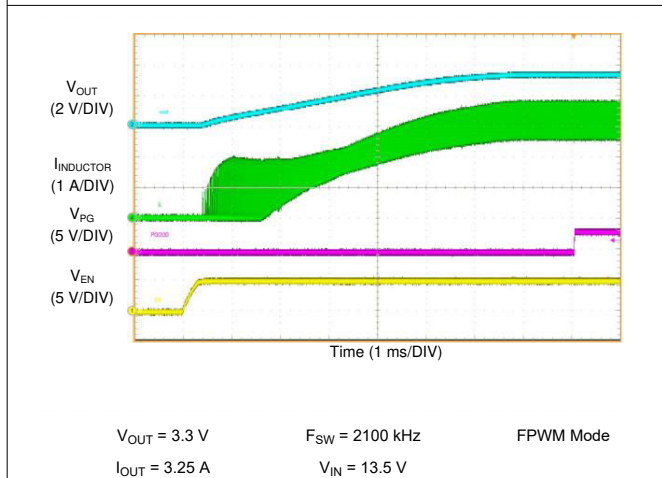
图 10-33. LM61460-Q1 Start-up with 3.25-A
