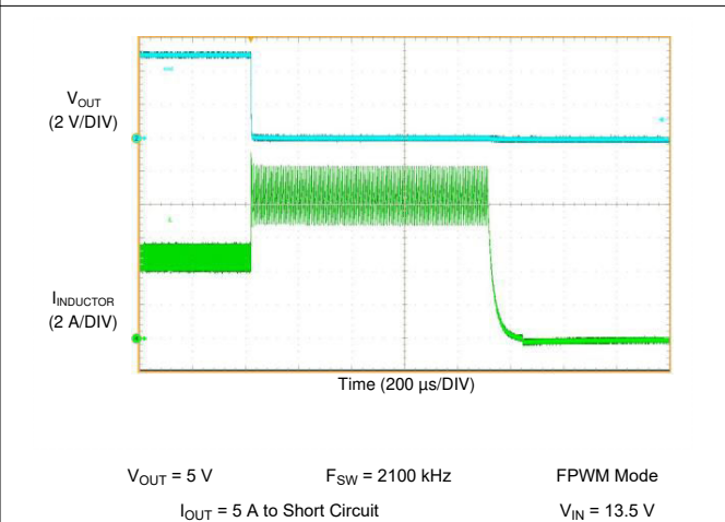
图 10-34. LM61460-Q1 Short Circuit Protection
