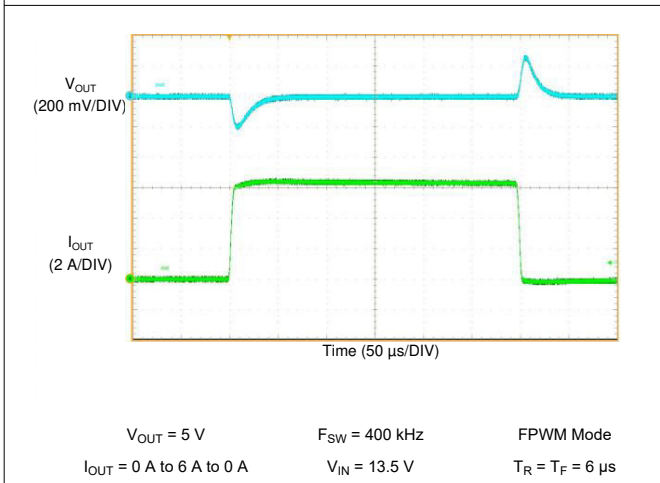
图 10-39. LM61460-Q1 Load Transient
