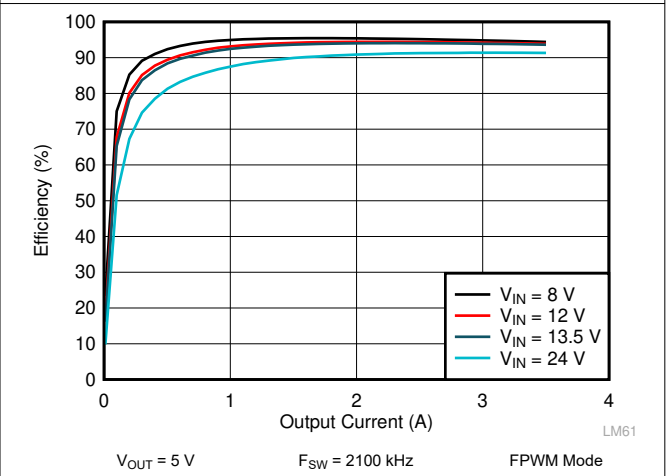
图 9-8. LM62435-Q1 Efficiency
