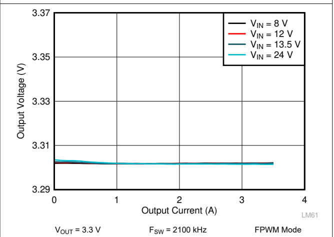
图 9-10. LM62435-Q1 Load and Line Regulation
