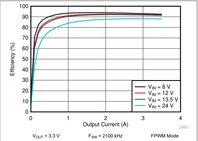
图 9-6. LM62435-Q1 Efficiency
