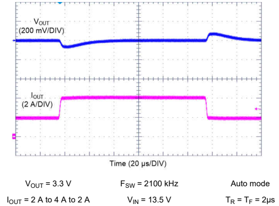
图 10-24. LM62440-Q1 Load Transient
