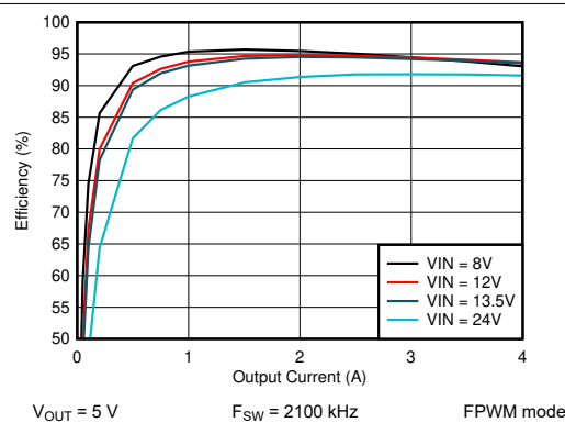
图 10-8. LM62440-Q1 Efficiency
