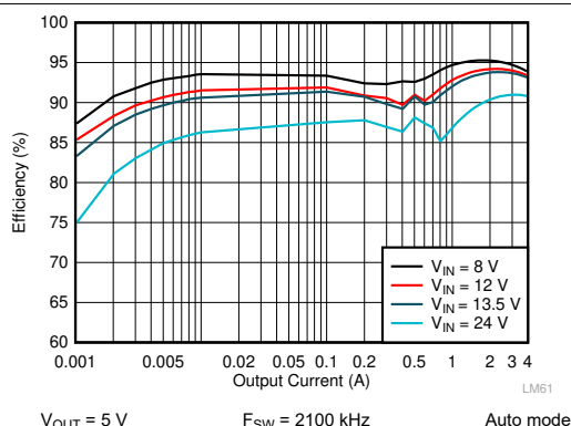
图 10-7. LM62440-Q1 Efficiency
