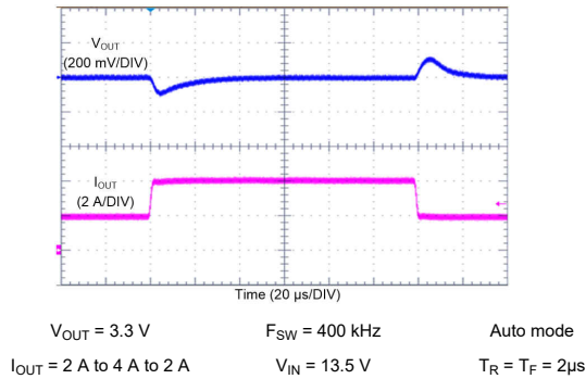
图 10-23. LM62440-Q1 Load Transient
