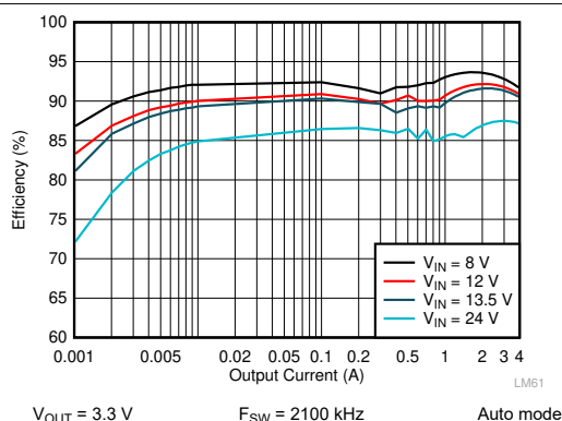
图 10-5. LM62440-Q1 Efficiency
