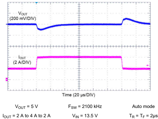
图 10-25. LM62440-Q1 Load Transient
