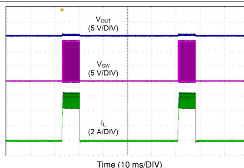
图 10-20. LM62440-Q1 Short Circuit Protection
