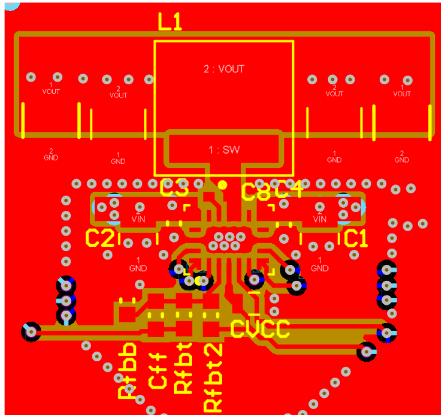
图 8-6. 布局示例
