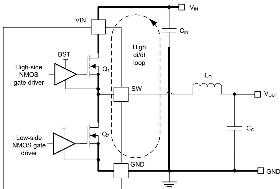
图 8-5. 具有快速边沿的电流环路
