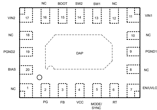
图 5-1. 20 引脚 RZT、WQFN-FCRLF 封装 (顶视图)
