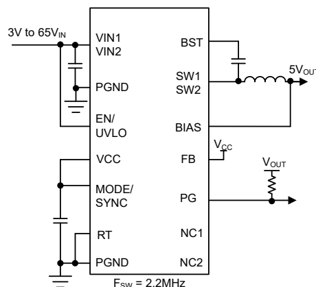
简化原理图
