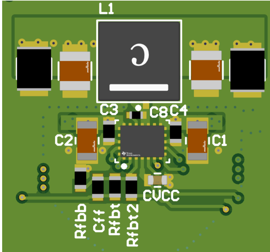
图 8-7. PCB 图像
