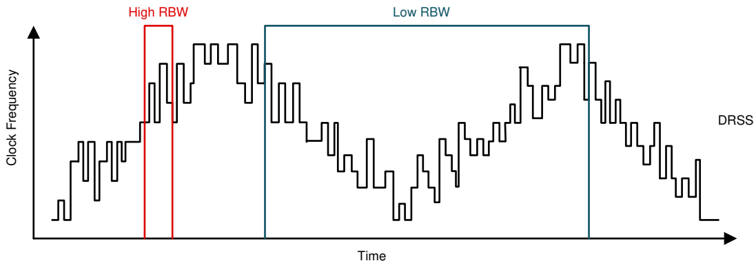
图 6-3. 双随机展频实现
