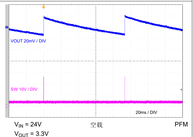
图 7-29. PFM 开关
