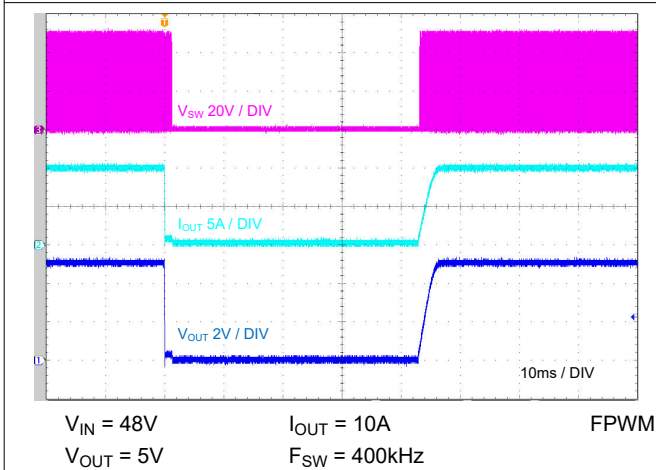
图 5-11. 短路恢复
