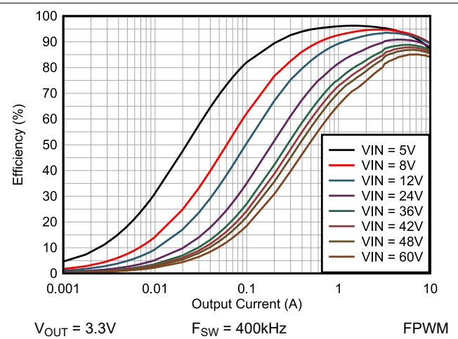
图 5-2. 效率与 I_{OUT} 之间的关系，对数标度
