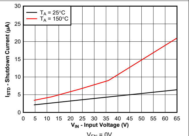
图 5-12. 关断电流与输入电压间的关系
