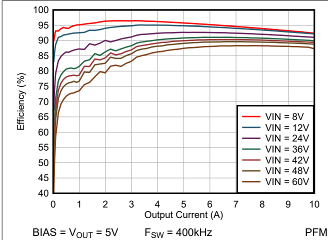
图 5-7. 效率与 I_{OUT} 之间的关系, 线性标度
