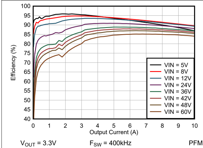
图 7-26. 效率与 I OUT 间的关系，线性标度
