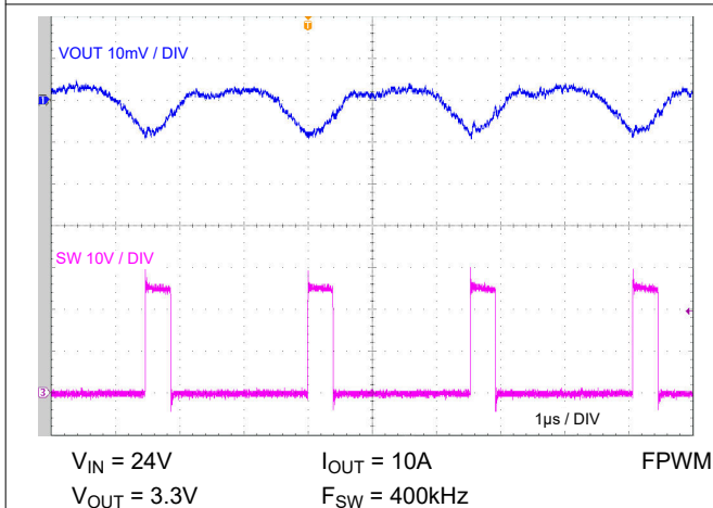
图 7-28. 满负载开关
