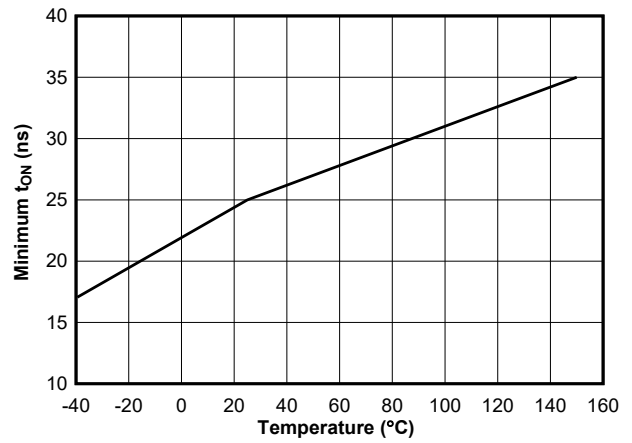
图 5-14. 最短导通时间与温度间的关系
