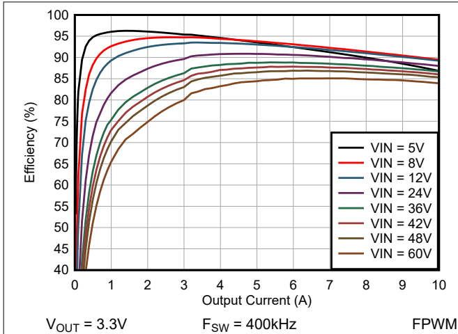
图 7-24. 效率与 I OUT 间的关系，线性标度
