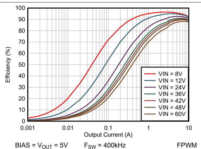
图 5-6. 效率与 I_{OUT} 之间的关系，对数标度
