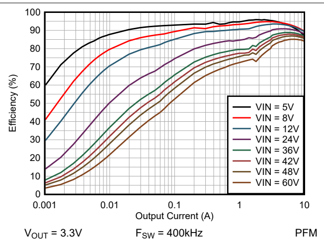
图 5-4. 效率与 I_{OUT} 之间的关系，对数标度
