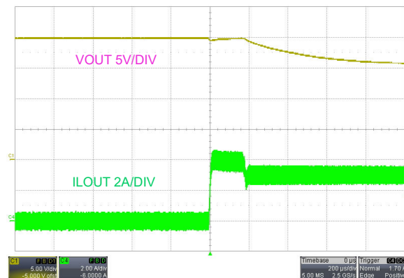
图 9-14. CV 至 CC 模式转换
