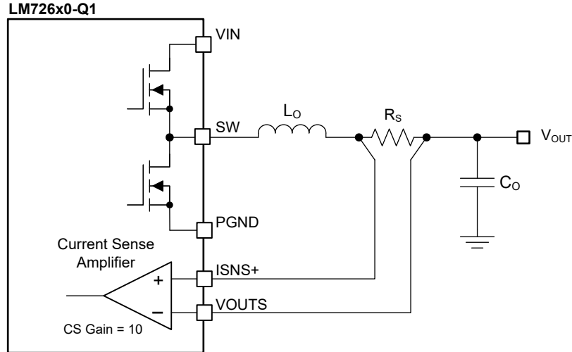
图 7-7. 分流电流检测实现
