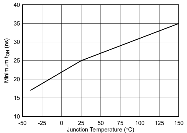
图 6-14. 最短导通时间与温度间的关系
