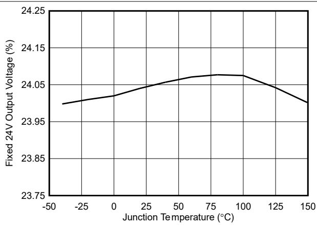
图 6-10. 固定输出电压与温度间的关系, V_{\text{OUT}} = 24\text{V}
