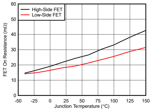
图 6-13. FET 导通电阻与温度间的关系
