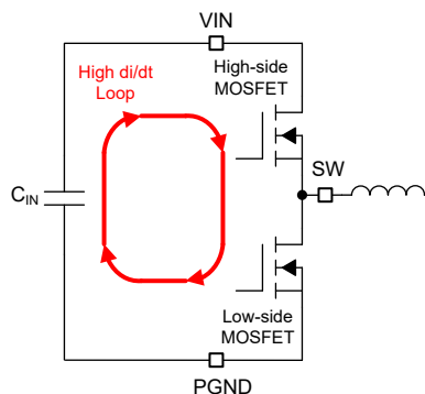
图 9-17. 输入电流环路
