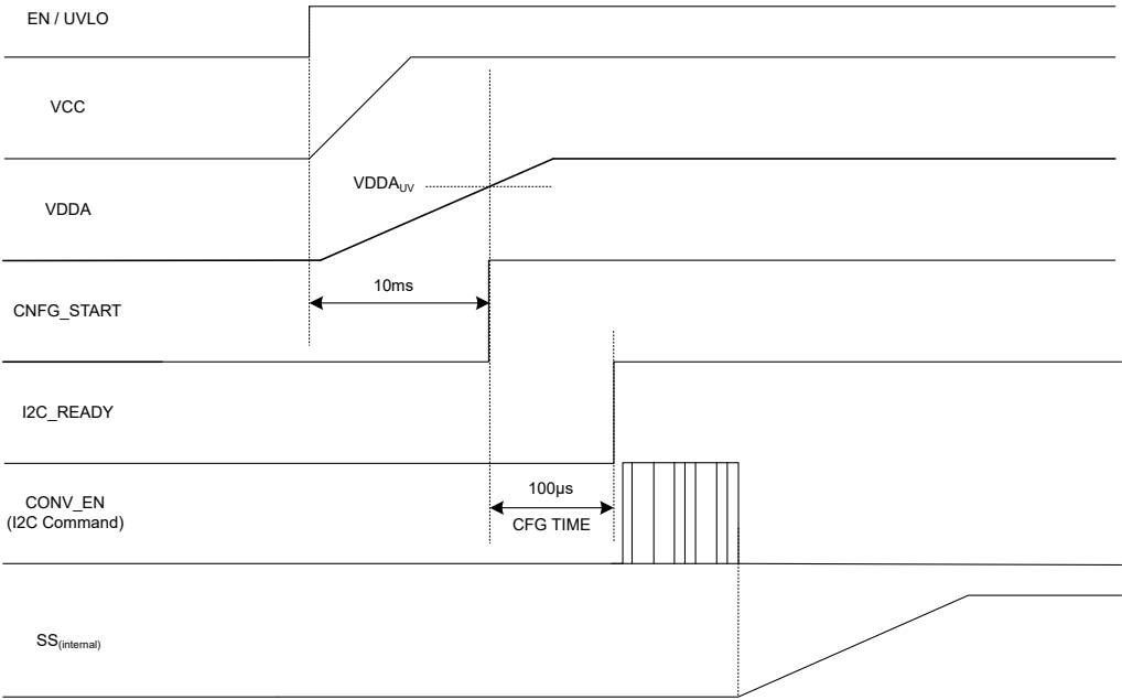
图 7-8. 配置时序
