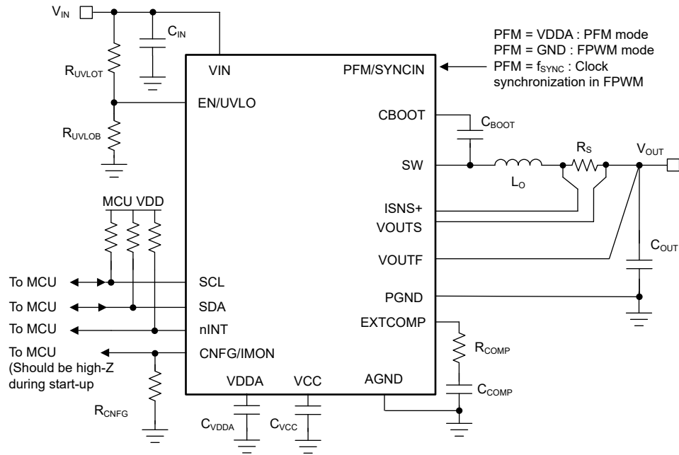
图 9-6. 具有 I2C 接口的应用电路
