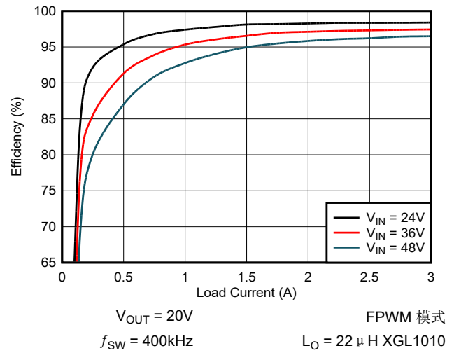
图 6-2. 效率 ( V_{OUT} = 20\text{V} )
