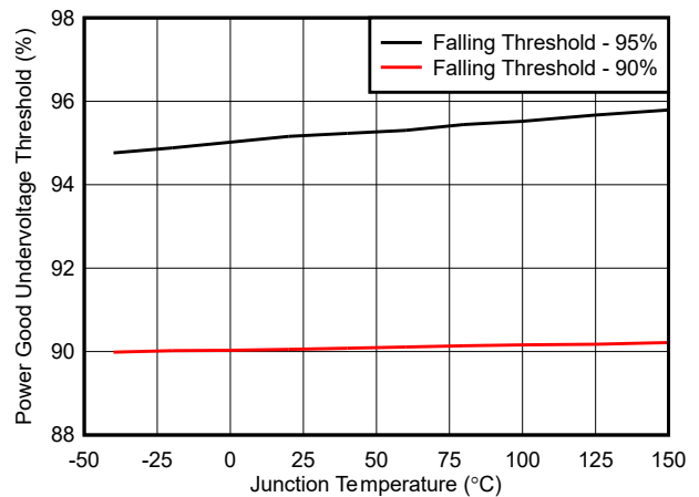
图 6-12. PG 欠压阈值与温度间的关系
