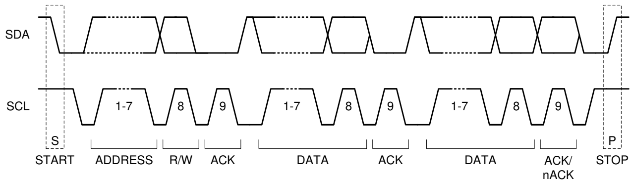
图 7-9. I 2 C 启动/停止/确认协议
