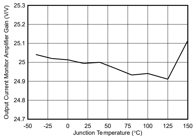
图 6-15. IMON 放大器增益与温度间的关系
