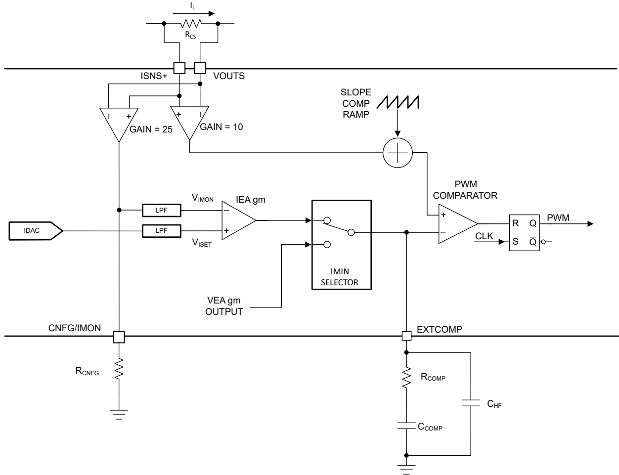
图 7-6. 电流环路功能方框图
