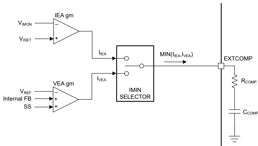
图 7-4. 双环路架构方框图
