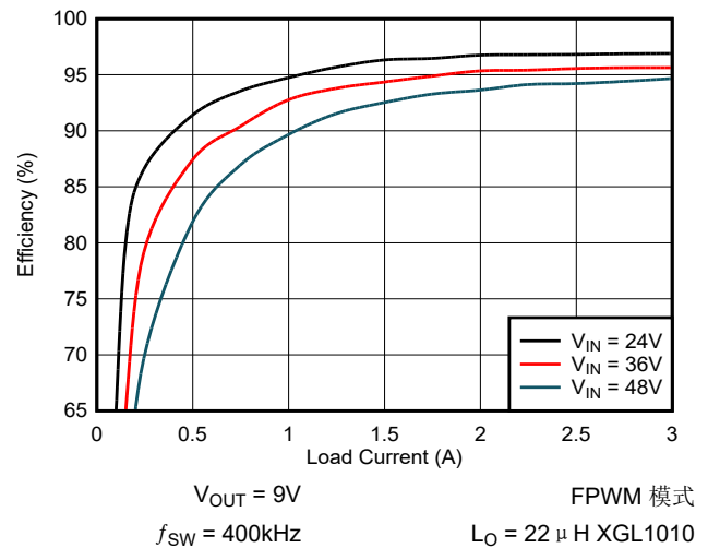
图 6-4. 效率 ( V_{OUT} = 9\text{V} )
