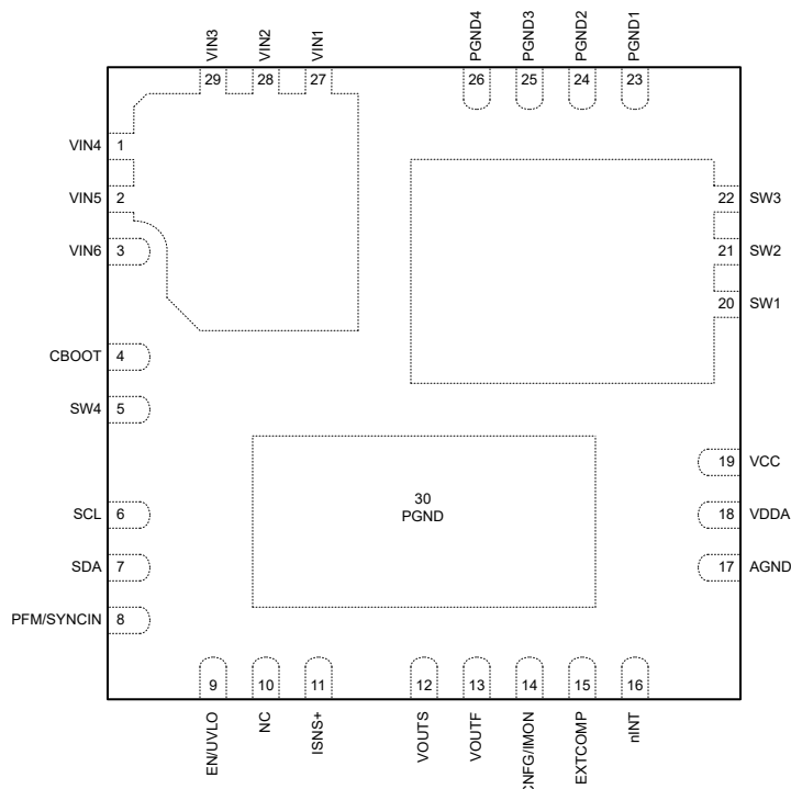
图 5-1. RRX 29 引脚 VQFN (顶视图)
