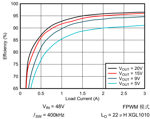
图 6-1. 效率 ( V_{IN} = 48\text{V} )
