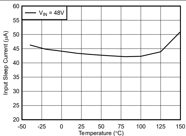
图 6-6. 输入睡眠电流与温度间的关系, V_{\text{OUT}} = 5\text{V}
