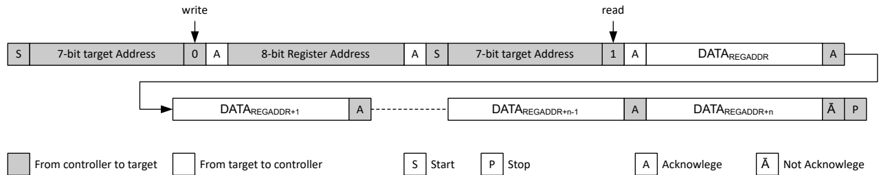
图 7-13. 从定义的寄存器地址开始进行顺序读取
