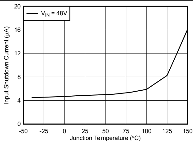
图 6-5. 输入关断电流与温度间的关系
