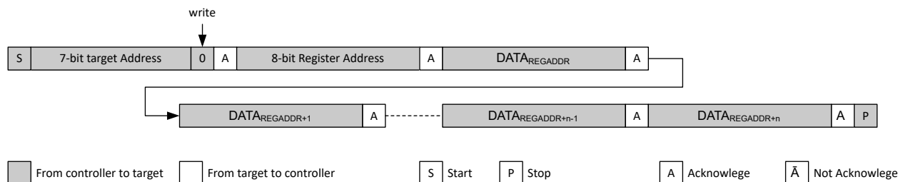
图 7-15. 在定义的寄存器地址开始进行顺序写入
