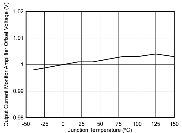
图 6-16. IMON 放大器电压偏移与温度间的关系
