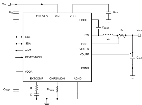
典型应用电路
