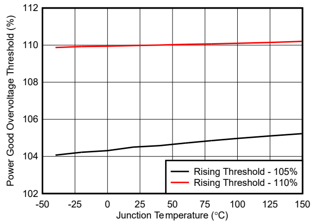
图 6-11. PG 过压阈值与温度间的关系
