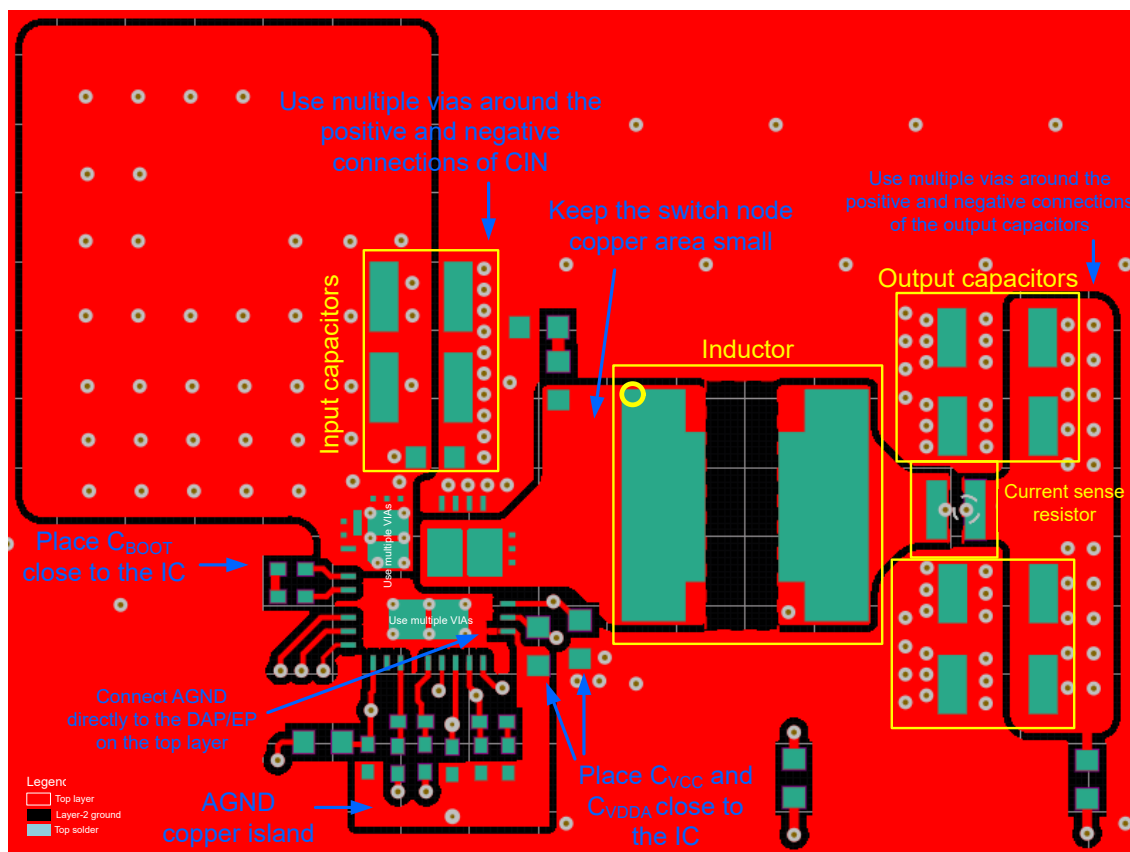
图 9-18. PCB 顶层
