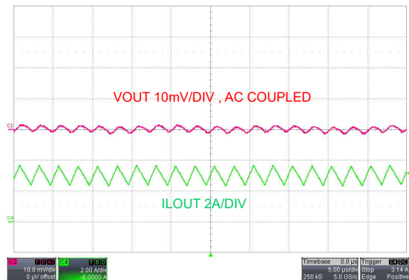
20V 输出, 3A 负载
