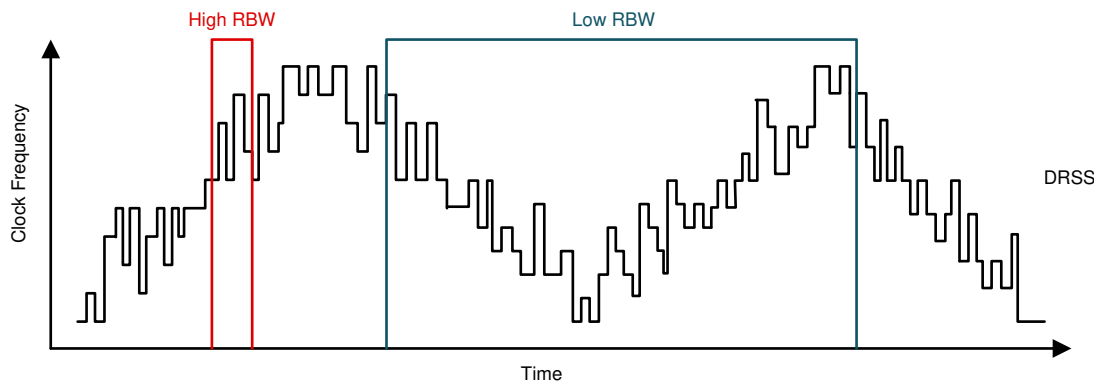
图 7-3. 双随机展频实现
