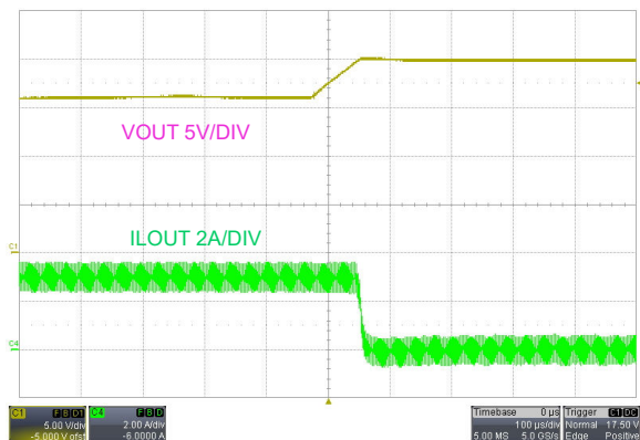
图 9-13. CC 至 CV 模式转换
