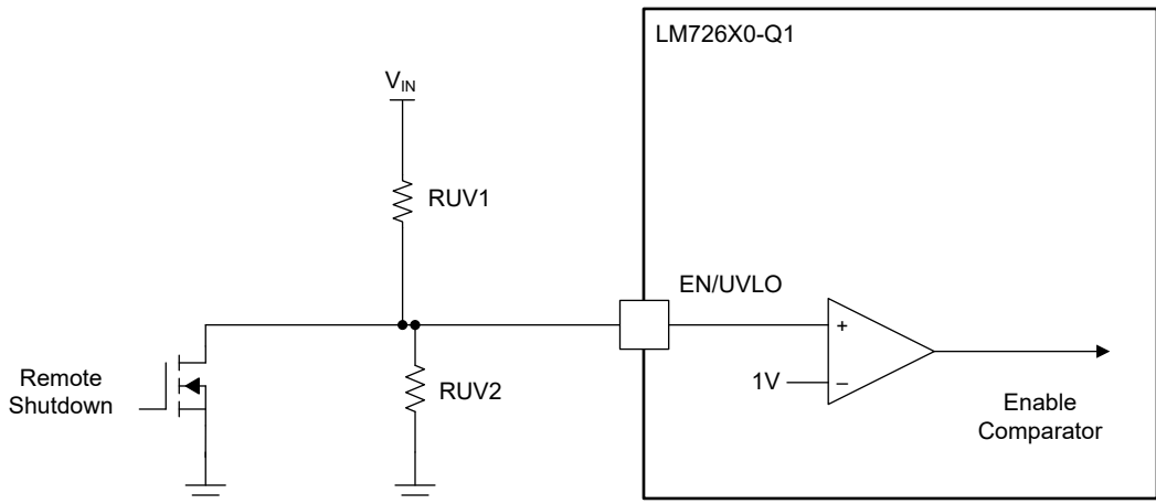
图 7-2. 可编程输入电压 UVLO 导通和关断
