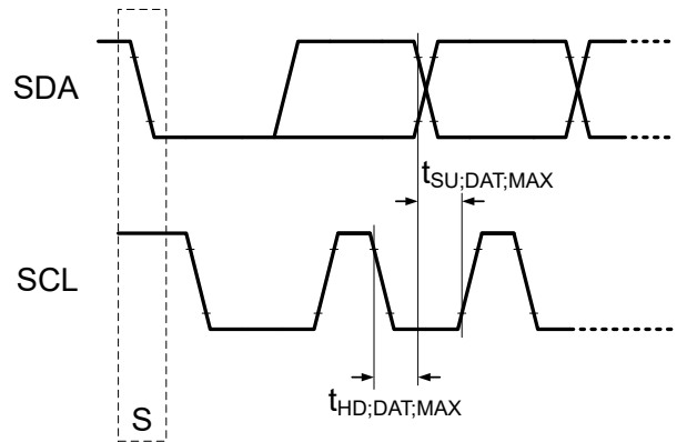
图 7-11. 最长上升和下降时间的 I 2 C 数据传输时序
