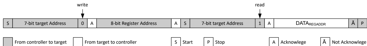
图 7-12. 从定义的寄存器地址进行单次读取
