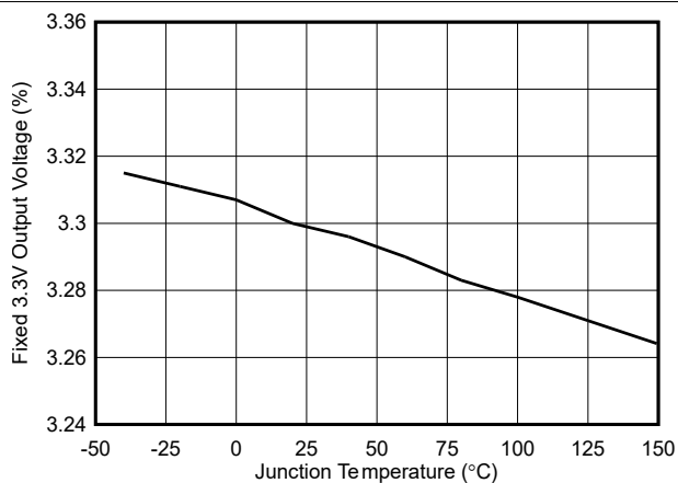
图 6-8. 固定输出电压与温度间的关系, V_{\text{OUT}} = 3.3\text{V}
