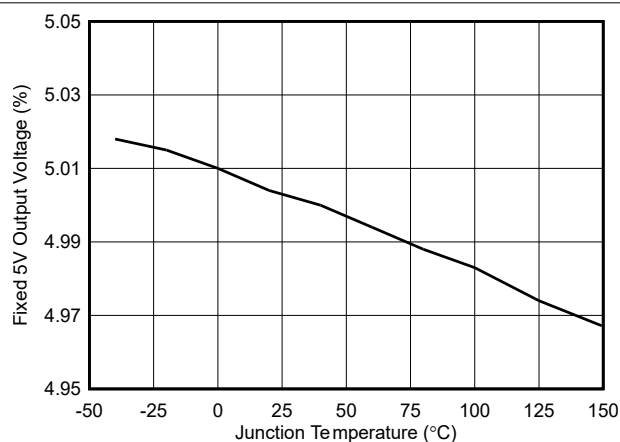
图 6-9. 固定输出电压与温度间的关系, V_{\text{OUT}} = 5\text{V}
