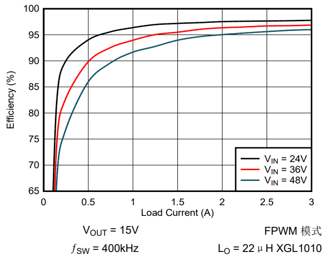
图 6-3. 效率 ( V_{OUT} = 15\text{V} )
