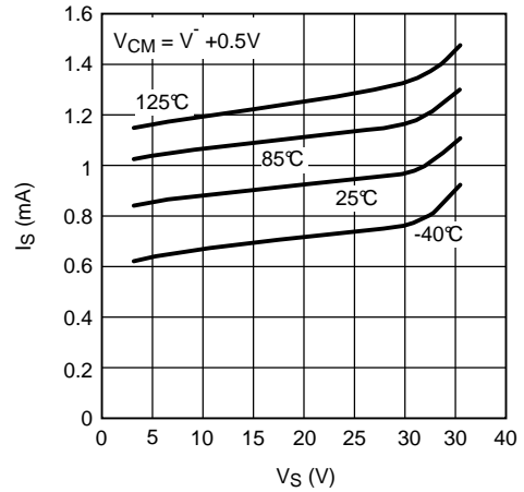
图 34. I_S 与 V_S 间的关系 (LM7321)
