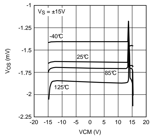
图 14. V_{OS} 与 V_{CM} 间的关系 (单位 1)
