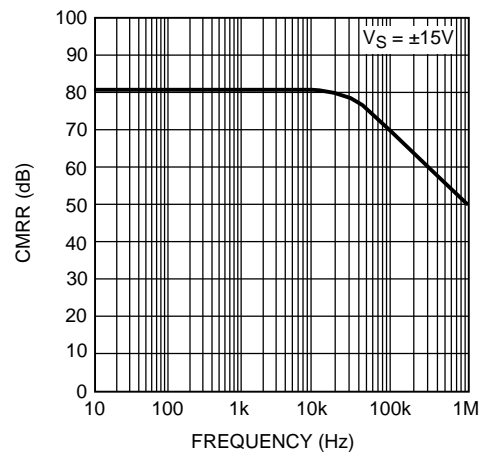
图 46. CMRR 与频率间的关系
