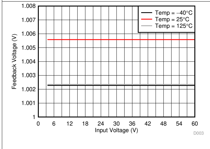
图 3. Feedback Voltage
