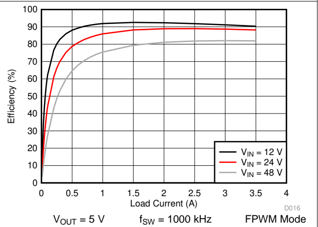
图 28. LM76003 Efficiency
