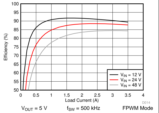
图 26. LM76003 Efficiency
