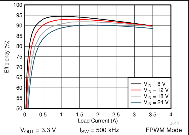
图 24. LM76003 Efficiency
