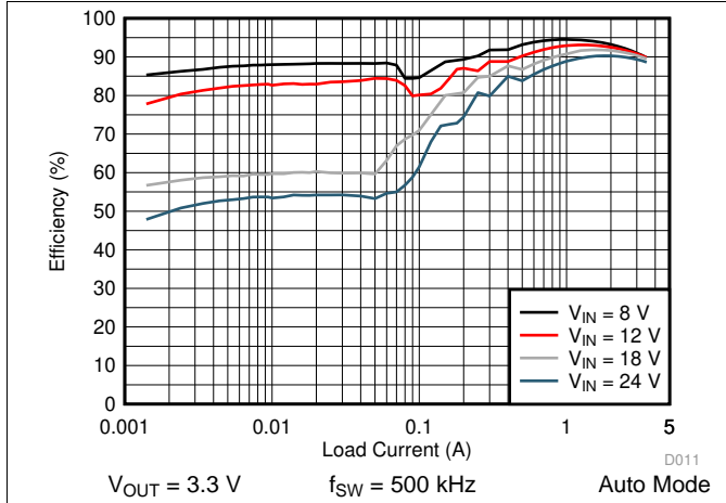
图 23. LM76003 Efficiency
