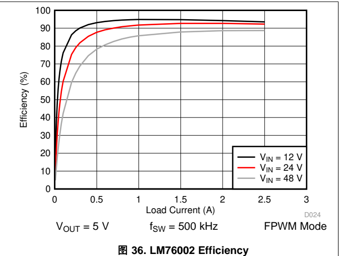
图 36. LM76002 Efficiency
