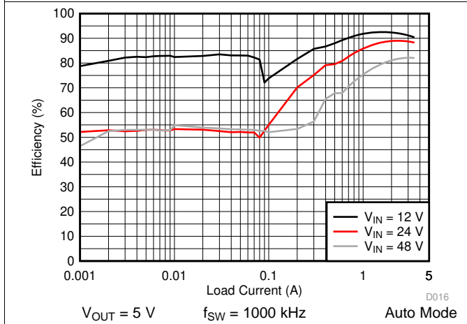
图 27. LM76003 Efficiency
