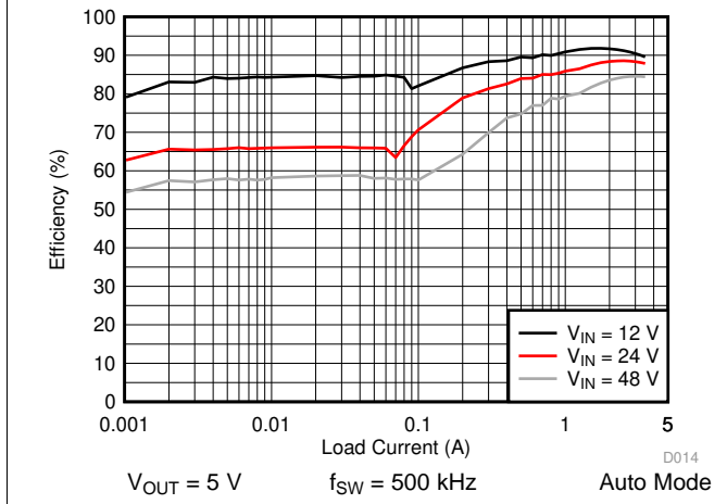
图 25. LM76003 Efficiency
