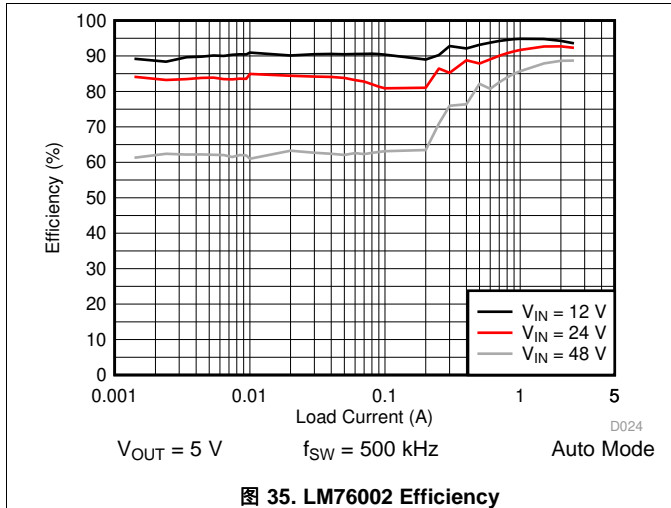
图 35. LM76002 Efficiency
