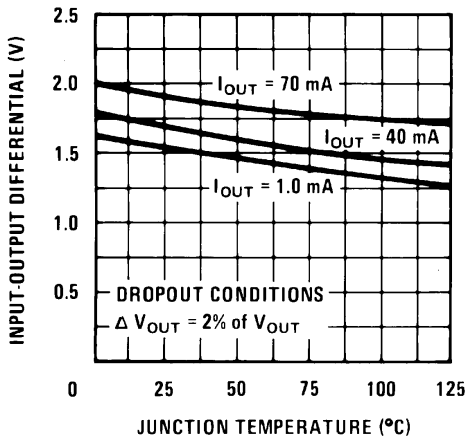
图 5-3. 压降电压
