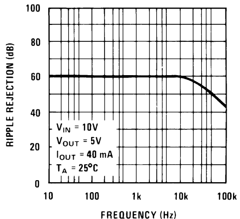
图 5-4. 纹波抑制
