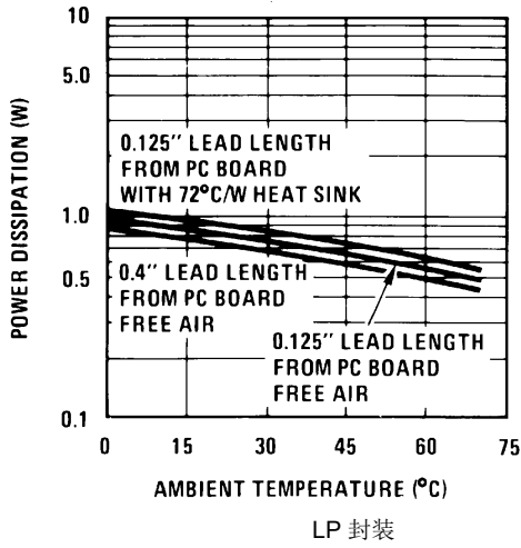
图 5-1. 最大平均功率耗散
