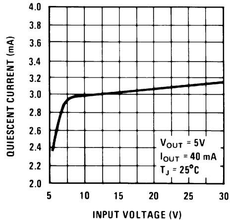
图 5-6. 静态电流
