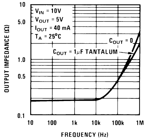
图 5-5. 输出阻抗
