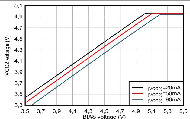
图 6-12. VCC2 LDO 输出电压与 BIAS 电压间的关系 V_{(VIN)} = 2.5\text{V}
