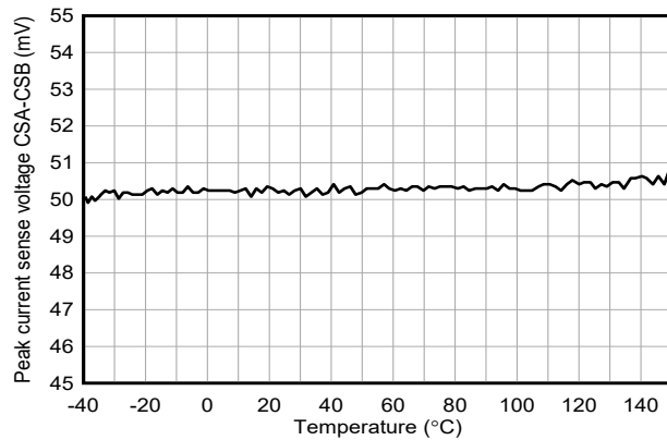
图 6-23. 峰值电流限制阈值电压与温度间的关系
