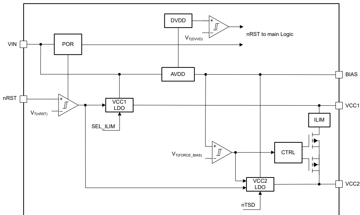
图 8-9. 参考系统功能方框图
