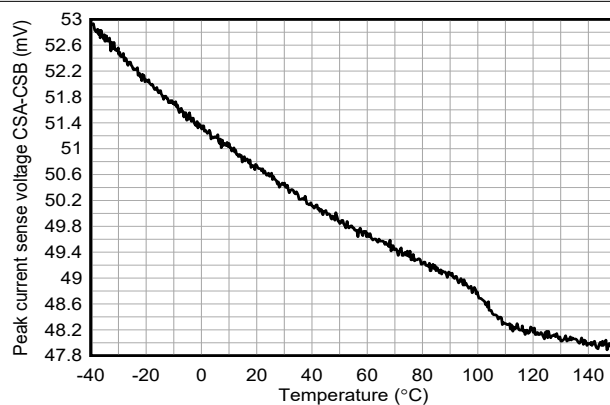
图 6-26. 平均电流限制阈值电压与温度间的关系 ILIM\_THRESHOLD = 0x64
