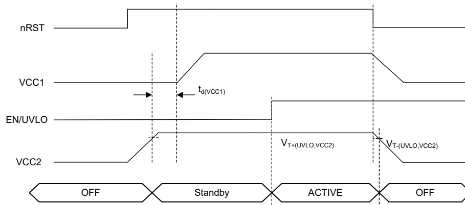
图 8-11. VCC 稳压器时序图
