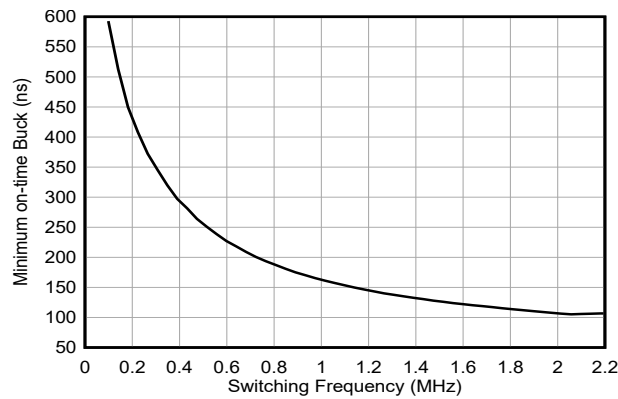
图 6-17. 降压最短导通时间与开关频率间的关系
