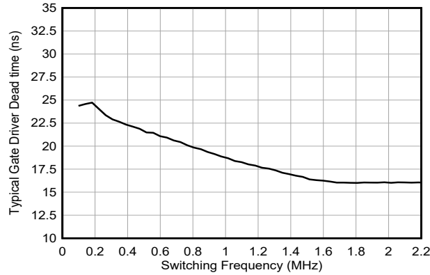
图 6-21. 栅极驱动器转换 (死区) 时间与开关频率间的关系 SEL_MIN_DEADTIME_GDRV = 0b01, SEL_SCALE_DT = 0b0, EN_CONST_TDEAD = 0b0
