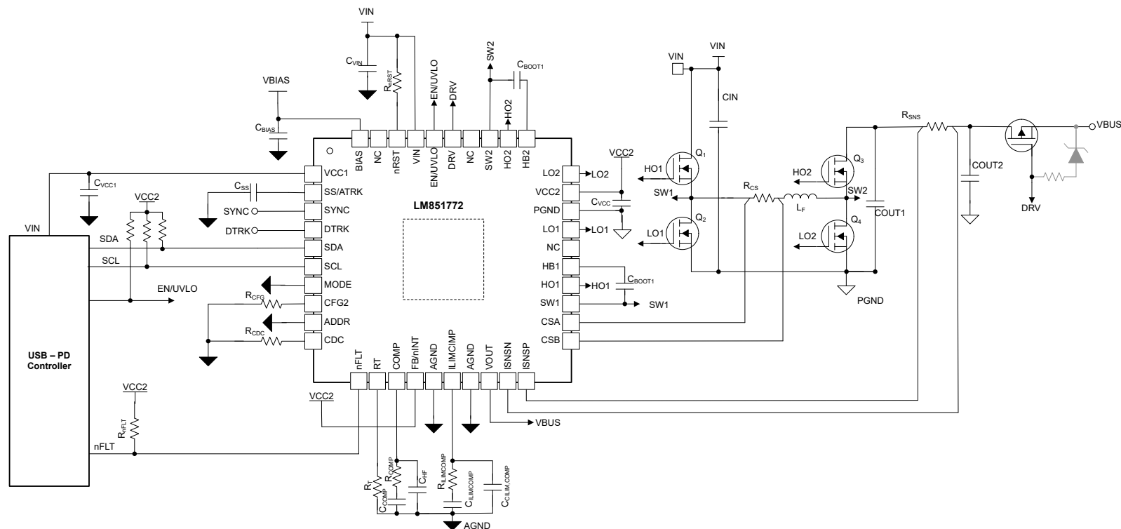
图 10-26. 具有电源路径的 USB PD 源的简化版原理图
