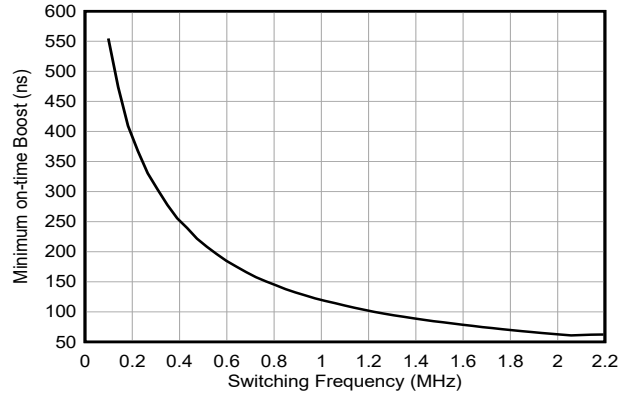
图 6-19. 升压最短导通时间与开关频率间的关系
