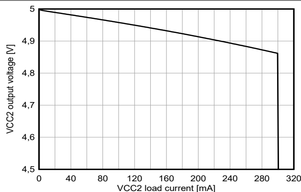
图 6-11. VCC2 LDO 输出电压与 VCC2 负载电流间的关系 V_{(VIN)} = 3.5\text{V} , V_{(BIAS)} = 12\text{V}
