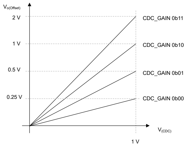
图 8-27. Vo 偏移电压与 CDC 电压的关系
