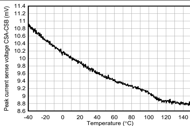
图 6-28. 平均电流限制阈值电压与温度间的关系 ILIM\_THRESHOLD = 0x14
