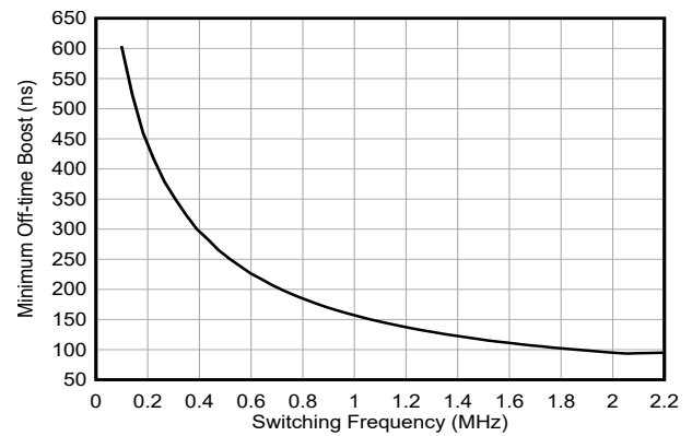
图 6-18. 升压最短关断时间与开关频率间的关系
