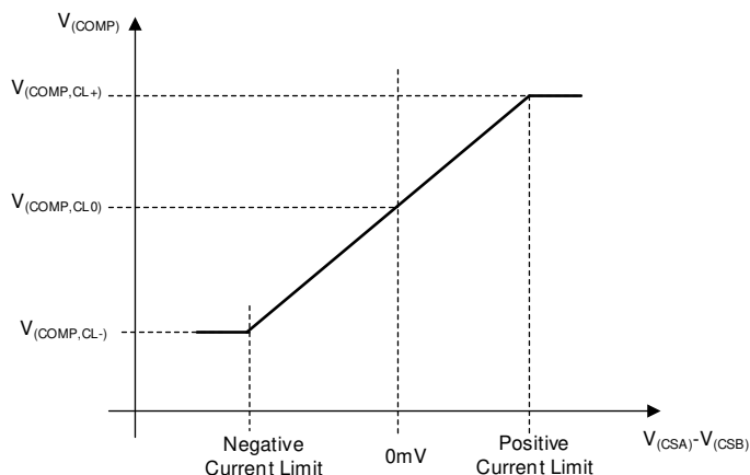
图 8-13. 峰值电流检测电压与 V_{COMP} 间关系的控制函数
