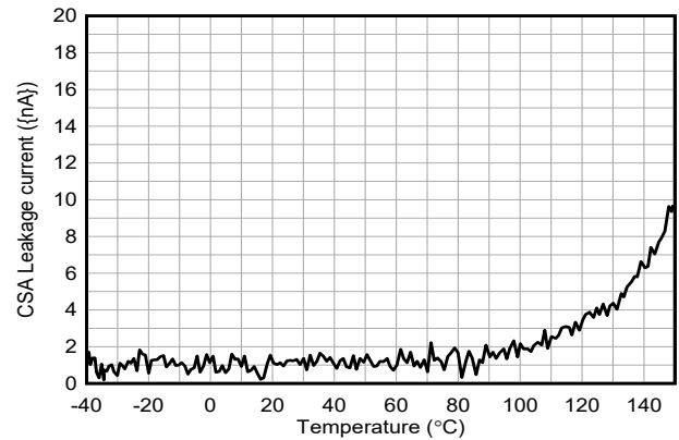
图 6-24. CSA 输入电流与温度间的关系
