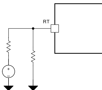
图 8-20. 动态更改频率的示例
