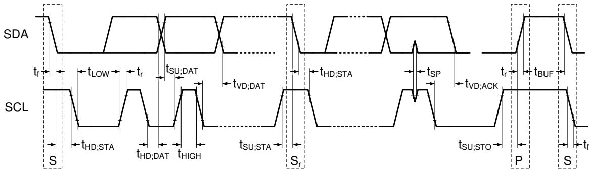
图 8-33. I 2 C 数据传输时序
