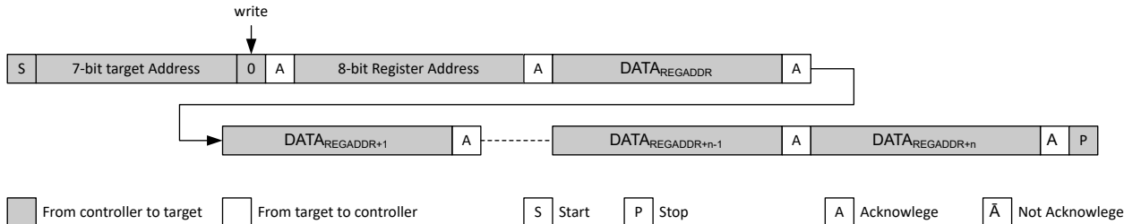
图 8-38. 在定义的寄存器地址开始进行顺序写入
