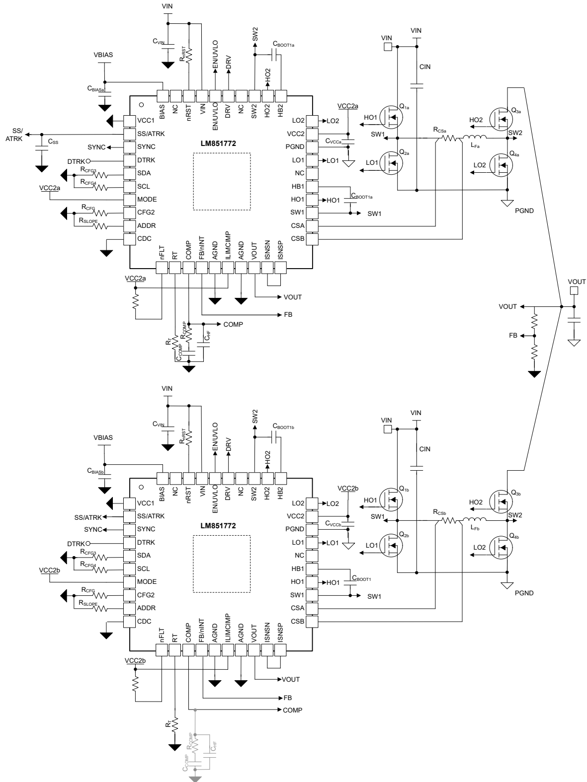
图 10-27. 两相运行的简化版原理图
