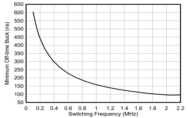
图 6-16. 降压最短关断时间与开关频率间的关系
