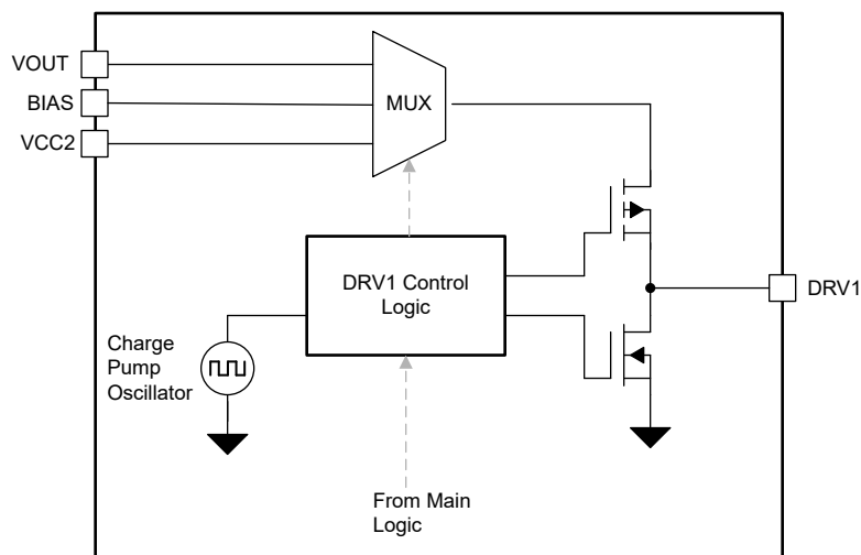
图 8-24. 功能方框图 - DRV 引脚
