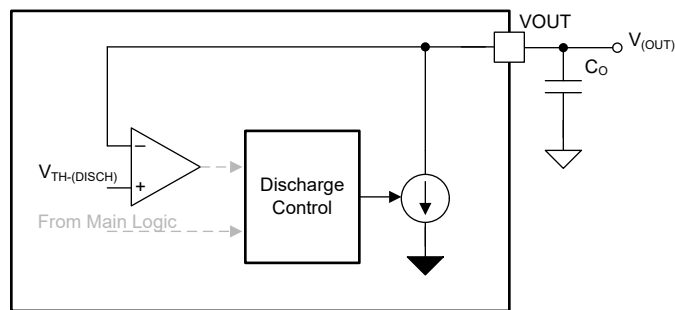
图 8-15. 功能方框图输出放电
