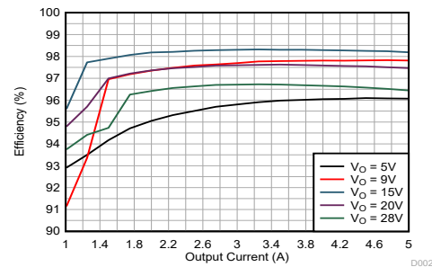
效率与输出电流间的关系，V I = 12V，PSM
