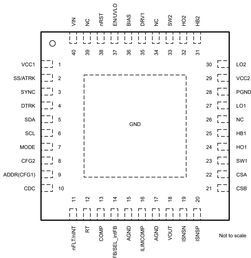
图 5-1. LM851772-Q1 RHA 封装，40 引脚 QFN (顶视图)
