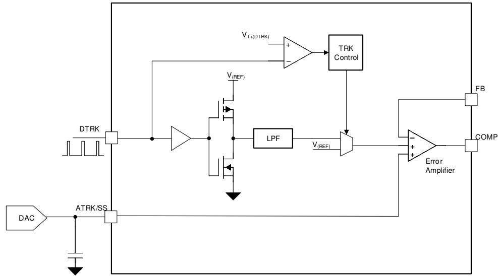
图 8-23. 输出电压跟踪功能方框图
