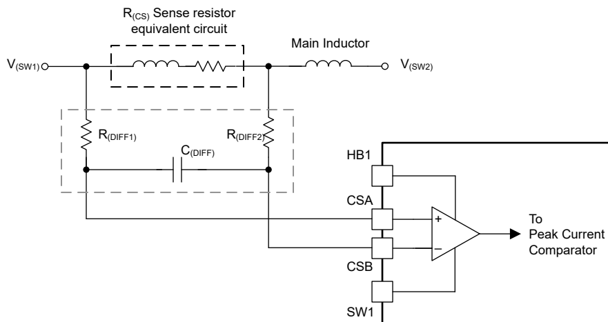
图 8-16. 峰值电流传感器的简化版原理图
