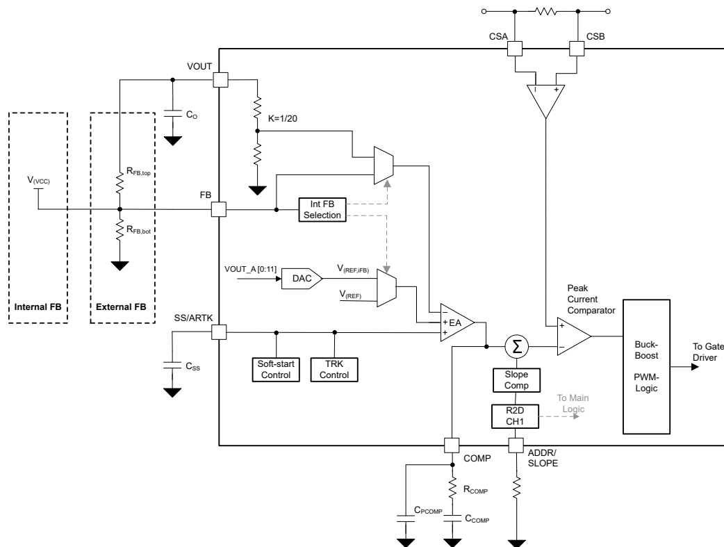
图 8-14. EA 功能方框图
