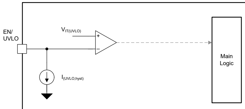
图 8-12. 功能方框图 UVLO
