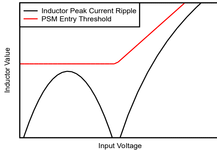
图 8-8. PSM 进入阈值与纹波电流随输入电压变化的通用曲线图
