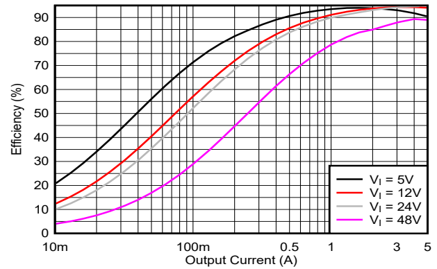
图 10-3. 效率与 I_O 间的关系 (MODE = VCC2, V_O = 12V )
