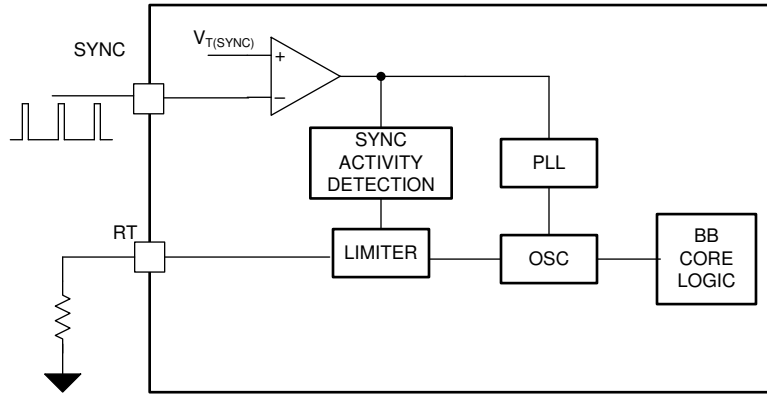
图 8-21. 主振荡器功能方框图
