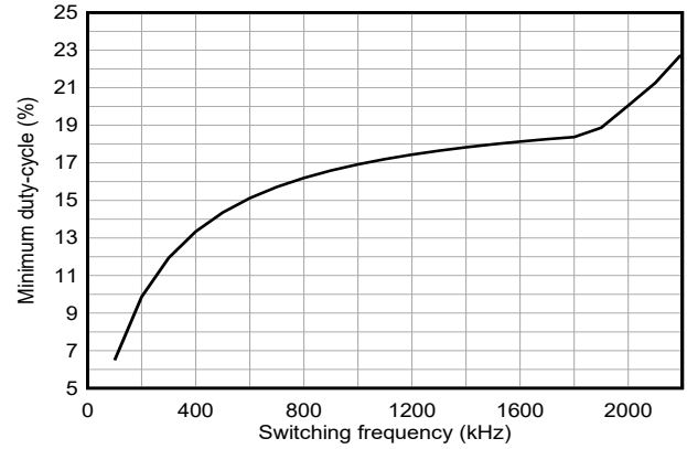
图 6-20. PSM 运行的降压最小占空比与开关频率间的关系 (SYNC_OUT = 启用)
