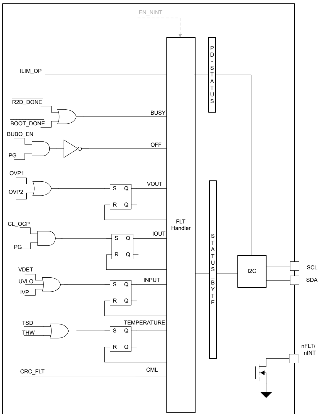
图 8-28. 功能方框图故障处理程序
