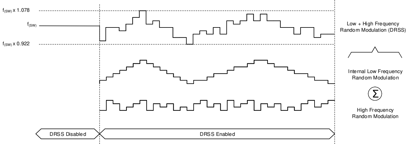
图 8-25. 双随机展频
