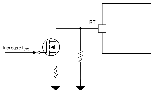
图 8-19. 跳频示例
