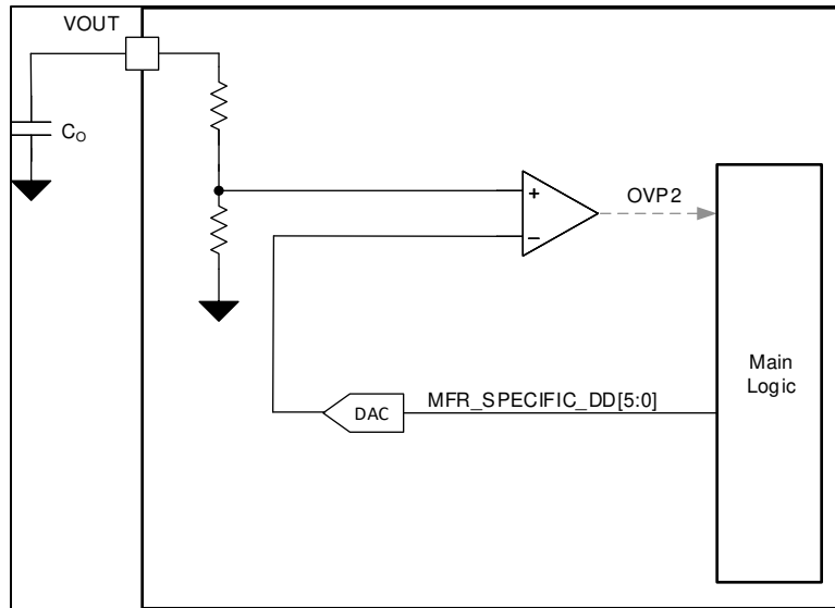
图 8-29. OVP2 功能方框图
