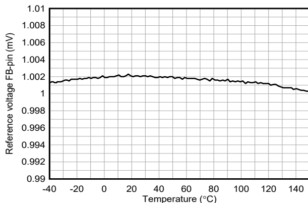
图 6-3. FB 引脚基准电压与温度间的关系
