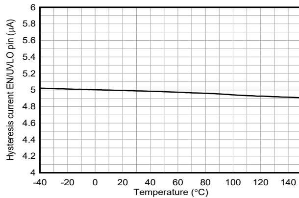
图 6-15. EN/UVLO 上的迟滞电流与温度间的关系
