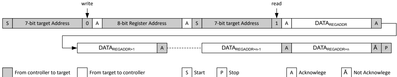
图 8-36. 从定义的寄存器地址开始进行顺序读取
