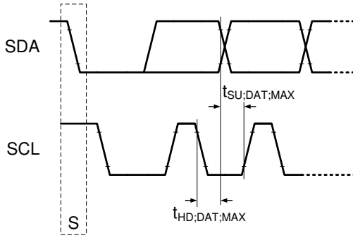
图 8-34. 最长上升/下降时间的 I 2 C 数据传输时序
