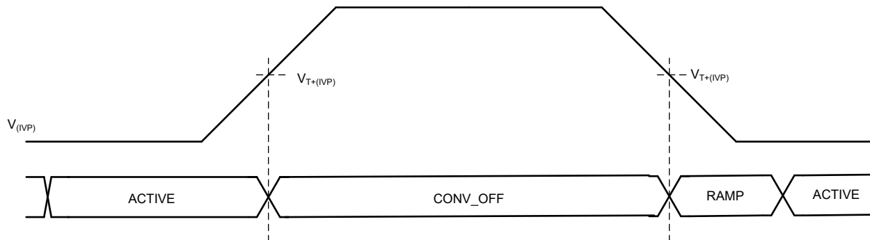
图 8-30. IVP 运行时序图
