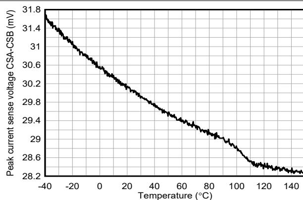
图 6-27. 平均电流限制阈值电压与温度间的关系 ILIM\_THRESHOLD = 0x3C
