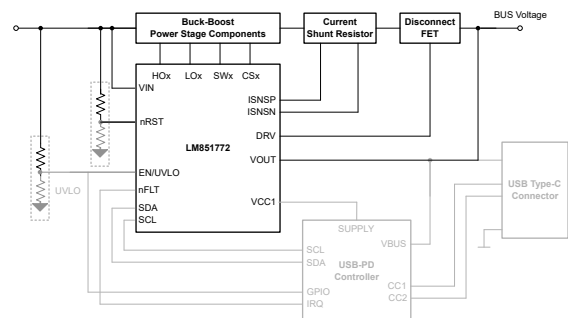
典型应用原理图
