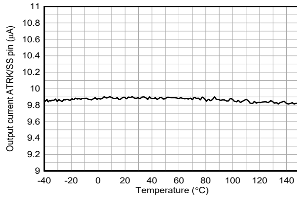
图 6-13. 软启动电流与温度间的关系
