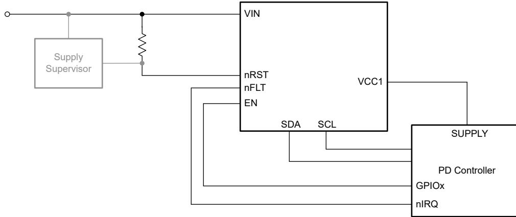
图 8-10. 简化版原理图
