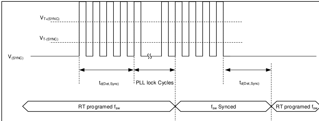
图 8-22. 时序图 SYNC 功能
