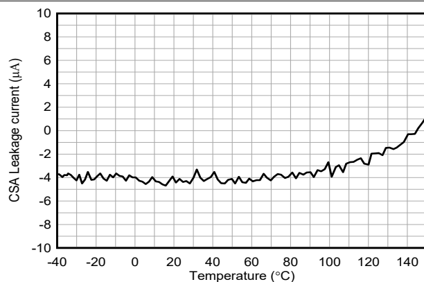
图 6-25. CSB 输入电流与温度间的关系
