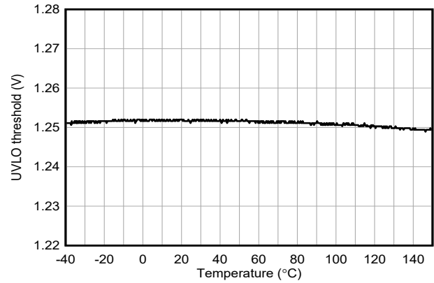
图 6-14. EN/UVLO 阈值与温度间的关系
