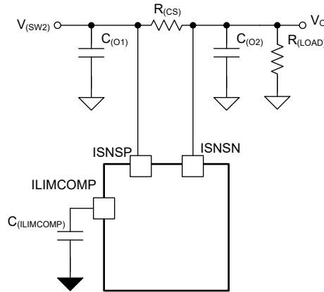
图 8-18. 具有阻性负载的电流限制元件简化版原理图
