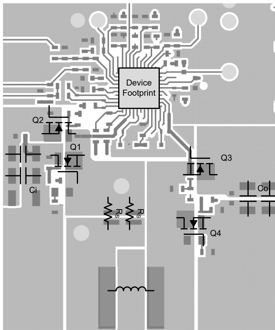
图 10-29. LM851772-Q1 简化版顶层示例
