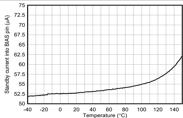
图 6-10. 流入 BIAS 的待机电流与温度间的关系 V_{(VIN)} = 3.5\text{V} , V_{(VIN)} = 12\text{V}
