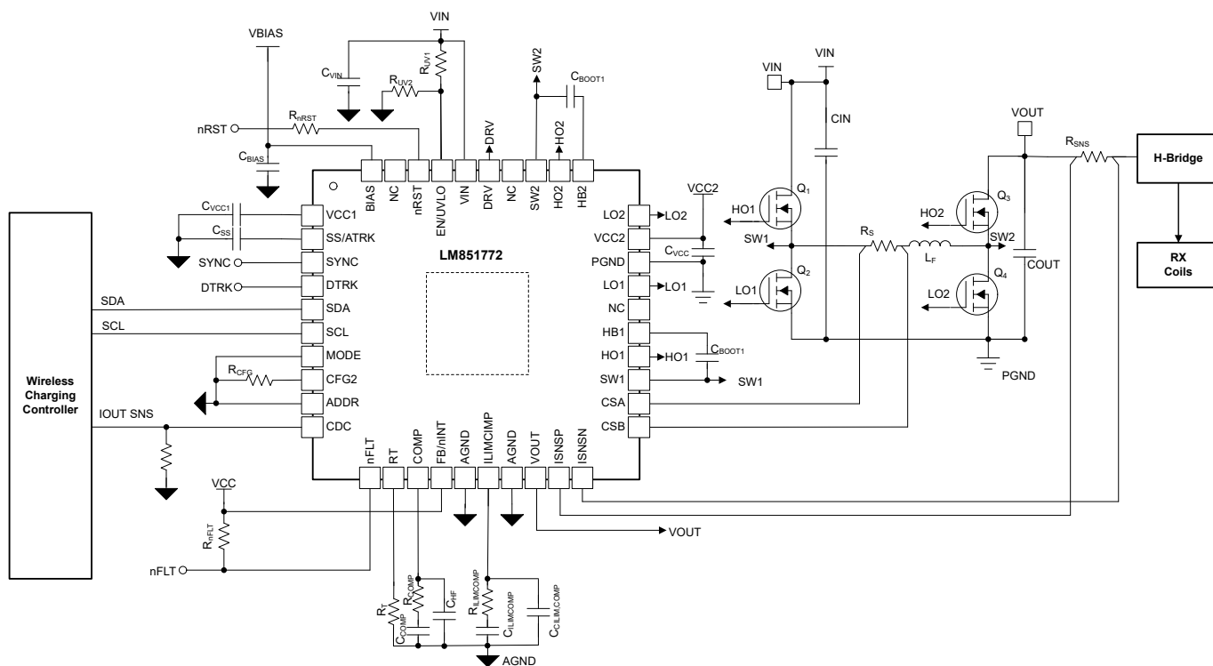
图 10-28. 无线充电电源的简化版原理图
