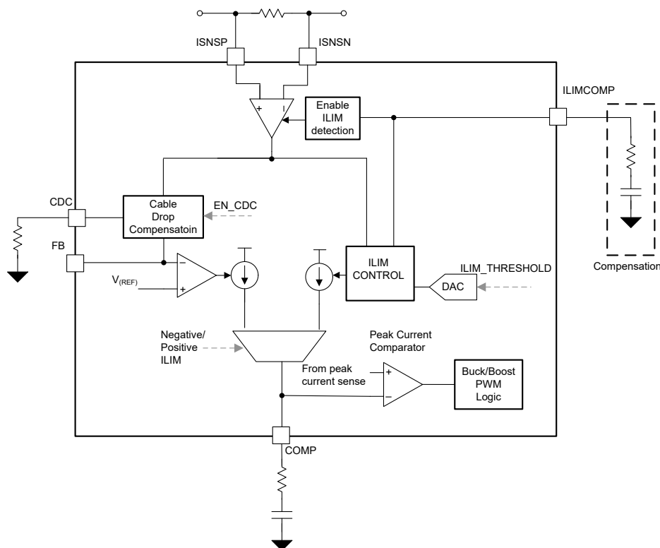
图 8-17. 电流监测功能方框图
