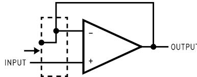
图 6-18. 跟随器
