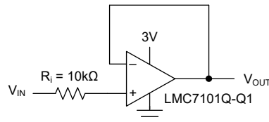
图 6-3. 在电压超过电源电压的情况下，提供 R_i 输入电流保护
