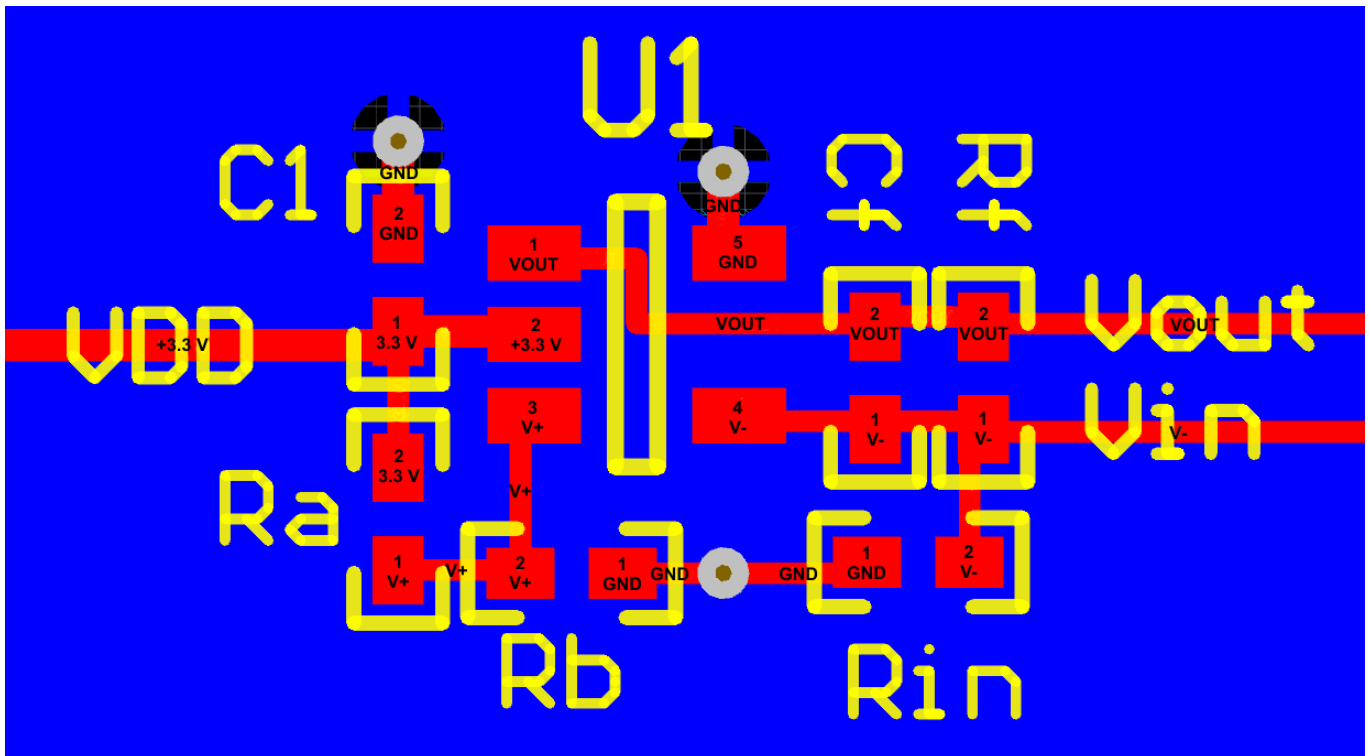
图 7-5. LMC7101Q-Q1 示例布局
