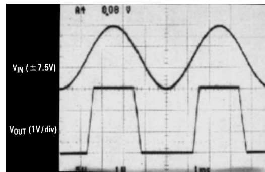
\pm 7.5\text{V} 的输入信号远远超过了图 6-3 中的 3V 电源，但由于 R_i 的原因，未产生相位反转。
