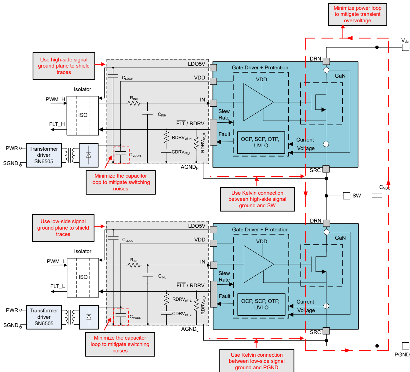
图 9-10. LMG3651R025 典型原理图及布局注意事项
