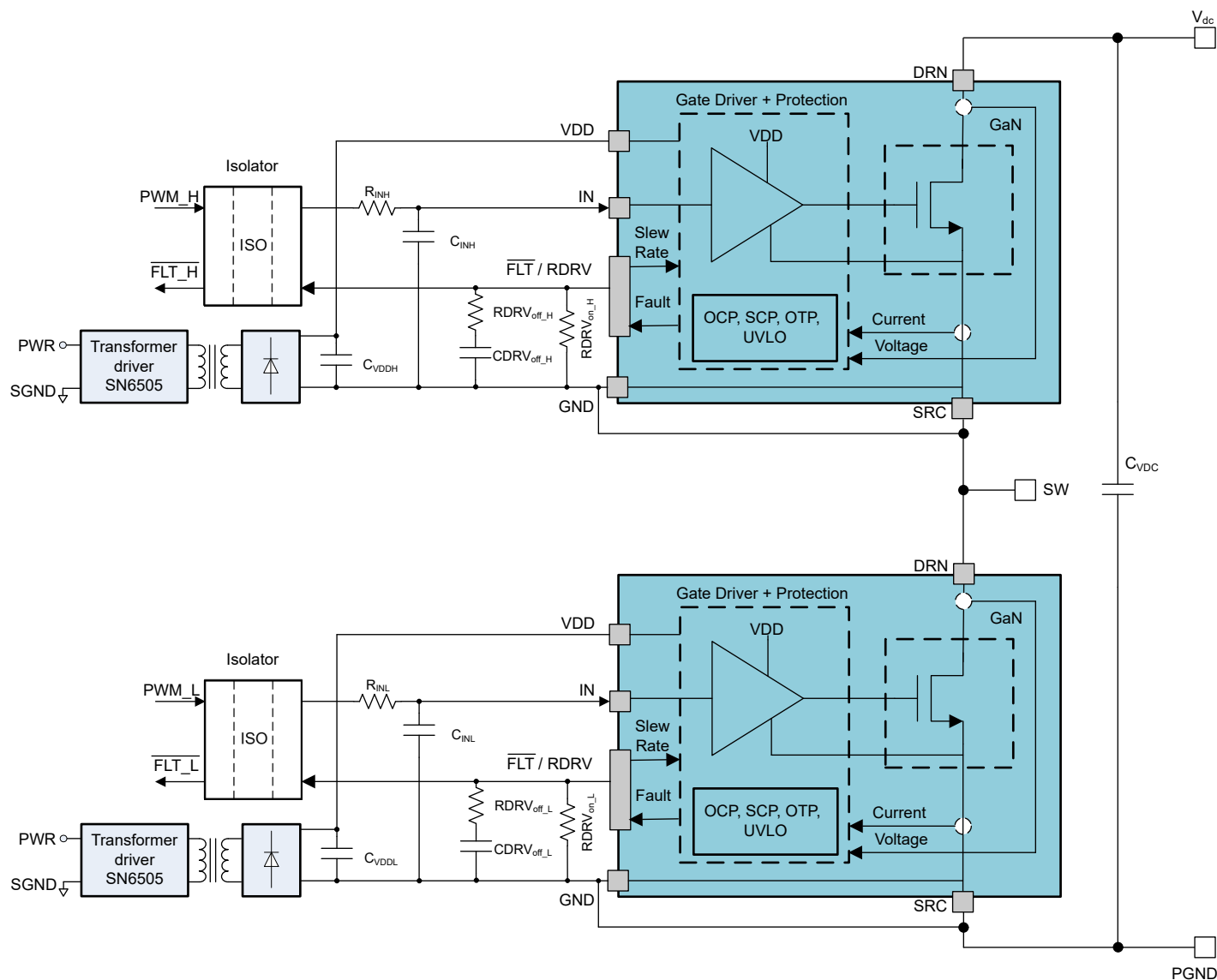
图 9-1. 采用隔离式电源的 LMG3650R025 典型半桥应用
