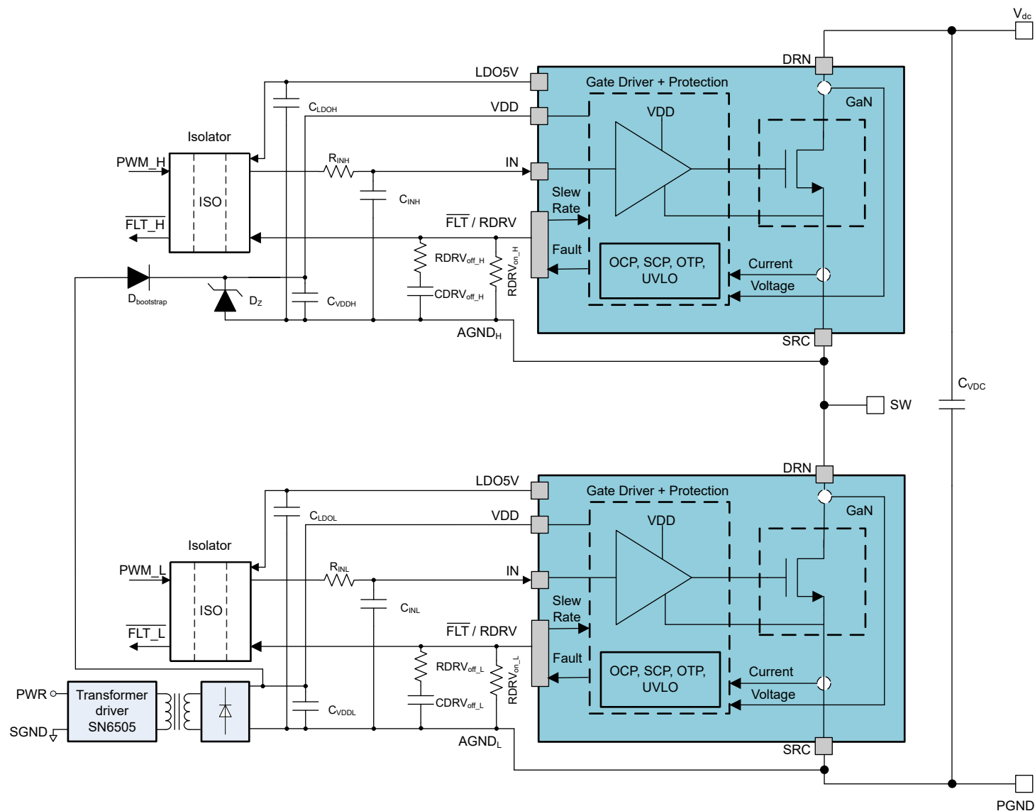
图 9-5. 具有自举功能的 LMG3651R070 典型半桥应用
