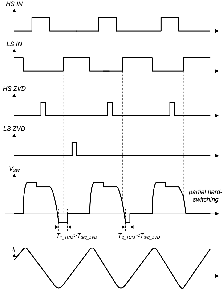
图 8-6. TCM TP PFC 转换器中的 ZVD 功能
