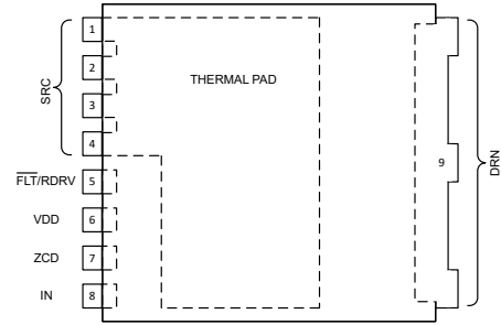
图 5-4. LMG3657R070 , TOLL 封装 (顶视图)
