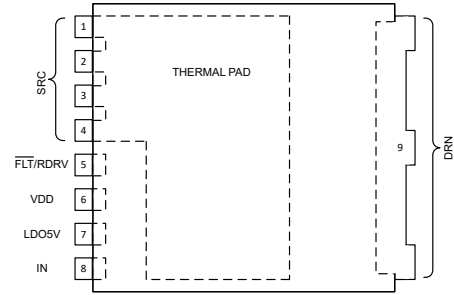
图 5-2. LMG3651R070 , TOLL 封装 (顶视图)
