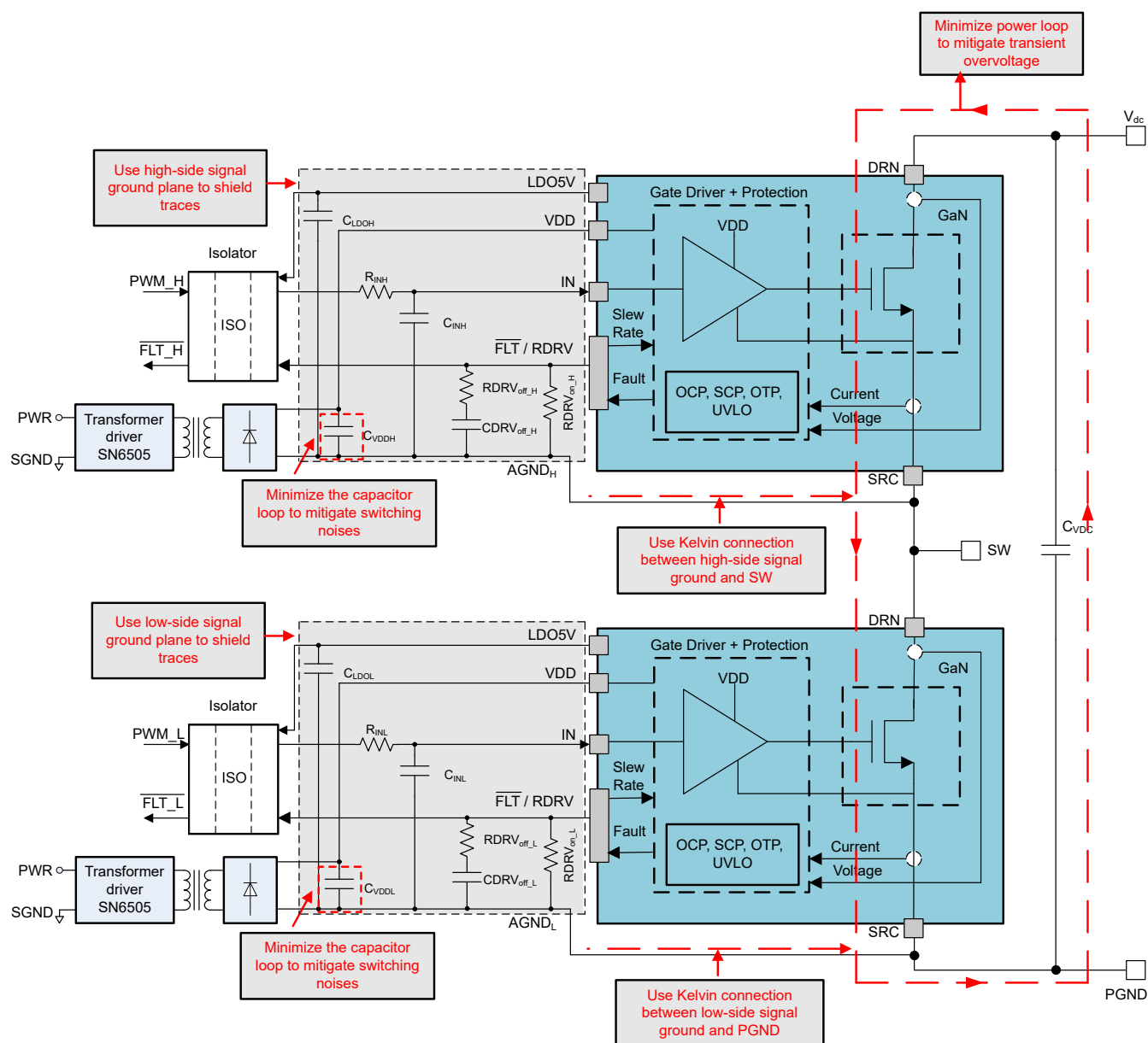
图 9-10. LMG3651R070 典型原理图及布局注意事项
