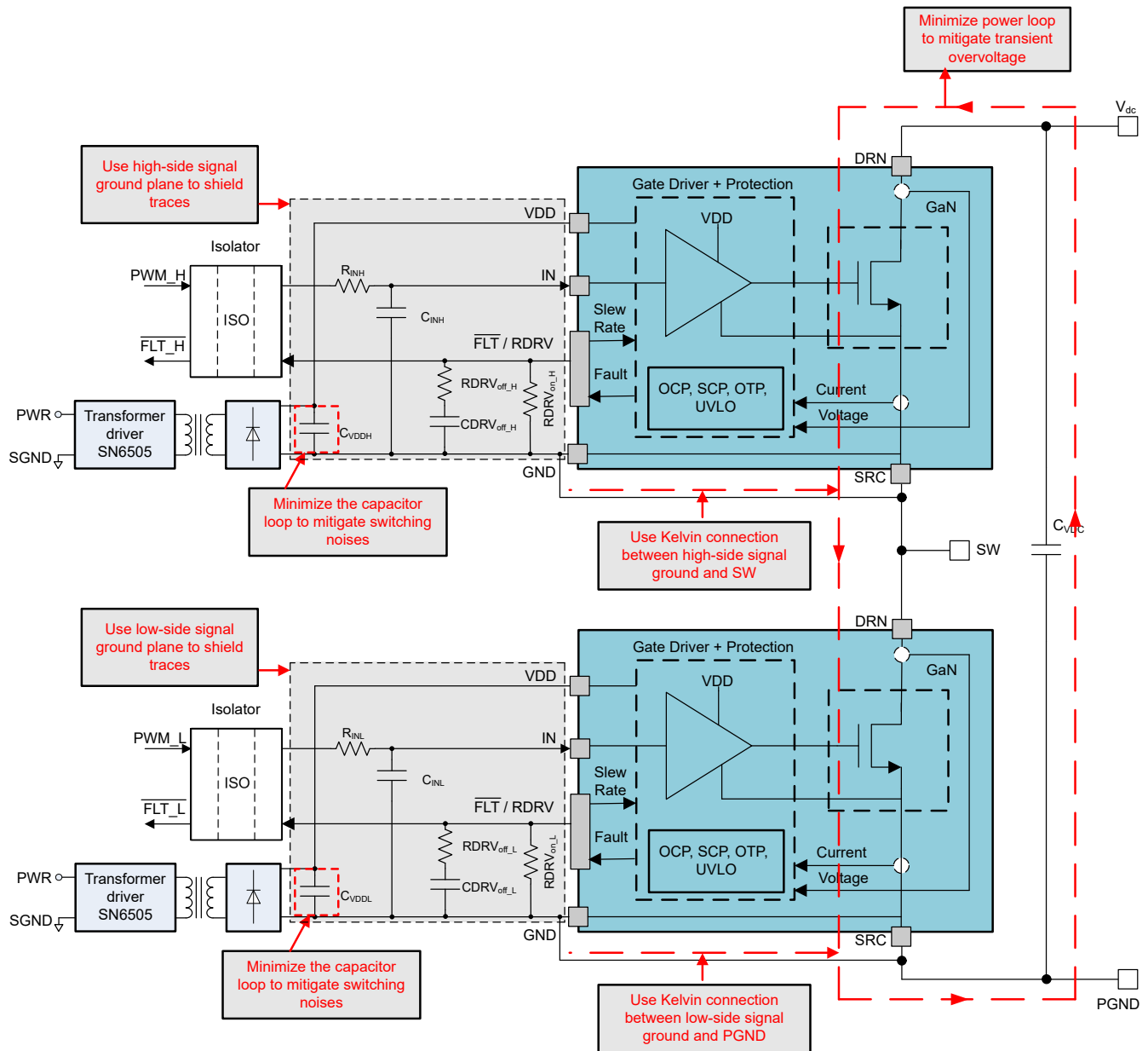
图 9-9. LMG3650R070 典型原理图及布局注意事项
