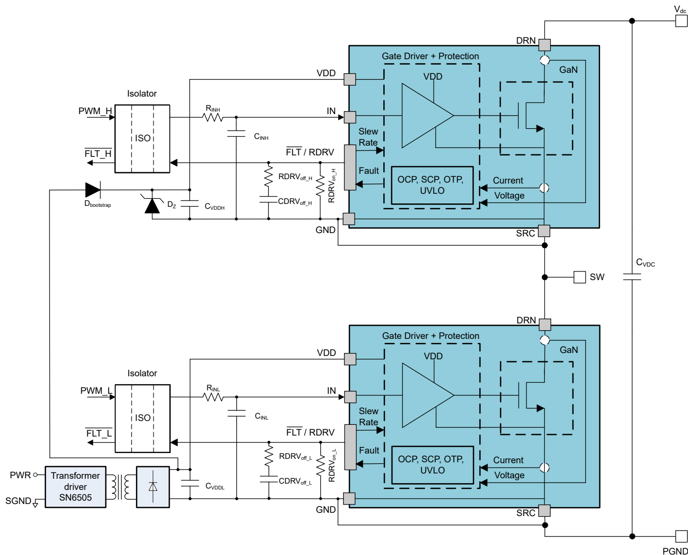
图 9-4. 具有自举功能的 LMG3650R070 典型半桥应用
