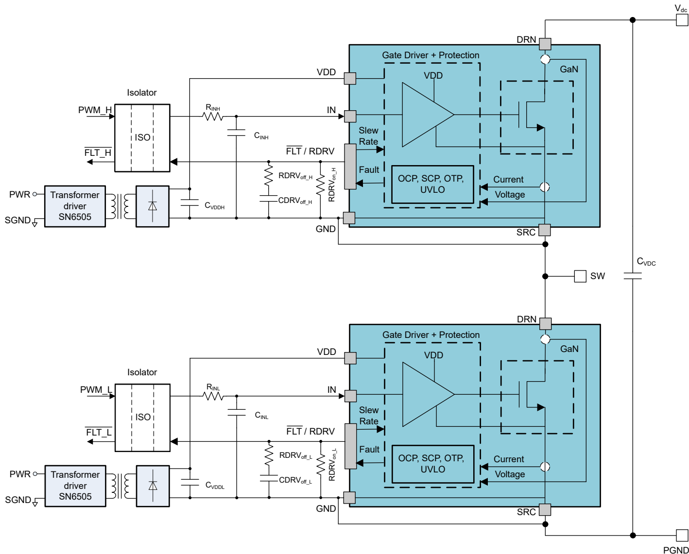
图 9-1. 采用隔离式电源的 LMG3650R070 典型半桥应用
