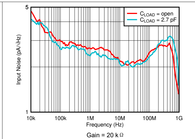
图 6-14. Input Noise Density vs Load Capacitance
