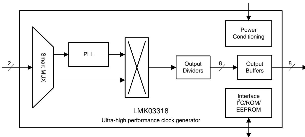
LMK03318 简化框图
