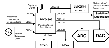
简化 LMK04906 方框图
