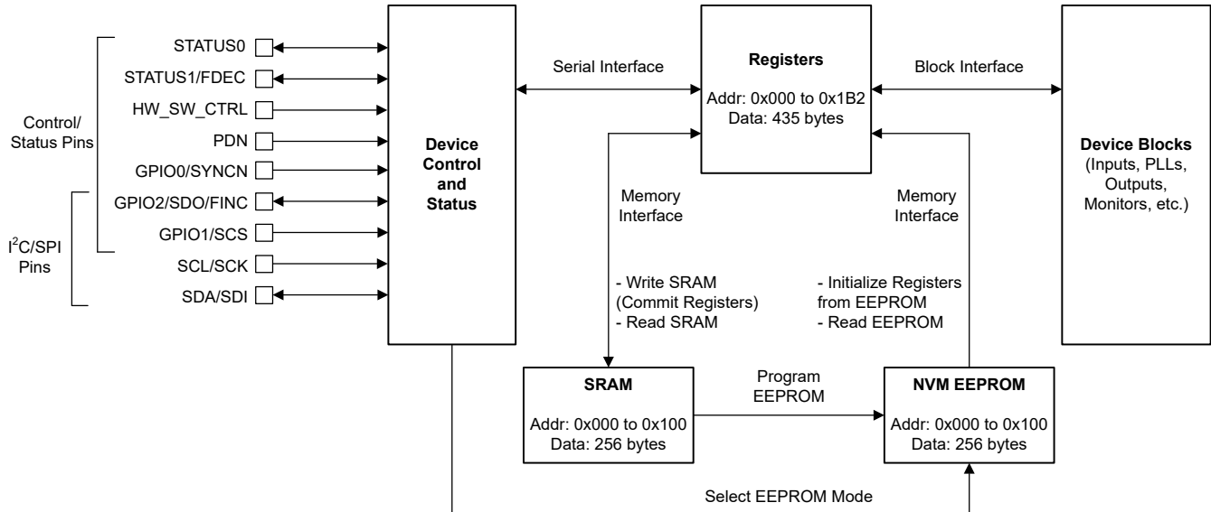
图 7-34. 器件控制、寄存器和存储器接口
