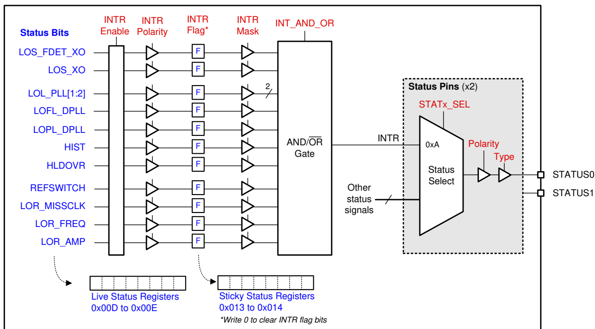
图 7-20. 状态和中断
