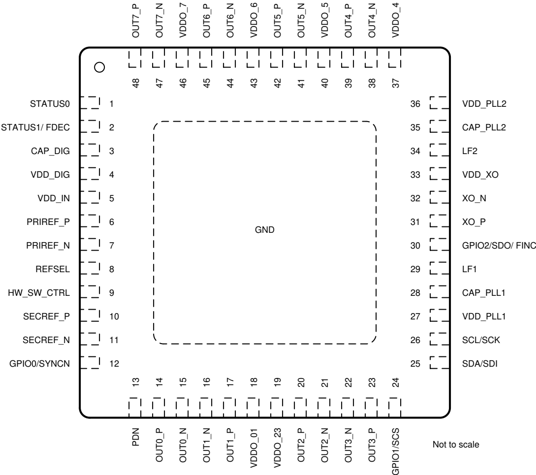
图 4-1. RGZ 封装 48 引脚 VQFN 顶视图
