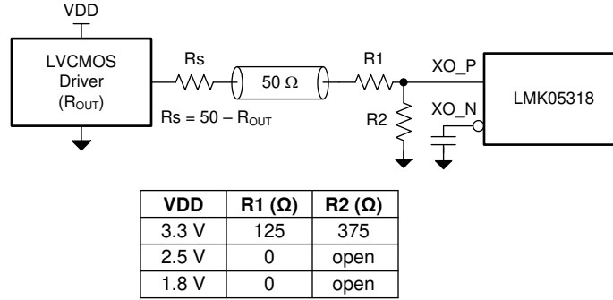
图 7-8. 单端 LVC MOS ( 1.8V、2.5V、3.3V ) 至 XO 输入 (XO_P)
