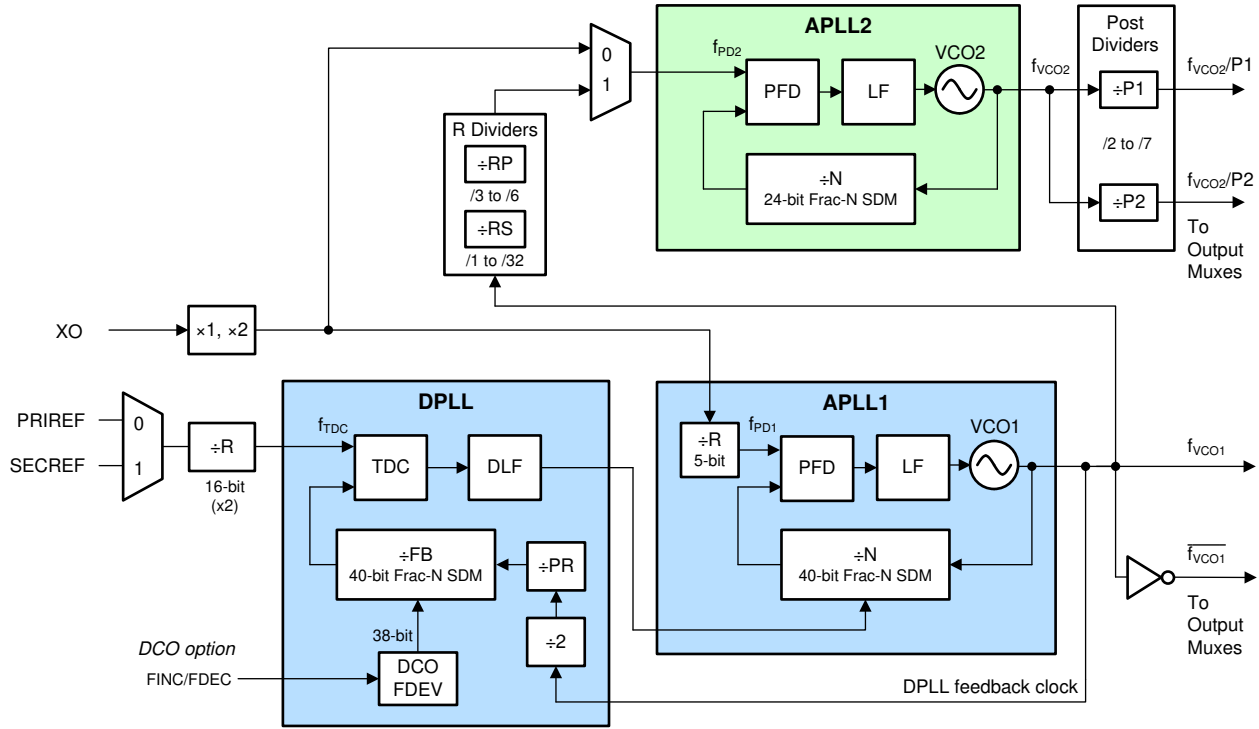
图 7-21. PLL 架构
