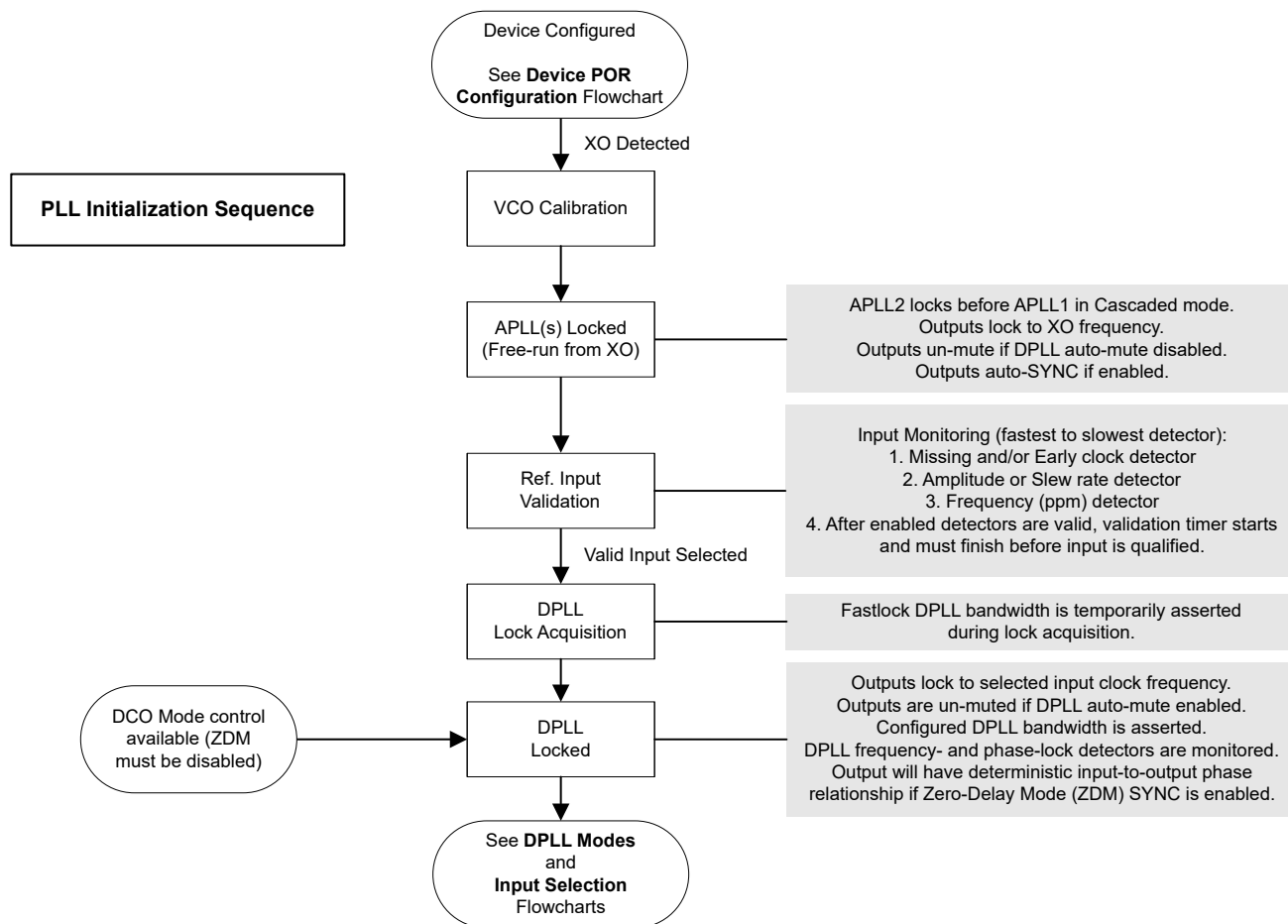
图 7-31. PLL 启动序列
