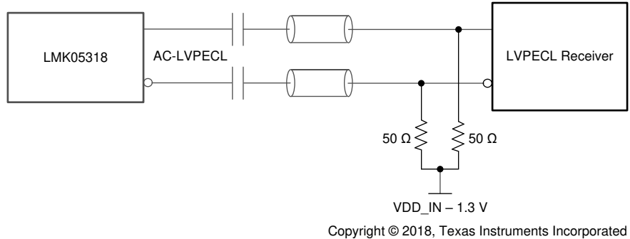
图 7-28. AC-LVPECL 输出至带外部端接/偏置的 LVPECL 接收器
