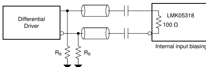
图 7-14. 差分交流耦合至基准 (PRIREF/SECREF) 或 XO 输入
