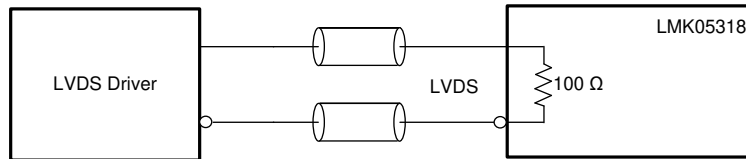
图 7-11. 直流耦合 LVDS 至基准 (PRIREF/SECREP) 或 XO 输入
