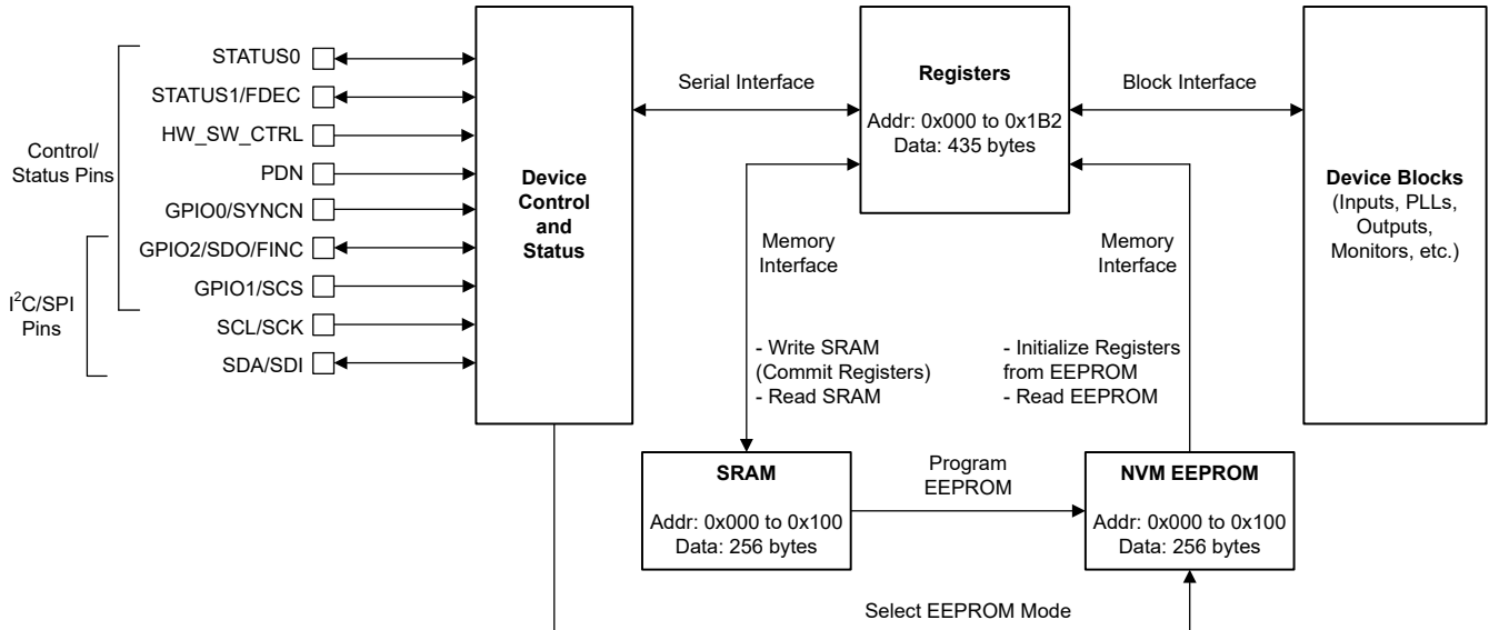
图 8-36. 器件控制、寄存器和存储器接口
