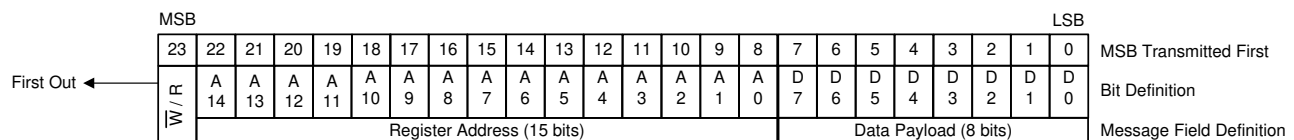
图 8-39. SPI 消息格式
