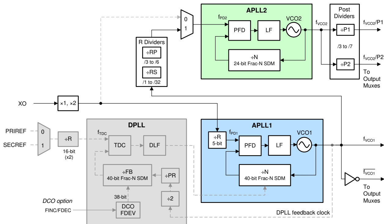
图 8-5. 具有级联 APLL2 的仅 APLL 模式
