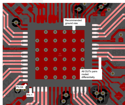
图 9-5. LMK5B33414 的 PCB 布局示例，顶层
