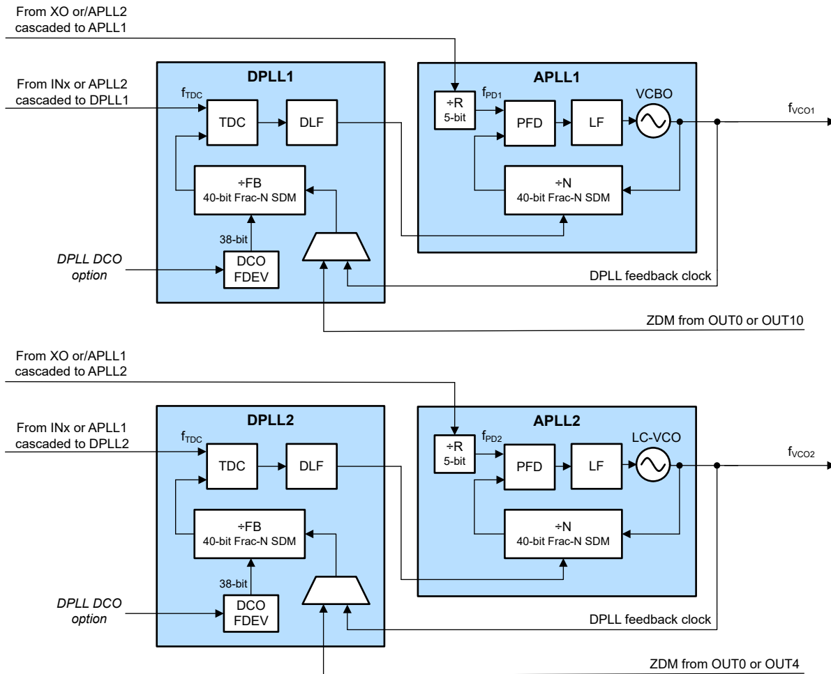
图 7-2. PLL 架构
