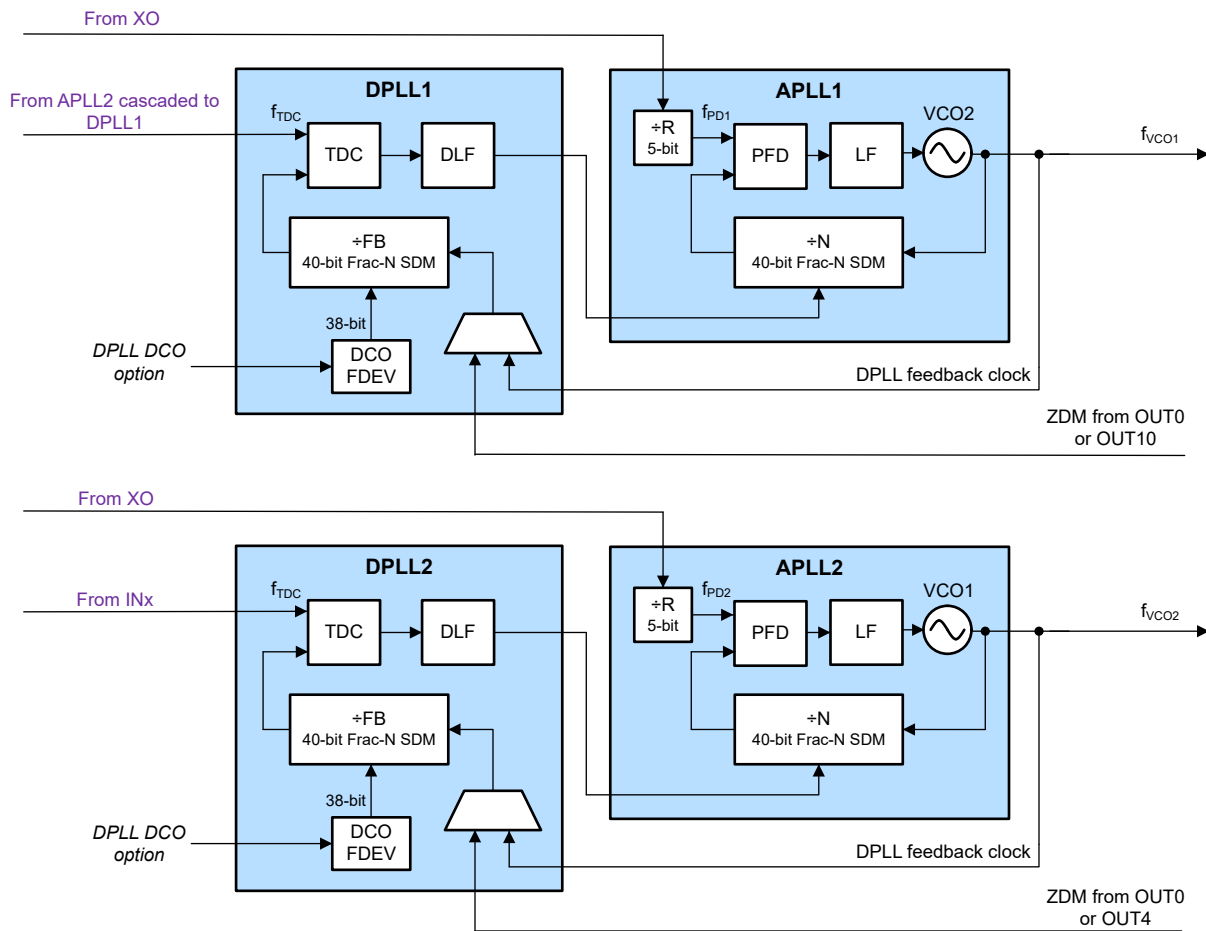
图 7-4. DPLL 级联模式
