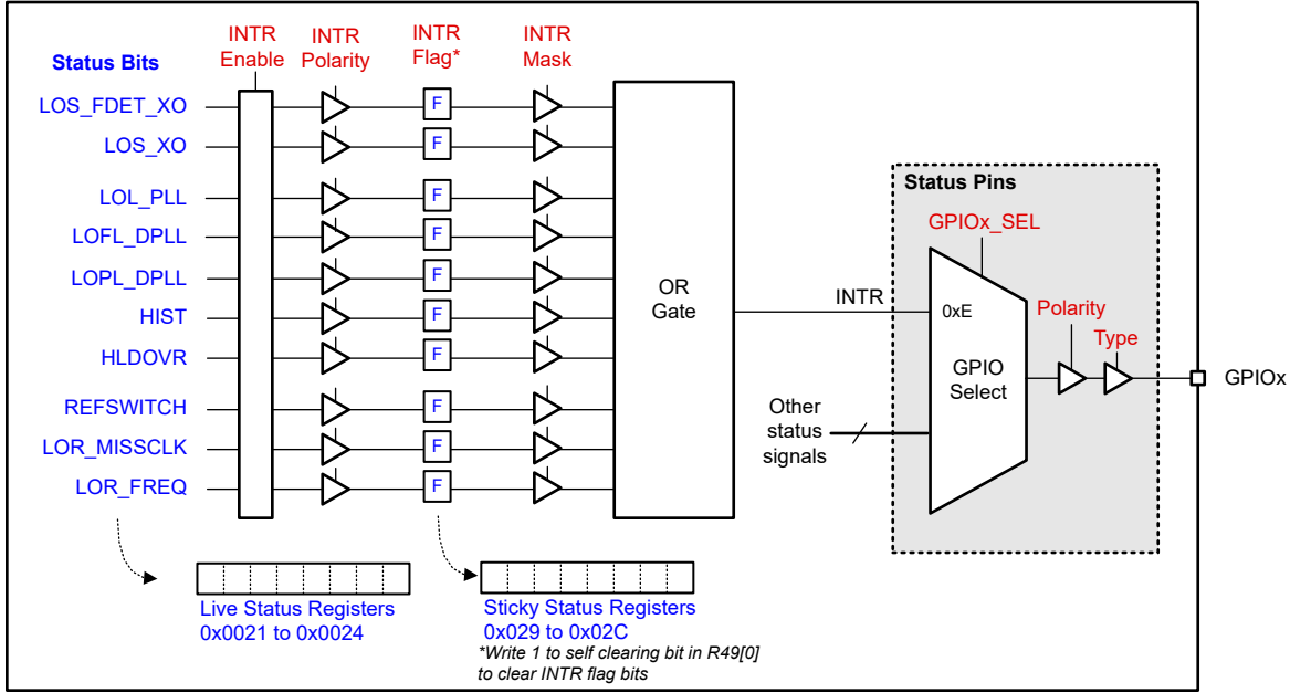
图 7-22. 状态和中断
