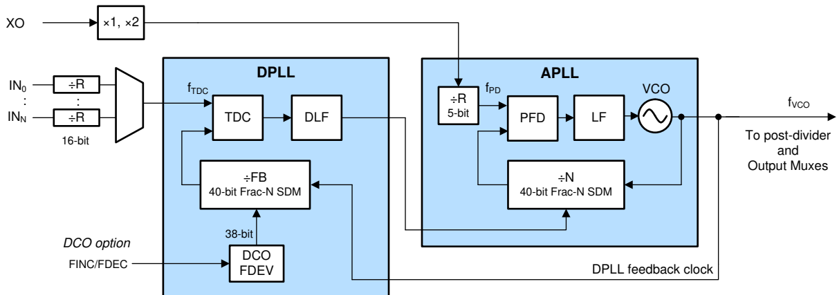
图 7-23. PLL 架构
