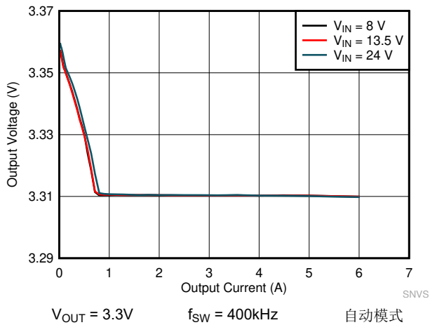
图 9-13. LMQ61460 负载和线性调整率
