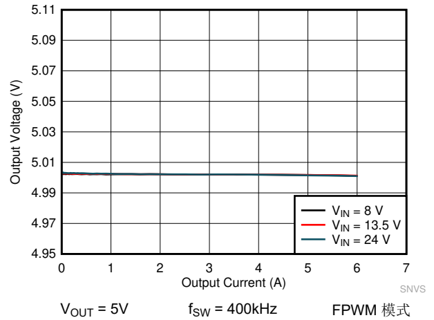
图 9-18. LMQ61460 负载和线性调整率
