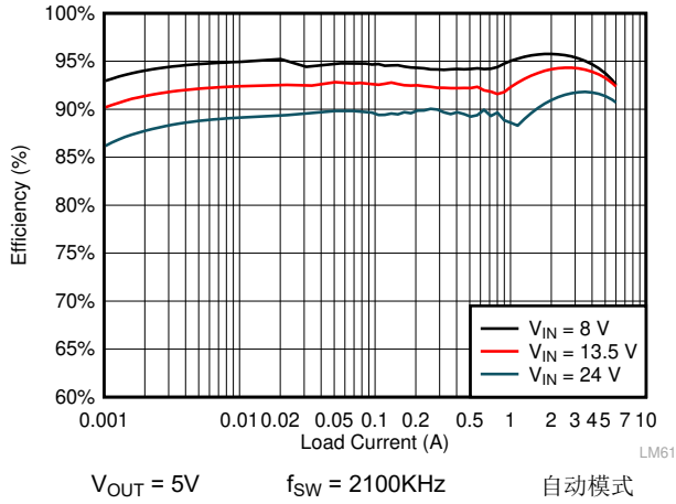
图 9-11. LMQ61460 效率
