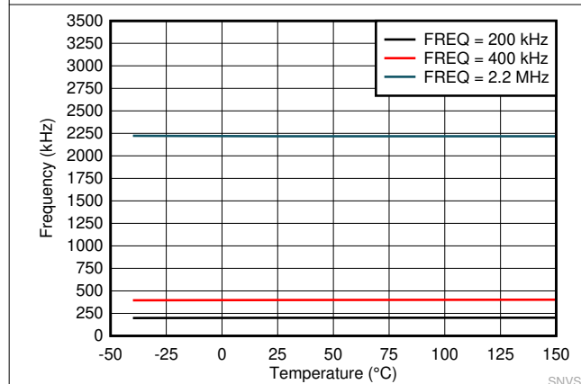
图 7-5. 开关频率
