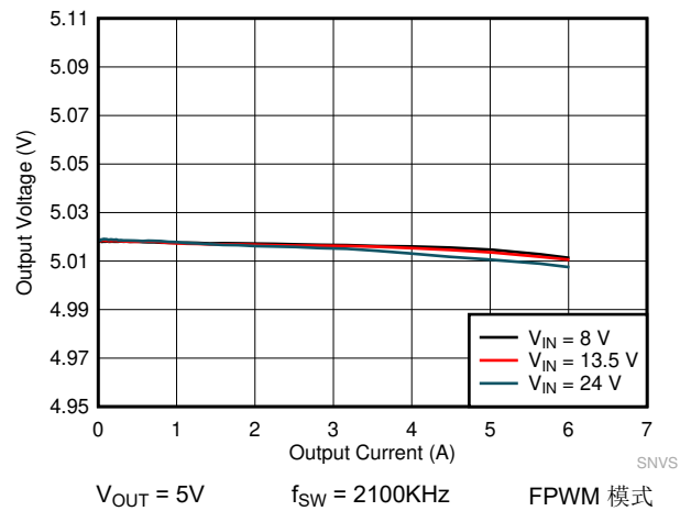
图 9-20. LMQ61460 负载和线性调整率
