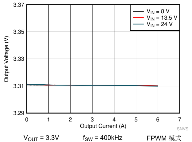
图 9-14. LMQ61460 负载和线性调整率
