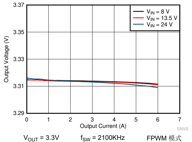
图 9-16. LMQ61460 负载和线性调整率
