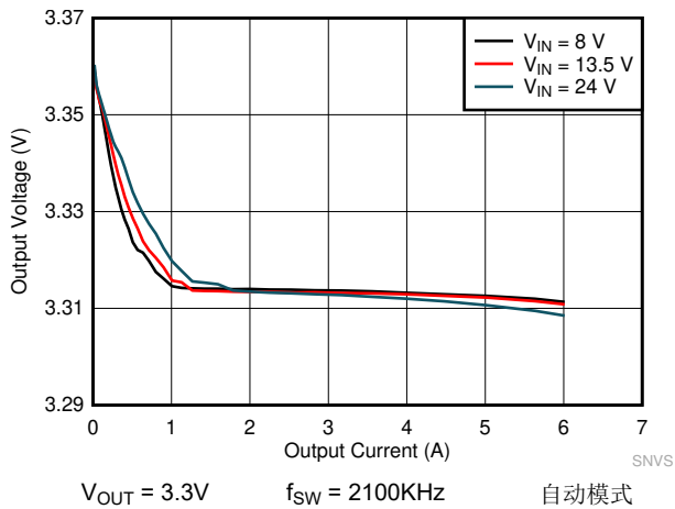
图 9-15. LMQ61460 负载和线性调整率
