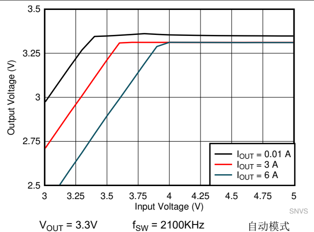
图 9-22. LMQ61460 压降曲线
