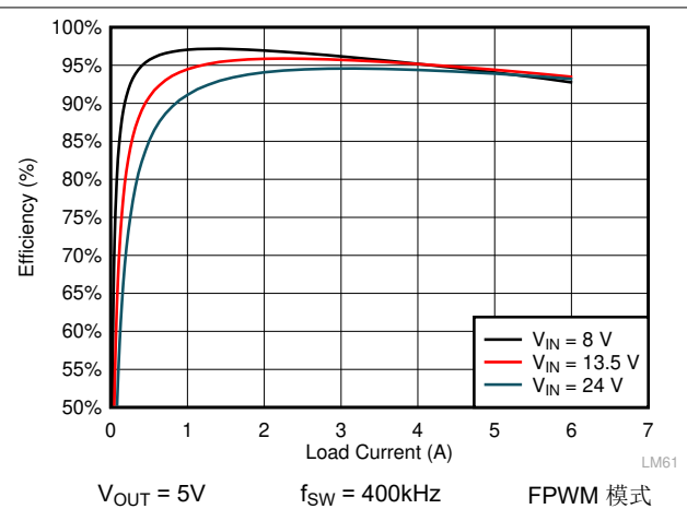
图 9-10. LMQ61460 效率
