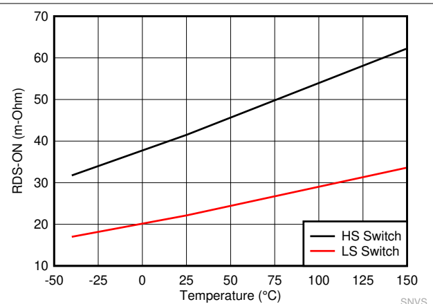
图 7-6. 高侧和低侧开关 R_{DS\_ON}
