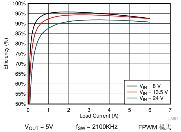
图 9-12. LMQ61460 效率
