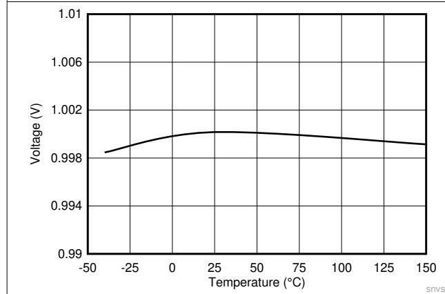
图 7-3. 反馈电压
