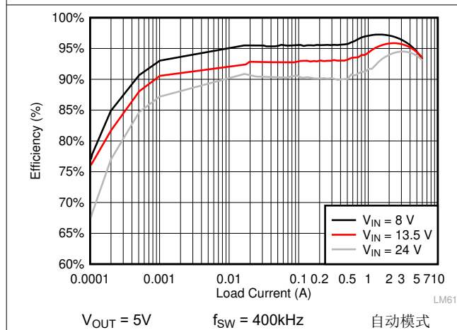
图 9-9. LMQ61460 效率
