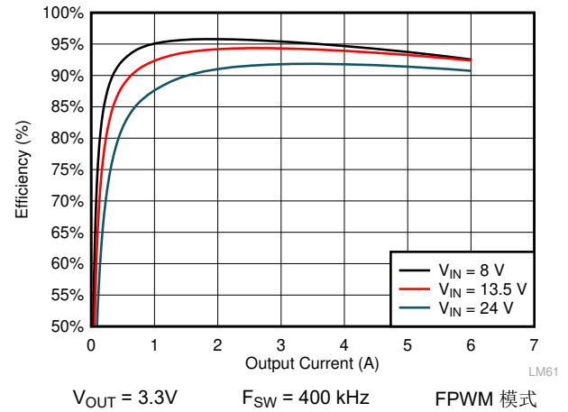
图 10-6. LMQ61460-Q1 效率
