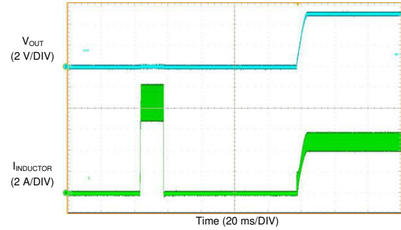
图 9-15. 短路恢复
