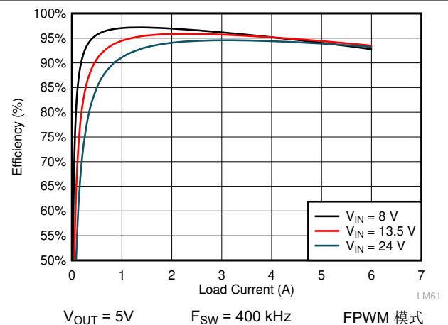
图 10-10. LMQ61460-Q1 效率
