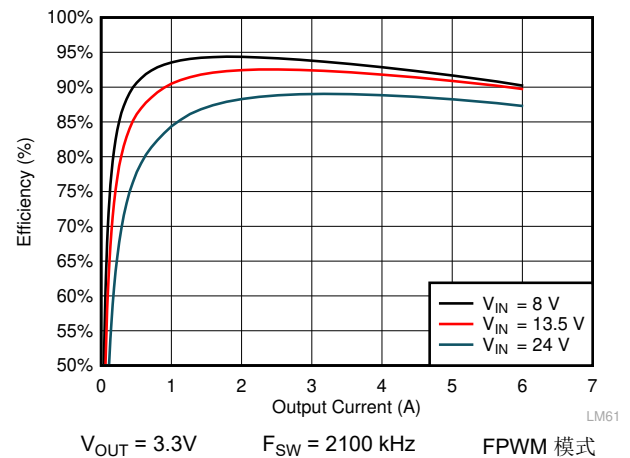
图 10-8. LMQ61460-Q1 效率
