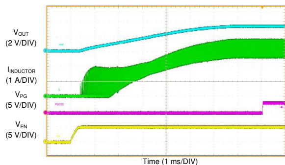
图 10-31. LMQ61460-Q1 在 50mA 负载下启动
