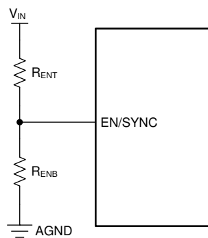
图 10-4. 使用 EN 的 UVLO
