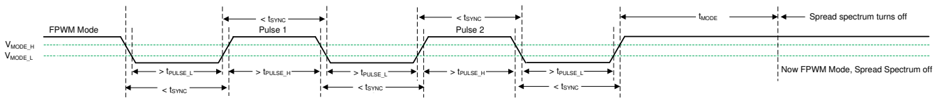
图 8-6. 在 FPWM 模式下禁用展频
