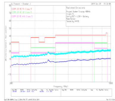
V_{OUT} = 5V F_{SW} = 400\text{ kHz} I_{OUT} = 5\text{ A} 测试频率：300 MHz 至 1 GHz
