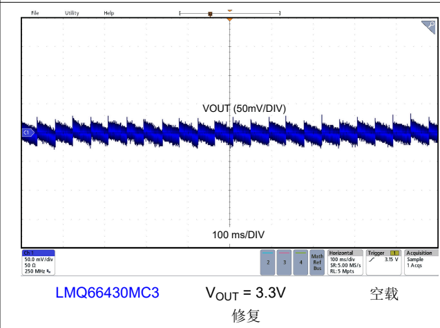
图 8-15. 输出电压纹波
