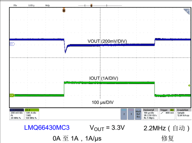
图 8-13. 负载瞬态
