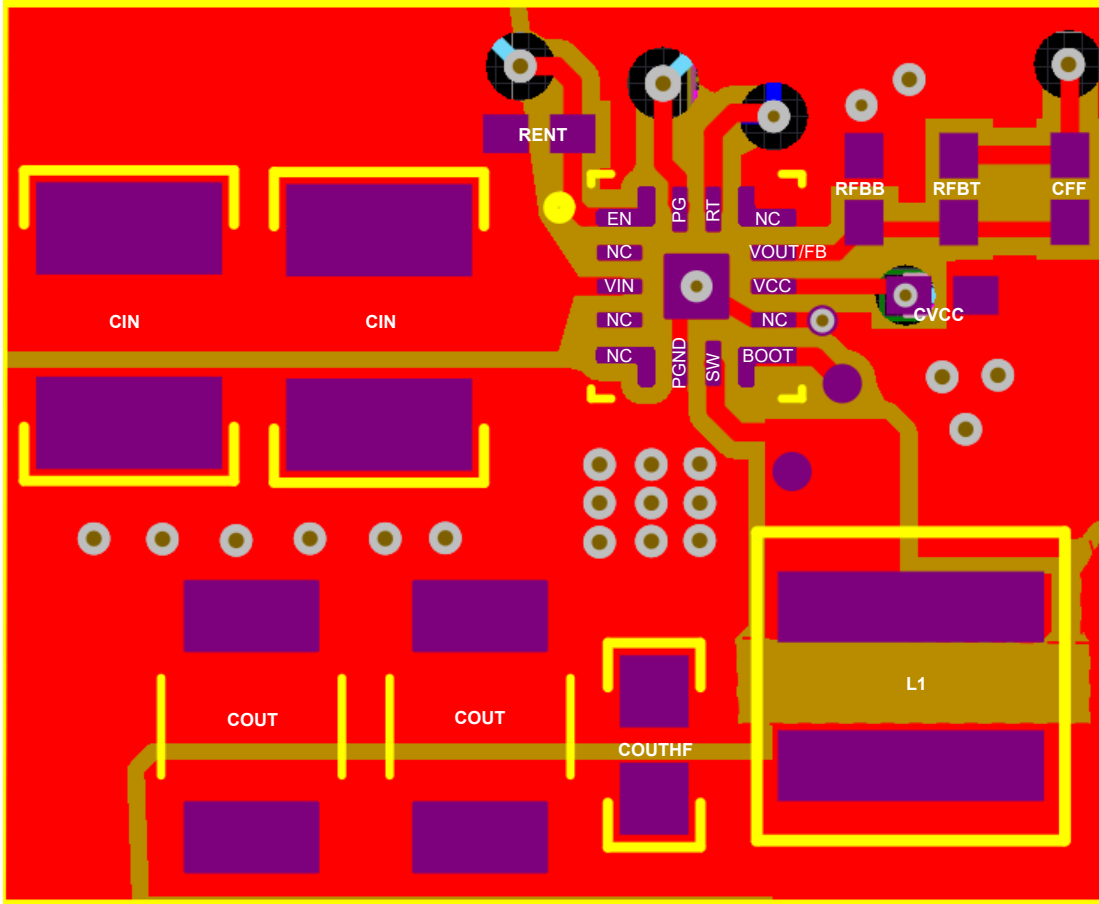
图 8-34. 布局示例
