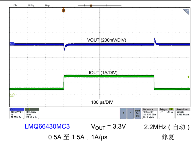
图 8-11. 负载瞬态
