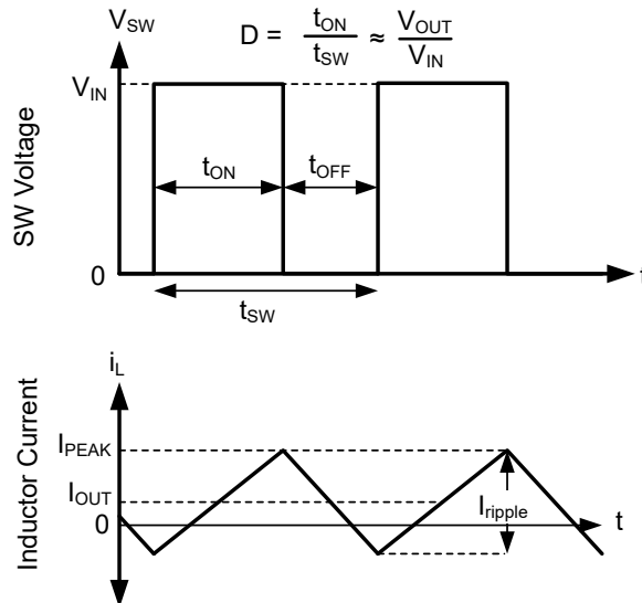
图 7-18. FPWM 模式运行
