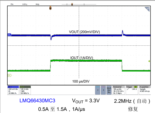
图 8-11. 负载瞬态
