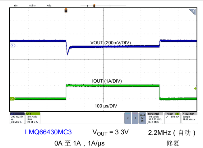
图 8-13. 负载瞬态
