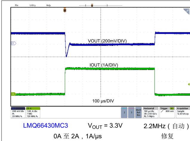
图 8-10. 负载瞬态
