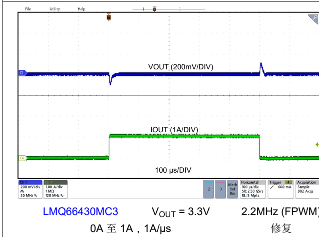
图 8-12. 负载瞬态
