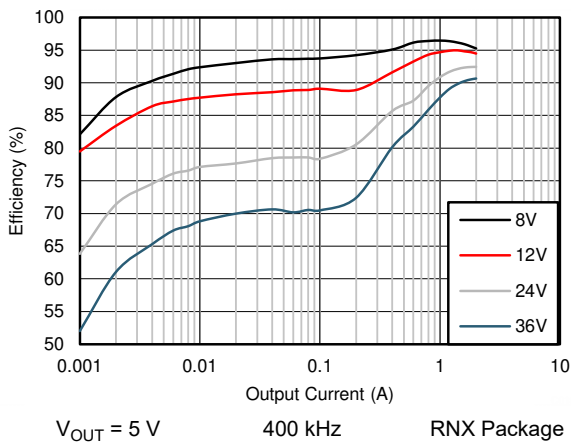
图 8-11. Efficiency
