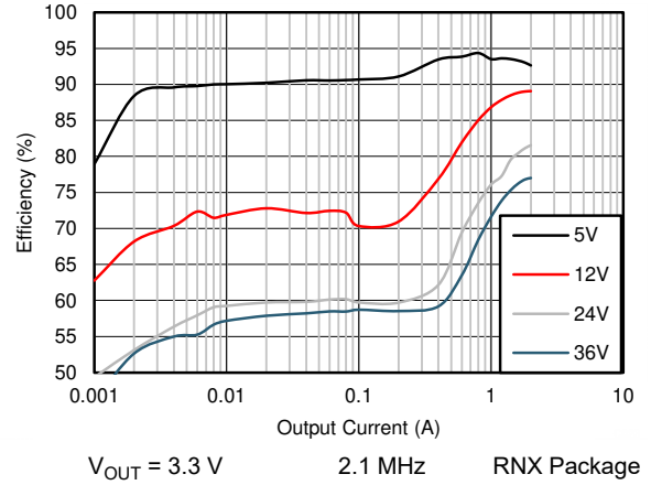
图 8-16. Efficiency
