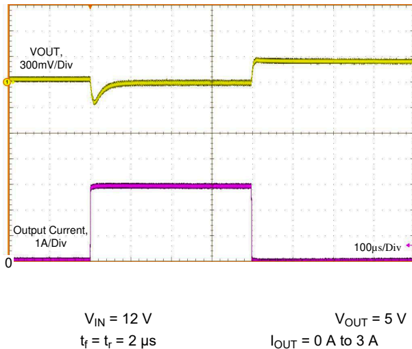
图 8-15. Load Transient
