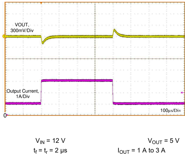
图 8-16. Load Transient
