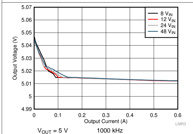
图 23. Load Regulation
