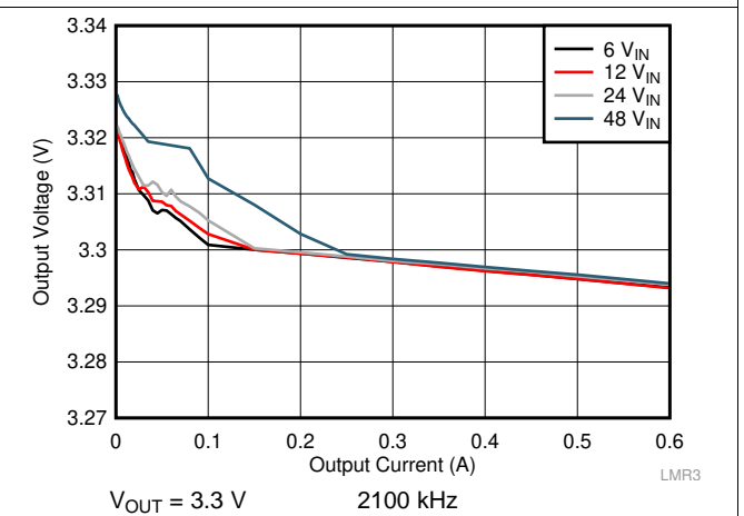
图 46. Load Regulation
