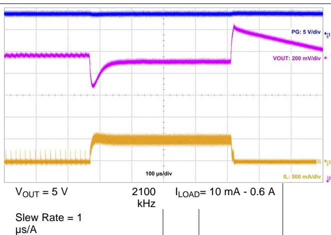
图 54. Load Transient
