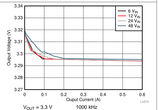
图 24. Load Regulation
