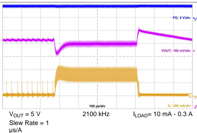
图 52. Load Transient
