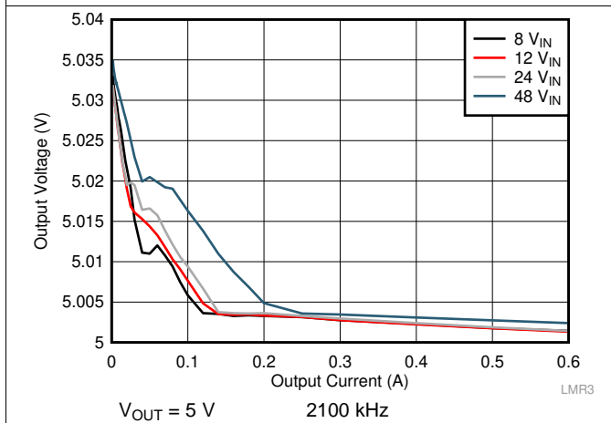
图 45. Load Regulation
