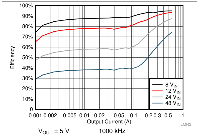
图 21. Efficiency
