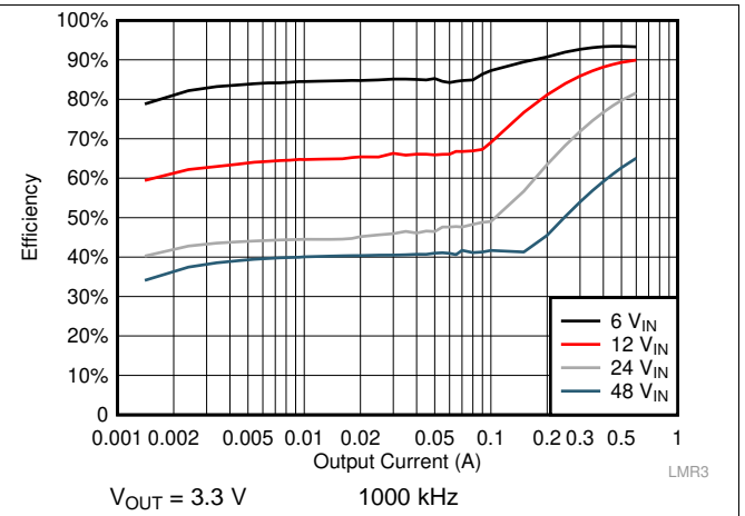
图 22. Efficiency
