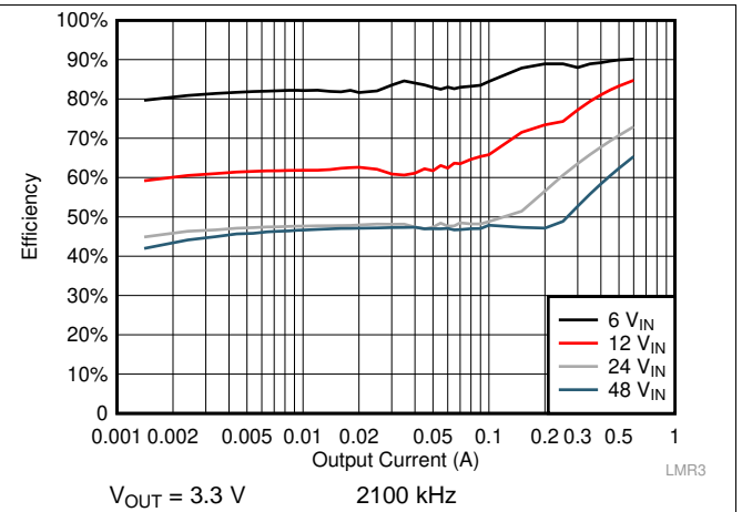
图 44. Efficiency
