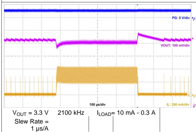
图 53. Load Transient
