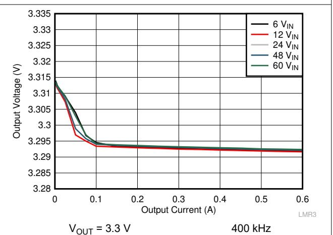
图 9-8. Load Regulation
