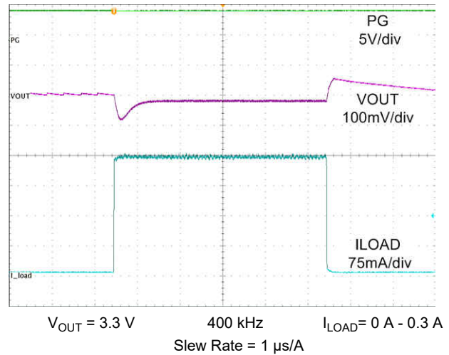
图 9-16. Load Transient
