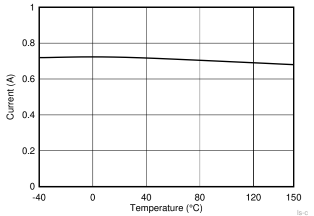
图 7-4. Low Side Current Limit
