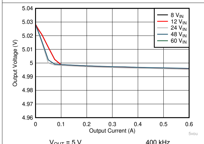
图 9-7. Load Regulation
