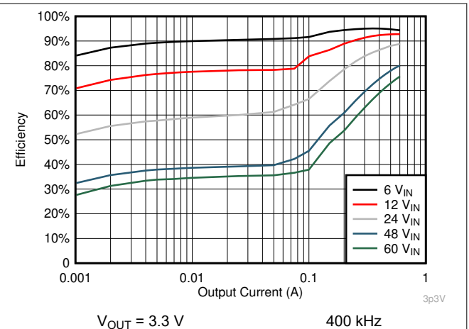
图 9-6. Efficiency
