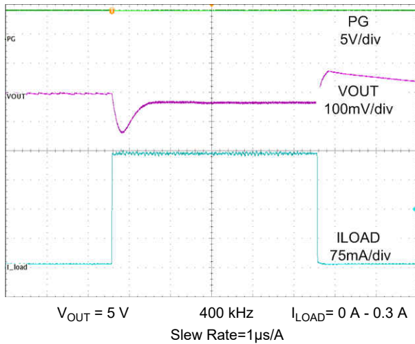
图 9-15. Load Transient
