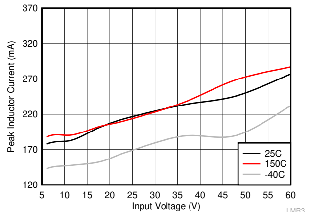
图 7-4. Low Side Current Limit
