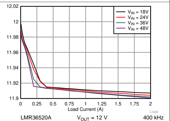
图 21. Load Regulation
