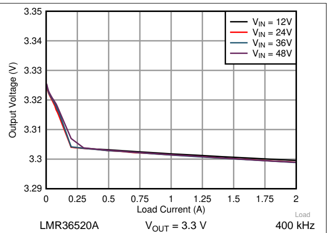
图 17. Load Regulation
