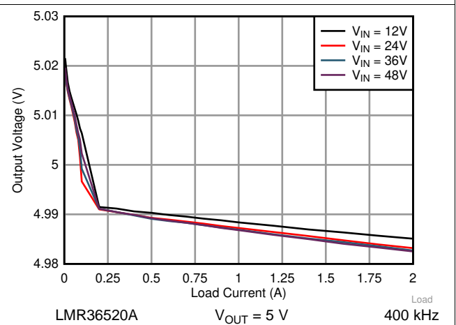
图 19. Load Regulation
