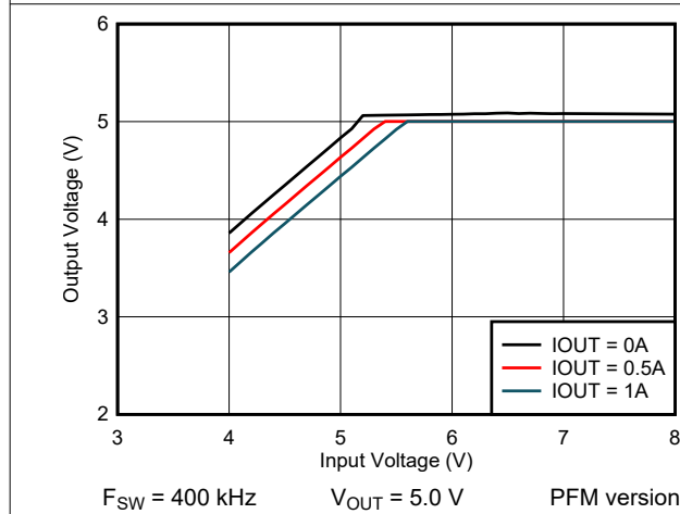
图 6-3. 5-V Dropout
