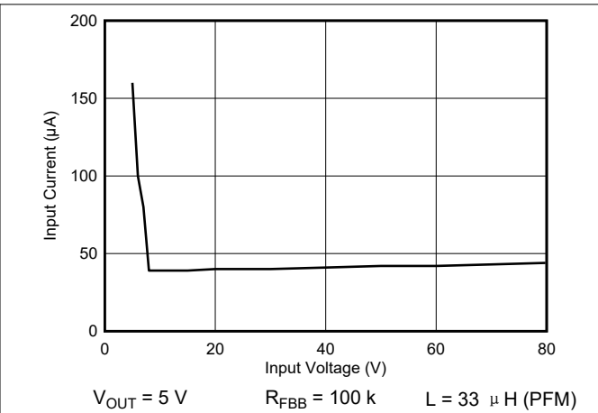
图 6-2. No Load Input Current vs Input Voltage
