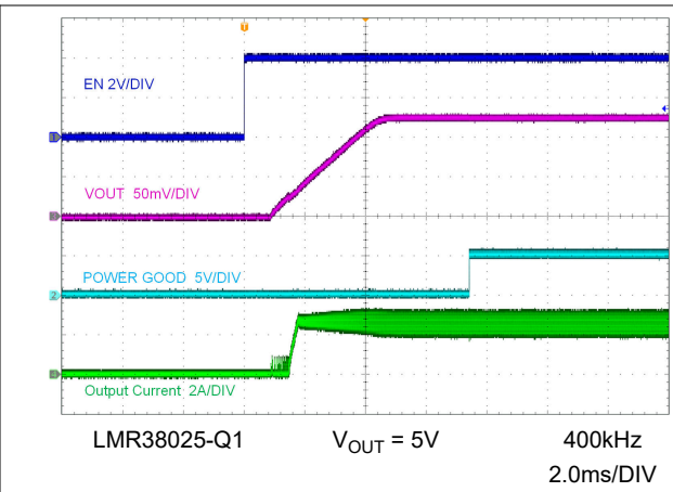
图 8-4. 由 EN 启动
