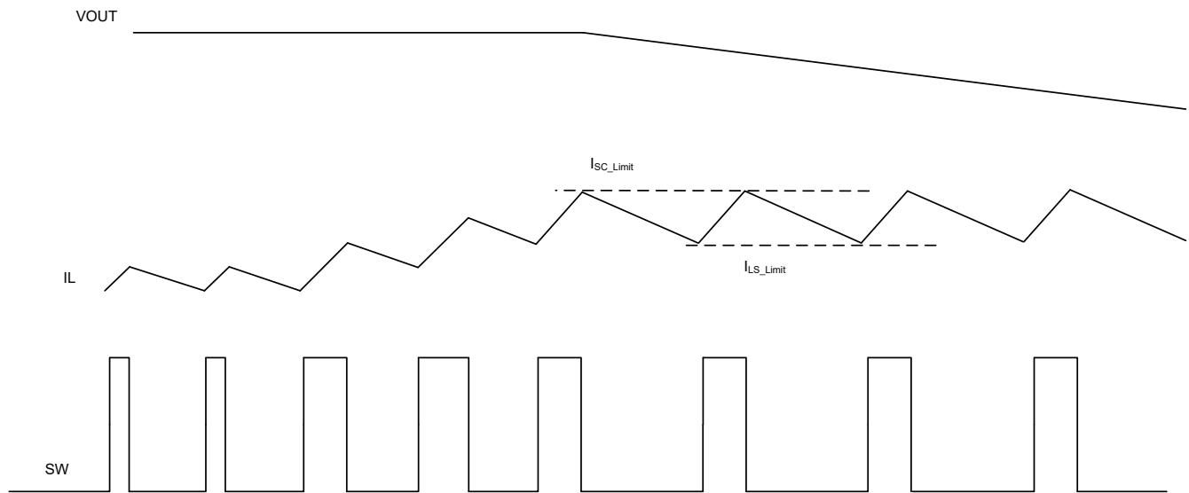
图 7-10. 对负载阶跃的过流响应
