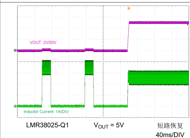
图 8-8. 短路恢复
