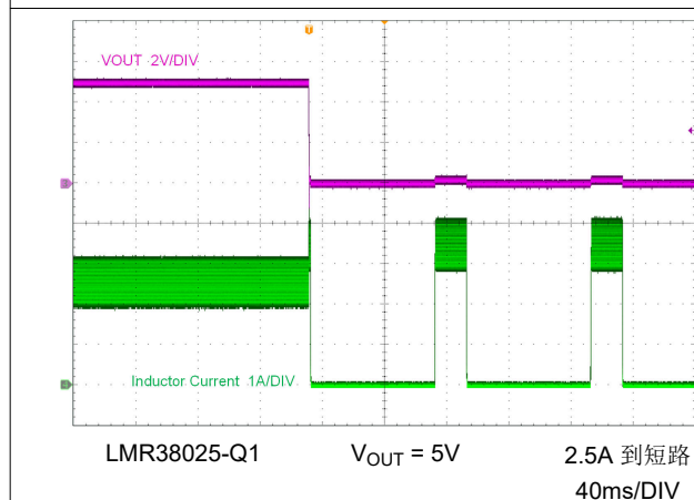
图 8-7. 应用短路
