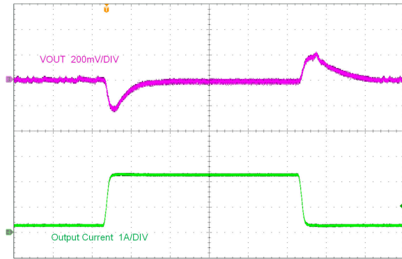
LMR38025-Q1(PFM) V_{OUT} = 5V 400kHz, (交流耦合) 100 \mu s/DIV 200mA/ \mu s 时为 250mA 至 2.25A
