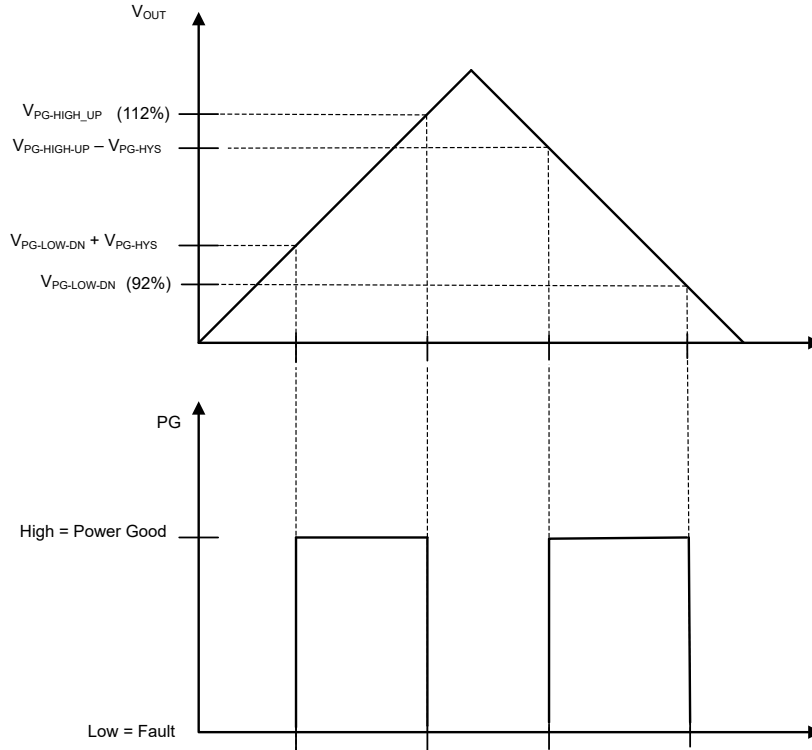
图 7-6. 静态电源正常运行
