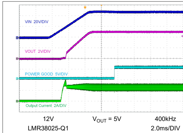
图 8-3. 由 VIN 启动
