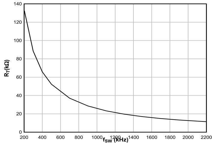
图 7-4. R T 与频率曲线间的关系
