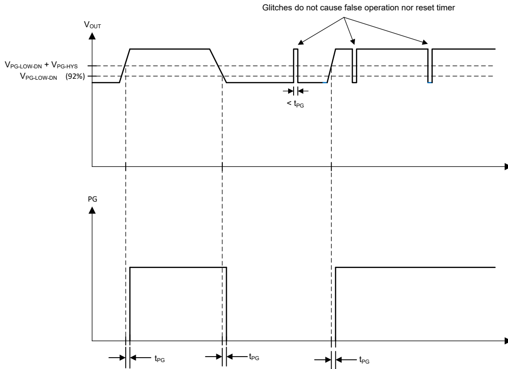
图 7-7. 电源正常时序行为
