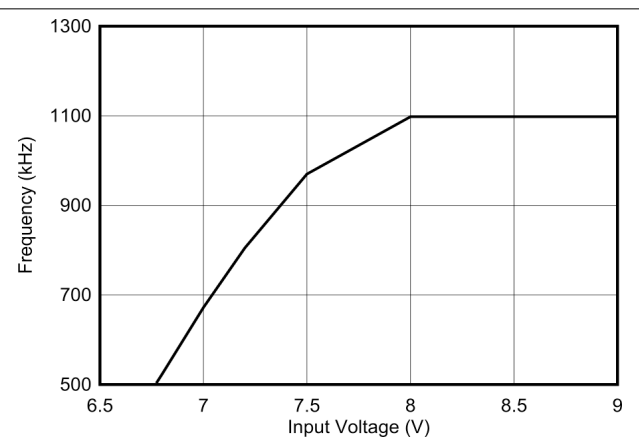
图 7-9. T_{OFF\_MIN} 时的典型频率折返
