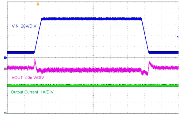
LMR38025-Q1(PFM) V_{OUT} = 5V 400kHz (交流耦合) 800 \mu s/DIV 200V/ms 时为 10V 至 70V
