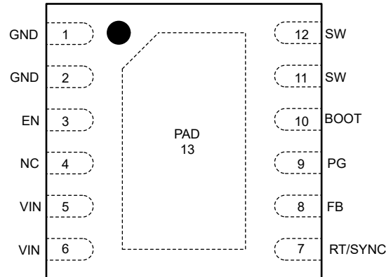
图 5-1. DRR 封装，12 引脚 WSON (俯视图)
