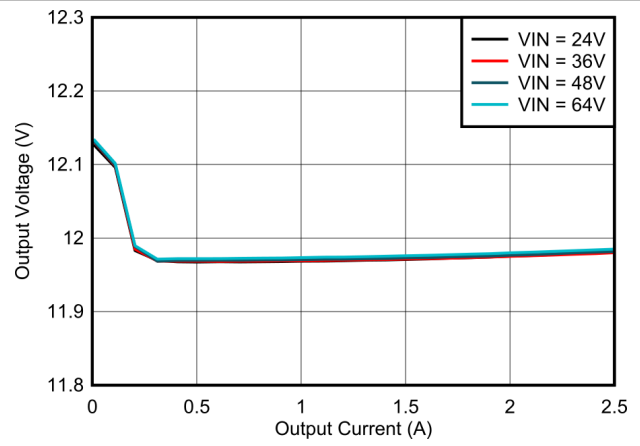
LMR38025-Q1 V_{OUT} = 12V 400kHz PFM 版本
