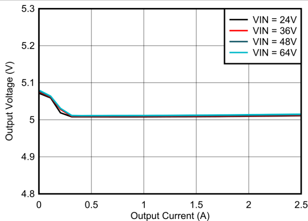
LMR38025-Q1 V_{OUT} = 5V 400kHz PFM 版本
