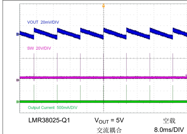
图 8-5. PFM 开关
