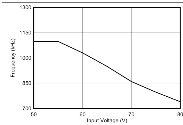
图 7-8. T_{ON\_MIN} 时的典型频率折返
