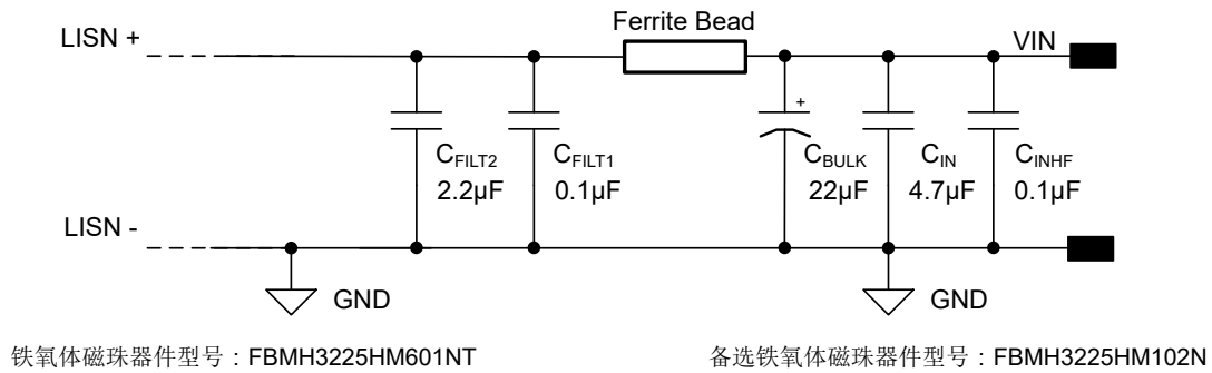
图 8-26. 典型输入 EMI 滤波器
