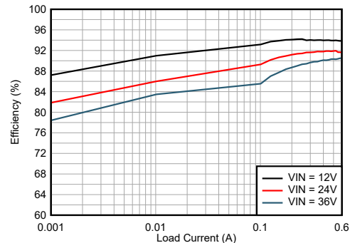
效率： V_{\text{OUT}} = 5\text{V} (固定值)、400kHz
