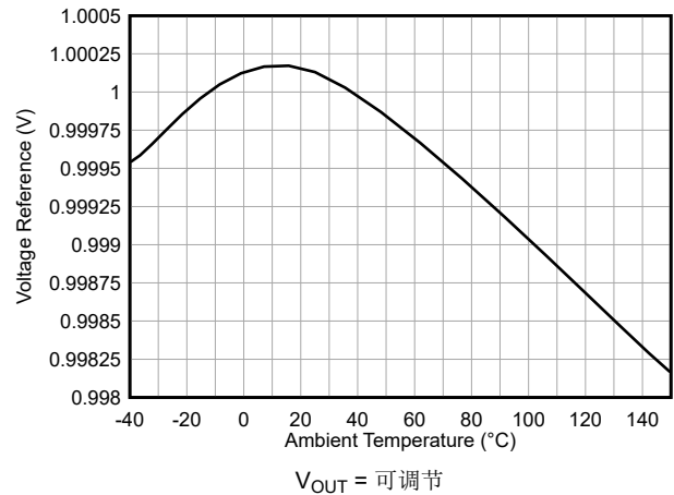
图 6-4. 反馈电压精度与温度间的关系
