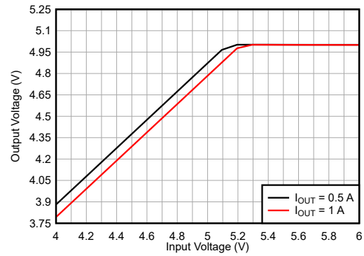
LMR43610MSC5 V_{OUT} = 5V 2.2MHz (自动) 固定
