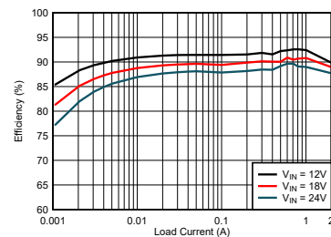
效率： V_{\text{OUT}} = 3.3\text{V} (固定值)、 2.2\text{MHz}
