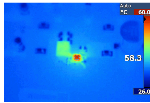
LMR43620MSC3 24V IN , 2A, 2.2MHz V_{OUT} = 3.3V 固定
