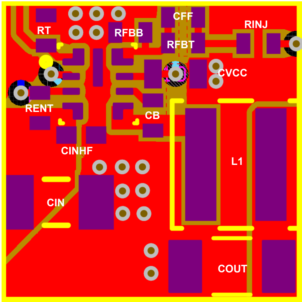
图 8-32. 示例布局
