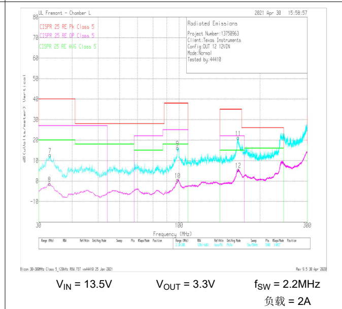
图 8-28. 典型 CISPR 25 辐射 EMI 30MHz - 300MHz 垂直双锥天线，蓝色：峰值检测，粉色 = 平均值检测
