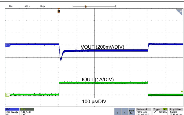
LMR43610MSC5 V_{OUT} = 5V 2.2MHz (自动) 0A 至 1A, 1A/ \mu s 固定
