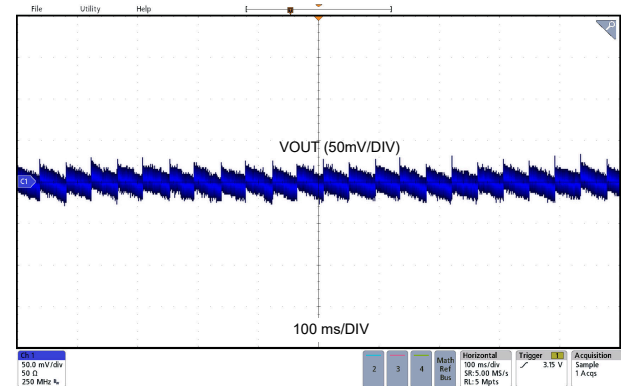
LMR43620MSC3 V_{OUT} = 3.3V 无负载 固定
