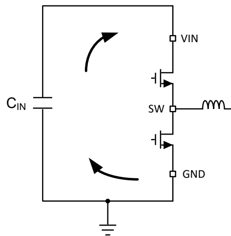
图 8-31. 具有快速边沿的电流环路
