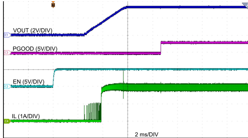
图 7-3. V_{IN} = 12V 、 V_{OUT} = 3.3V 、 I_{OUT} = 2A 时的使能启动
