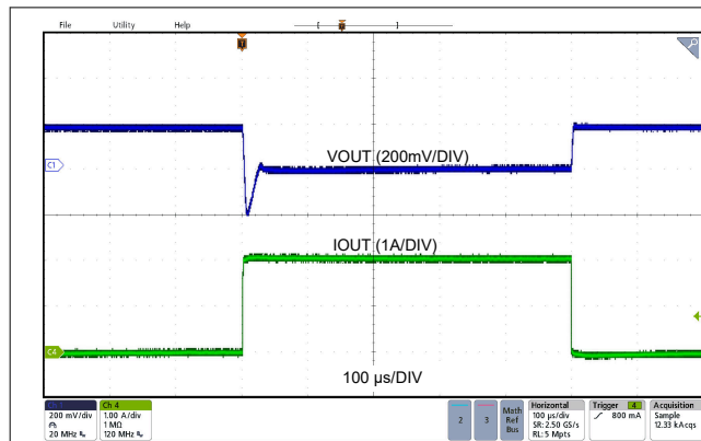
LMR43620MSC3 V_{OUT} = 3.3V 2.2MHz (自动) 0A 至 2A, 1A/ \mu s 固定
