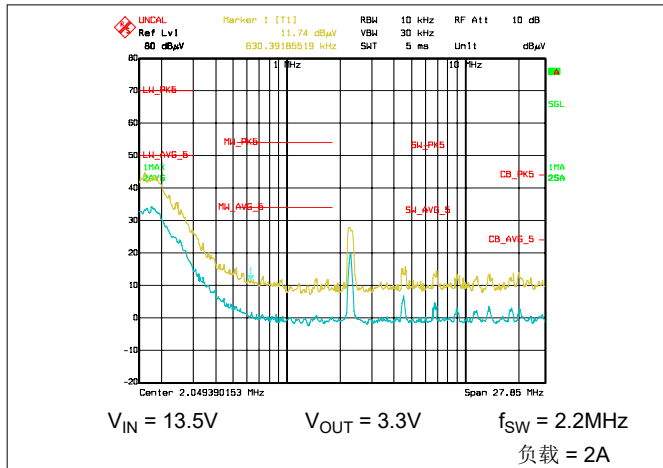
图 8-25. 典型 CISPR 25 传导 EMI 150kHz -30MHz 黄色：峰值检测，蓝色 = 平均值检测
