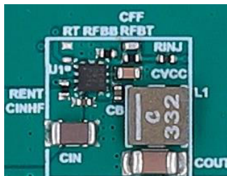
典型设计尺寸 (10mm × 10mm)
