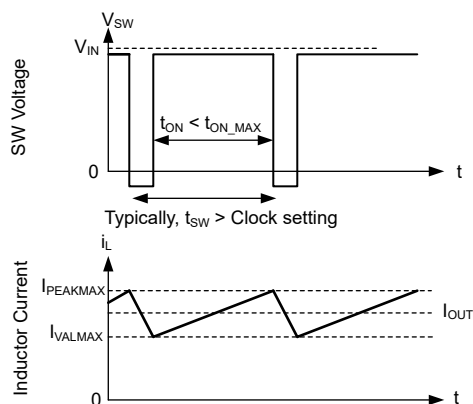
图 7-13. 电流限值波形
