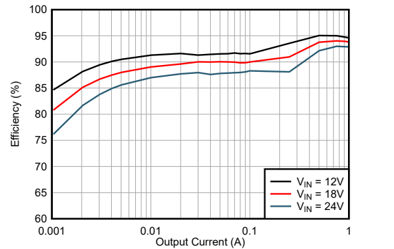
LMR43610RS3 V_{OUT} = 3.3V 400kHz (自动) 固定
