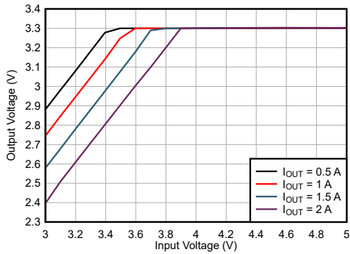
LMR43620MSC3 V_{OUT} = 3.3V 2.2MHz (自动) 固定
