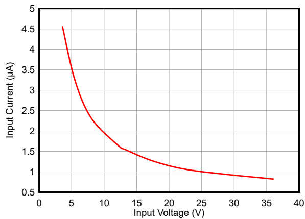
LMR43620MSC3 V_{OUT} = 3.3V 2.2MHz (自动) 固定
