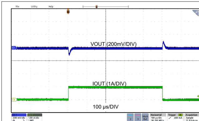
LMR43610MSC5 V_{OUT} = 5V 2.2MHz (FPWM) 0A 至 1A, 1A/ \mu s 固定
