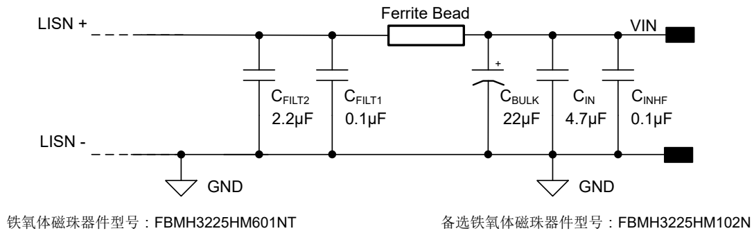
图 8-29. 典型输入 EMI 滤波器
