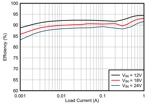
LMR43610MSC5 V_{OUT} = 5V 2.2MHz (自动) 固定
