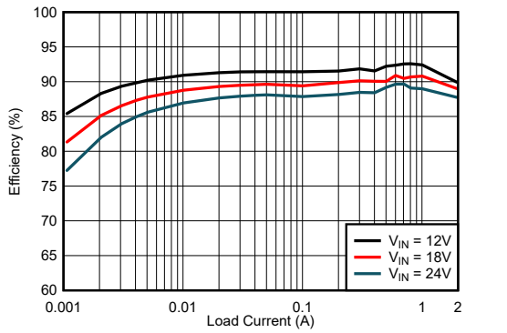
LMR43620MSC3 V_{OUT} = 3.3V 2.2MHz (自动) 固定
