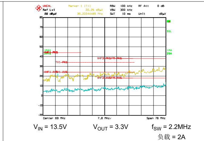
图 8-26. 典型 CISPR 25 传导 EMI 30MHz 至 108MHz 黄色：峰值检测，蓝色 = 平均值检测
