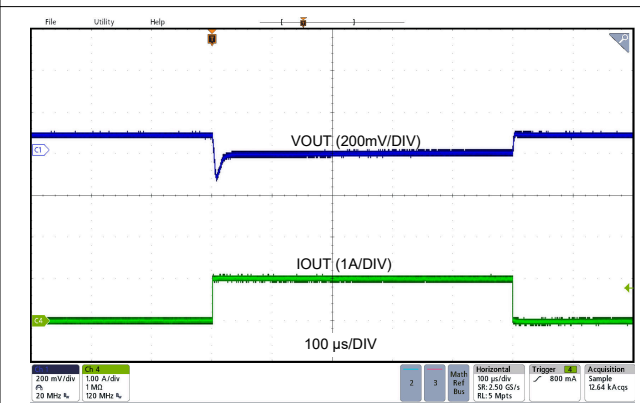
LMR43620MSC3 V_{OUT} = 3.3V 2.2MHz (自动) 0A 至 1A, 1A/ \mu s 固定
