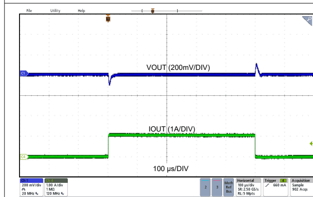
LMR43620MSC3 V_{OUT} = 3.3V 2.2MHz (FPWM) 0A 至 1A, 1A/ \mu s 固定
