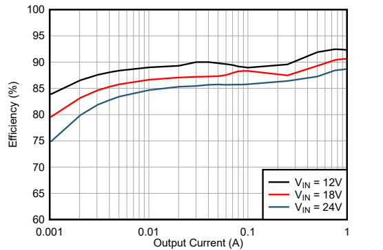
LMR43610RS3 V_{OUT} = 3.3V 1MHz (自动) 固定
