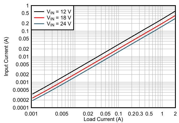
LMR43620MSC3 V_{OUT} = 3.3V 2.2MHz (自动) 固定
