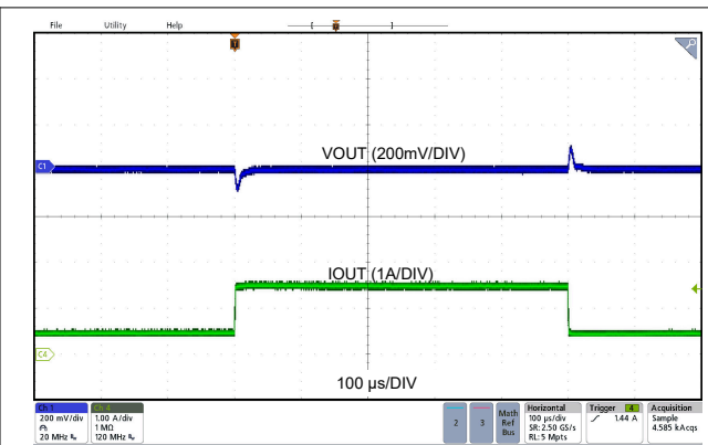
LMR43620MSC3 V_{OUT} = 3.3V 2.2MHz (自动) 0.5A 至 1.5A, 1A/ \mu s 固定
