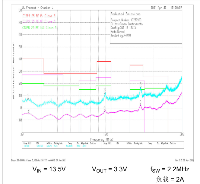
图 8-27. 典型 CISPR 25 辐射 EMI 30MHz - 300MHz 水平双锥天线，蓝色：峰值检测，粉色 = 平均值检测
