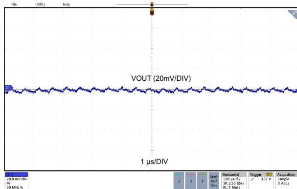
LMR43620MSC3 V_{OUT} = 3.3V 2A 负载 固定
