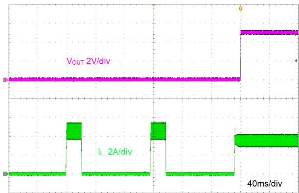
图 8-9. 短路恢复
