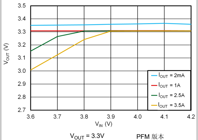
图 6-12. 3.3V 压降
