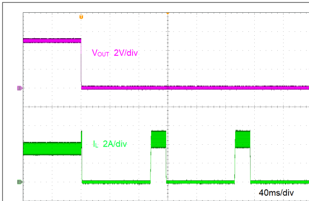
图 8-8. 短路保护
