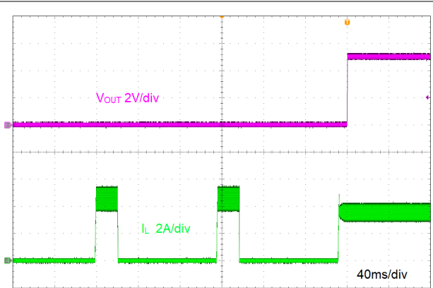
图 8-9. 短路恢复
