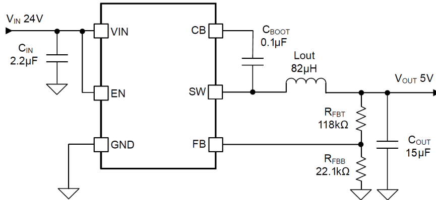
图 8-1. 应用电路
