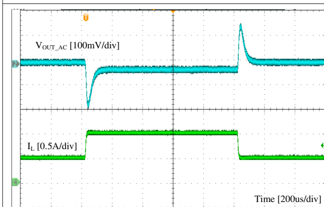
图 8-7. Load Transient
