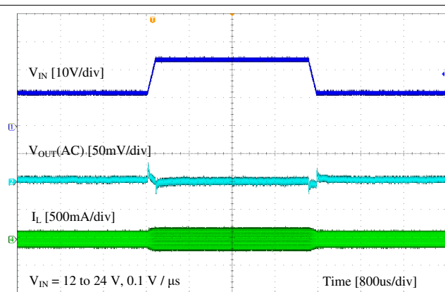
图 8-8. Line Transient
