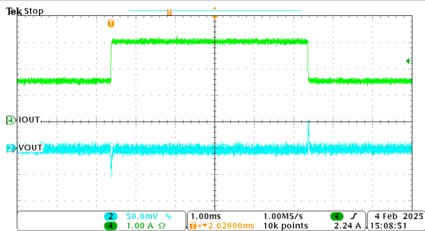
器件类型 = 3A 3.3V 固定输出 模式 = FPWM F_{SW} = 2\text{MHz}
