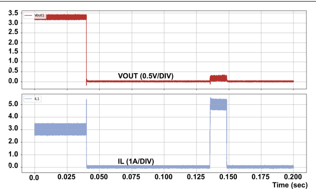
器件类型 = 3A 3.3V 固定输出 模式 = FPWM F_{SW} = 2\text{MHz}
