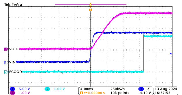
器件类型 = 3A 3.3V 固定输出 模式 = 自动 F_{SW} = 2\text{MHz}
