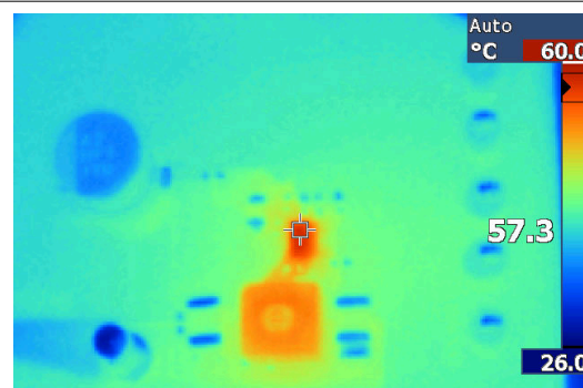
图 8-17. 热性能
