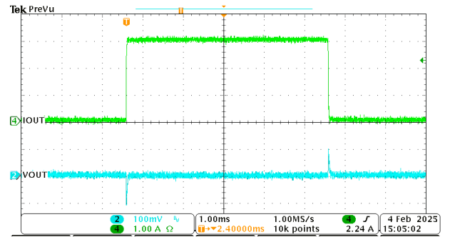
器件类型 = 3A 3.3V 固定输出 模式 = FPWM F_{SW} = 2\text{MHz}
