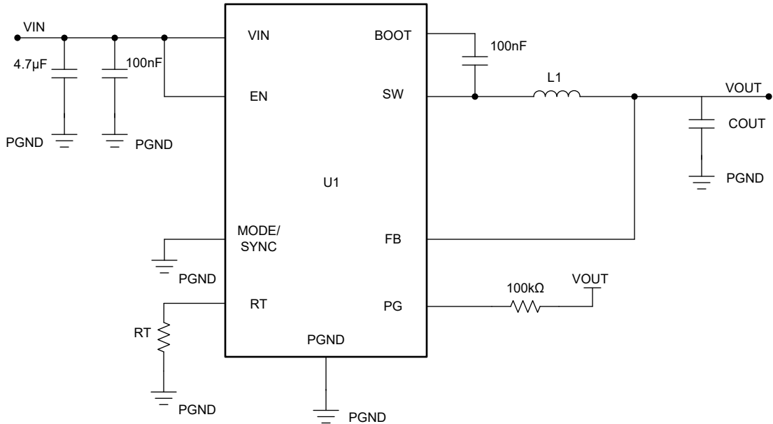
图 8-25. 应用电路示例
