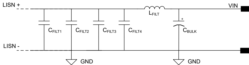
图 8-24. 典型输入 EMI 滤波器原理图
