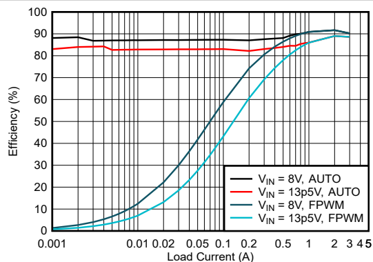
器件类型 = 3A 3.3V 固定输出 模式 = 自动/FPWM F_{SW} = 2MHz
