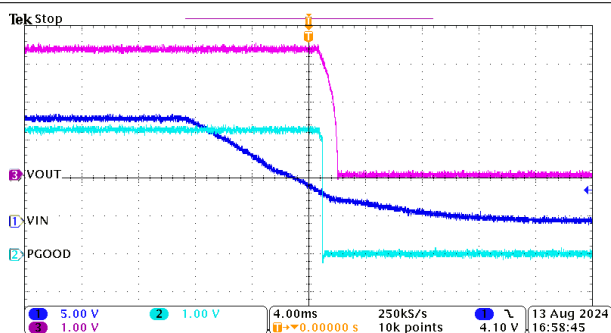
器件类型 = 3A 3.3V 固定输出 模式 = 自动 F_{SW} = 2\text{MHz}
