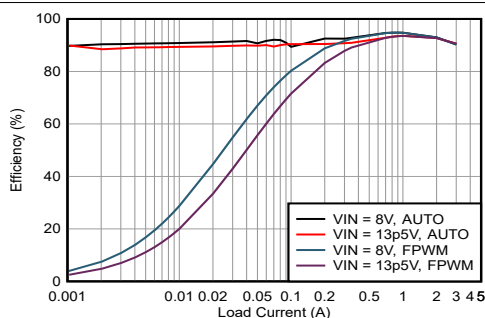
器件类型 = 3A 3.3V 固定输出 模式 = 自动/FPWM F_{SW} = 400kHz
