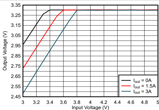
器件类型 = 3A 3.3V 固定输出 模式 = FPWM F_{SW} = 2MHz
