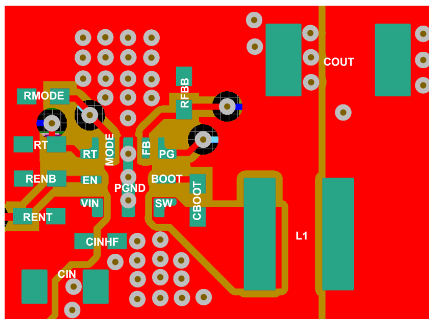
图 8-27. 固定输出版本
