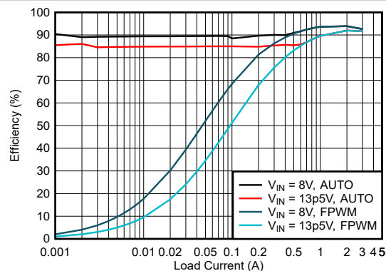
器件类型 = 3A 5V 固定输出 模式 = 自动/FPWM F_{SW} = 2MHz
