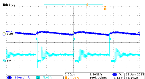
图 8-14. 短路恢复
