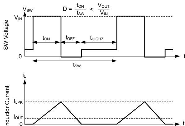
图 7-7. PFM 运行
