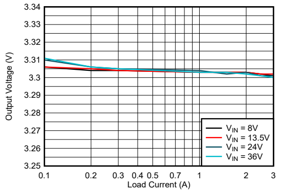
器件类型 = 3A 3.3V 固定输出 模式 = 自动 F_{SW} = 2\text{MHz}
