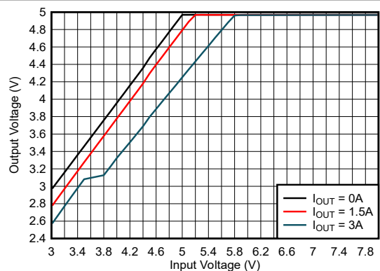
器件类型 = 3A 5V 固定输出 模式 = FPWM F_{SW} = 2MHz
