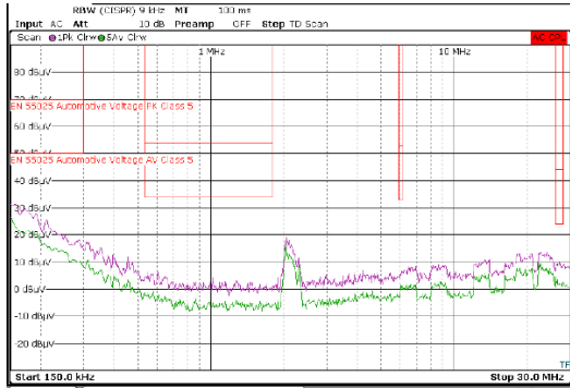
图 8-20. 传导 EMI 与 CISPR25 限值 (紫色：峰值信号，绿色：平均信号)，LMR60440QEVm
