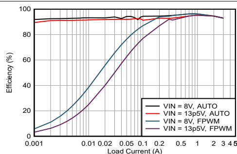
器件类型 = 3A 5V 固定输出 模式 = 自动/FPWM F_{SW} = 400kHz
