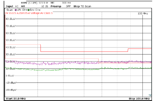
图 8-21. 传导 EMI 与 CISPR25 限值 (紫色：峰值信号，绿色：平均信号)，LMR60440QEVm
