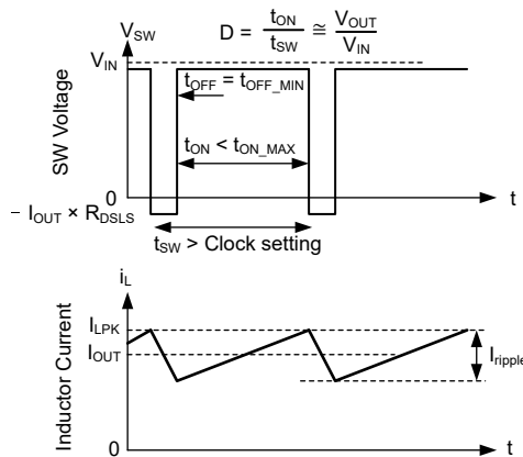
图 7-10. 压降波形
