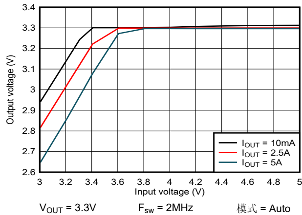
图 8-10. 压降曲线
