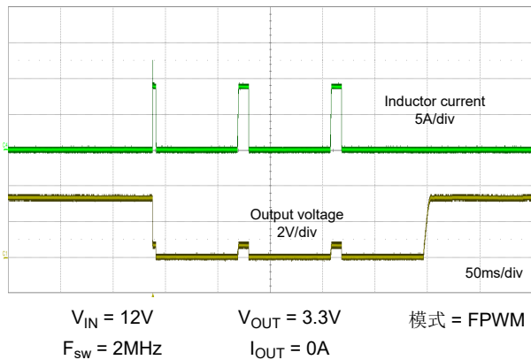
图 8-18. 短路行为
