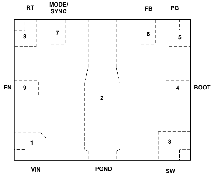
图 5-1. VBC 封装，9 引脚 WQFN-FCRLF ( 顶视图 )
