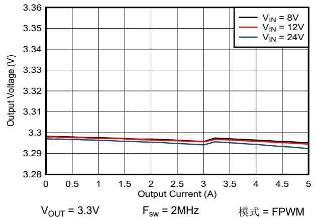
图 8-7. 负载和线路调节 - FPWM 模式
