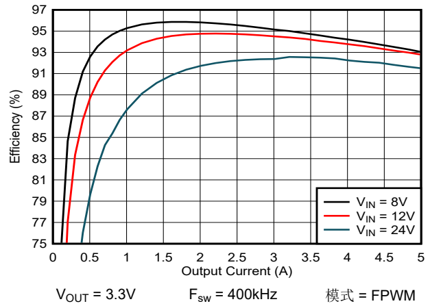
图 8-5. 效率 - FPWM 模式
