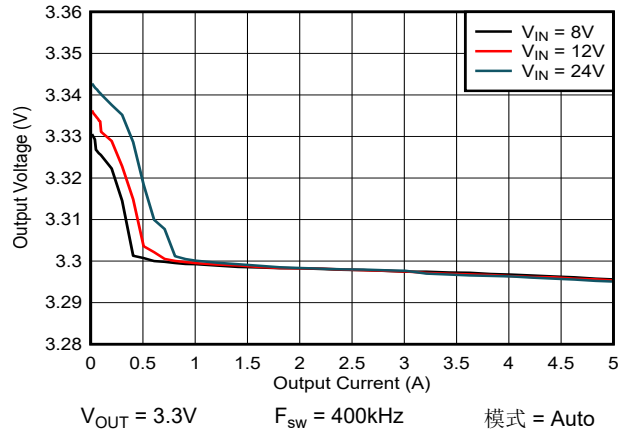
图 8-8. 负载和线路调节 - 自动模式
