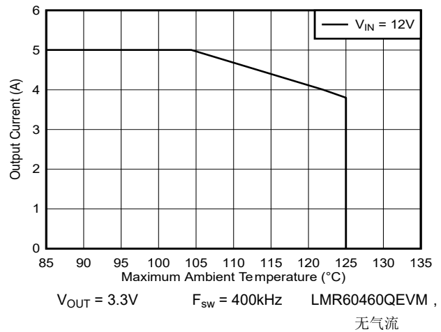
图 8-11. 输出电流与最大环境温度间的关系
