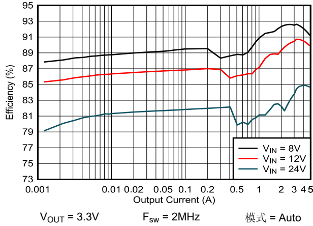
图 8-2. 效率 - 自动模式
