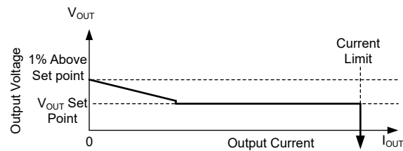
图 7-7. 自动模式下稳态输出电压与输出电流间的关系
