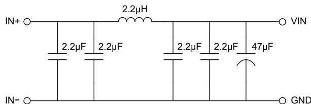
图 8-21. 推荐的输入 EMI 滤波器
