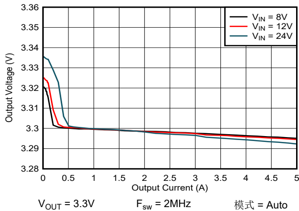
图 8-6. 负载和线路调节 - 自动模式
