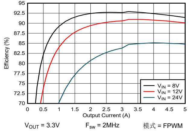
图 8-3. 效率 - FPWM 模式
