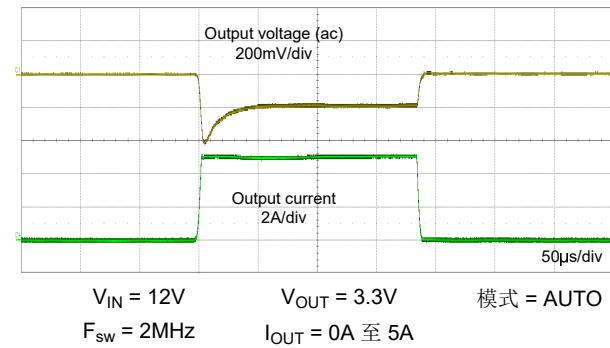
图 8-12. 负载瞬态
