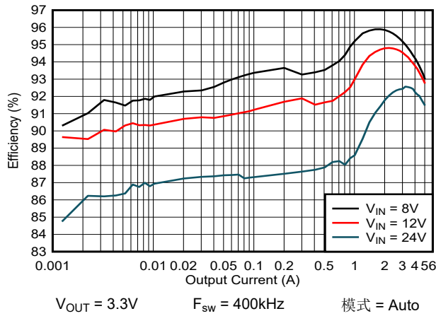
图 8-4. 效率 - 自动模式
