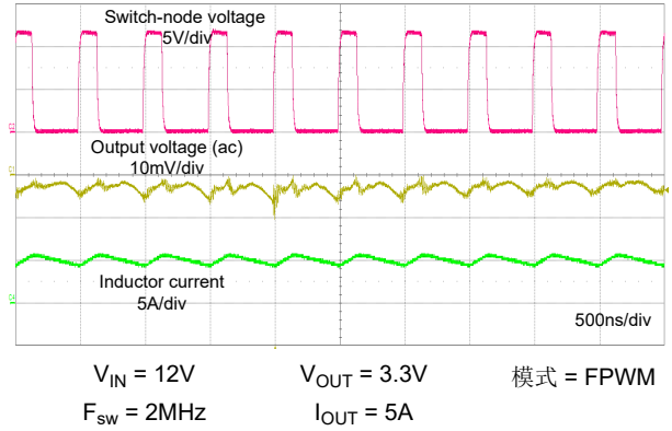
图 8-15. 稳态开关波形和输出电压纹波
