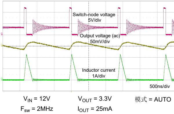
图 8-14. 稳态开关波形和输出电压纹波
