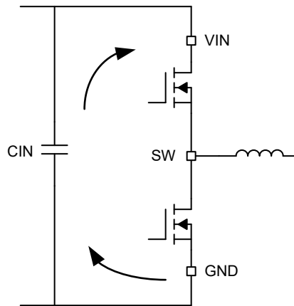
图 8-22. 具有快速边沿的电流环路
