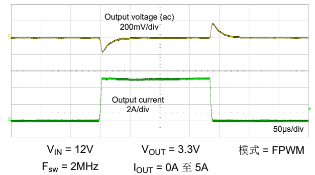
图 8-13. 负载瞬态
