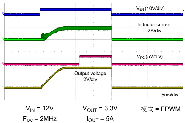
图 8-17. 在 5A 负载条件下实现启动和关断控制
