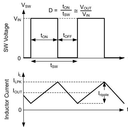
图 7-8. 连续导通模式 (CCM) 下的 SW 电压和电感器电流波形
