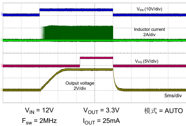
图 8-16. 在 50mA 负载条件下实现启动和关断控制
