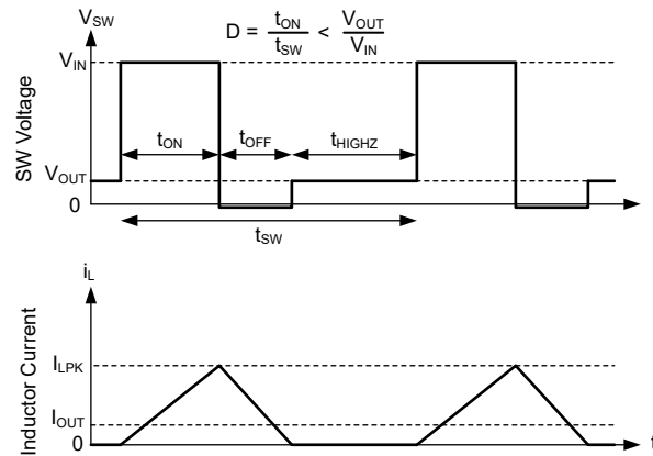
图 7-6. PFM 操作
