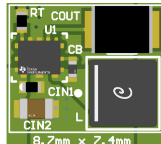
EVM 布局 - 2.2MHz 3.3V 固定输出
