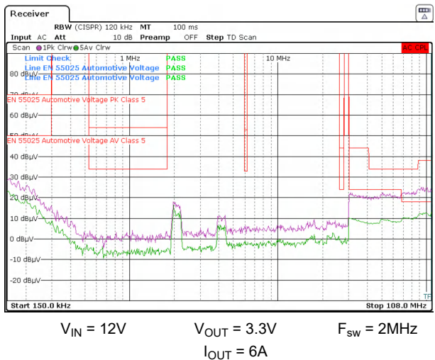
图 8-19. 传导 EMI 与 CISPR 25 限值 (粉色: 峰值信号, 绿色: 平均信号)
