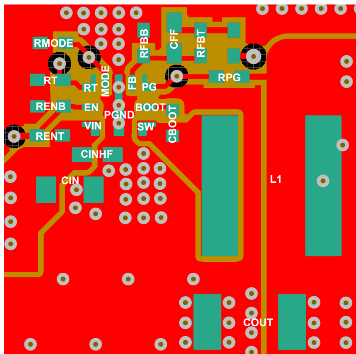
图 8-23. 可调节输出版本
