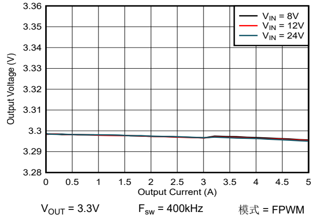
图 8-9. 负载和线路调节 - FPWM 模式
