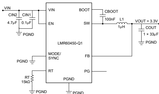
示例原理图 - 2.2MHz 3.3V 固定输出
