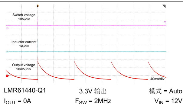
图 8-13. 稳态波形
