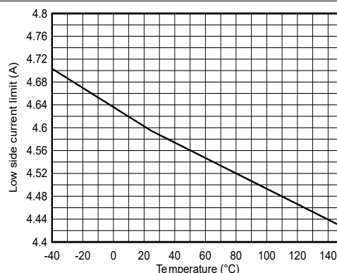
图 6-2. 低侧 MOSFET 电流限值
