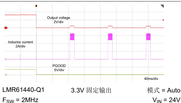
图 8-10. 应用短路
