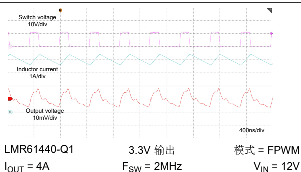
图 8-12. 稳态波形
