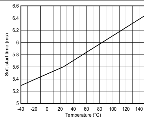
图 6-6. 软启动时间
