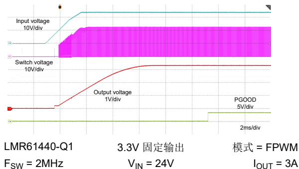
图 8-8. 启动运行
