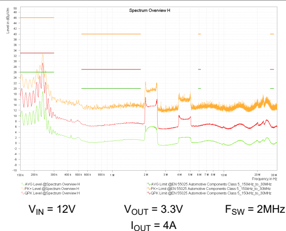
图 8-15. 辐射 EMI (单极) 与 CISPR 25 限值对比
