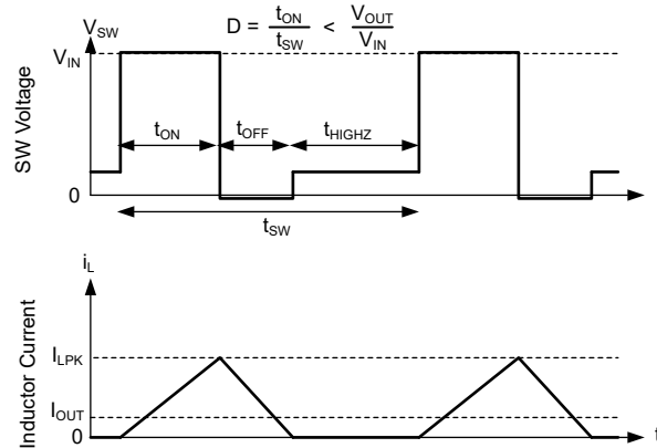
图 7-7. PFM 操作
