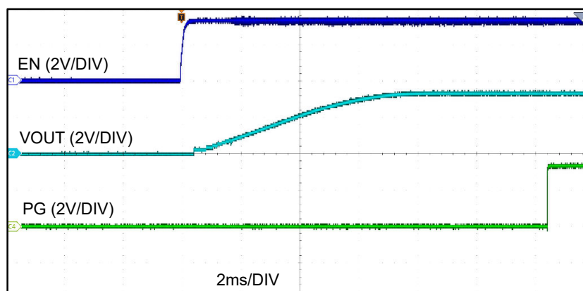
图 7-2. 使能软启动
