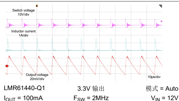
图 8-11. 稳态波形
