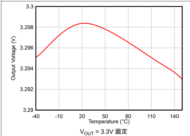
图 6-3. 输出电压精度与温度间的关系
