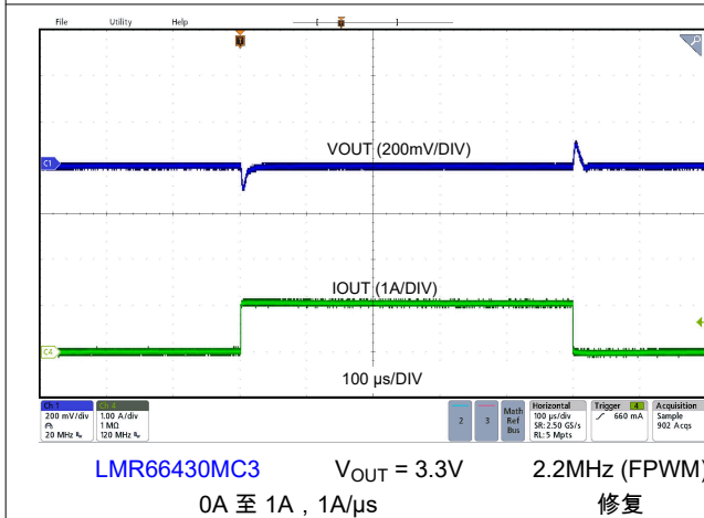
图 8-12. 负载瞬态
