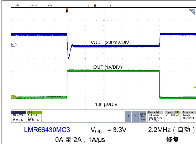
图 8-10. 负载瞬态
