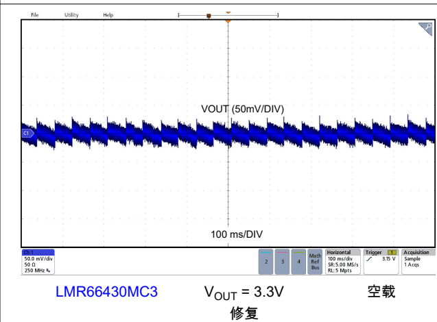
图 8-15. 输出电压纹波
