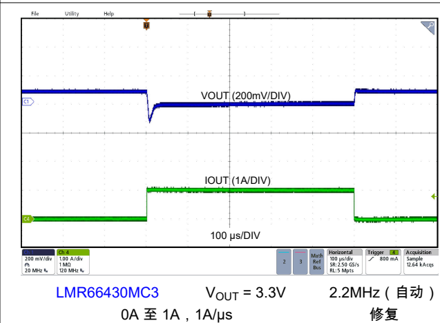
图 8-13. 负载瞬态
