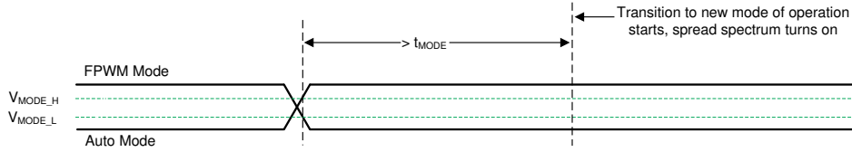
图 7-4. 自动模式和 FPWM 模式之间的转换
