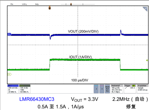
图 8-11. 负载瞬态
