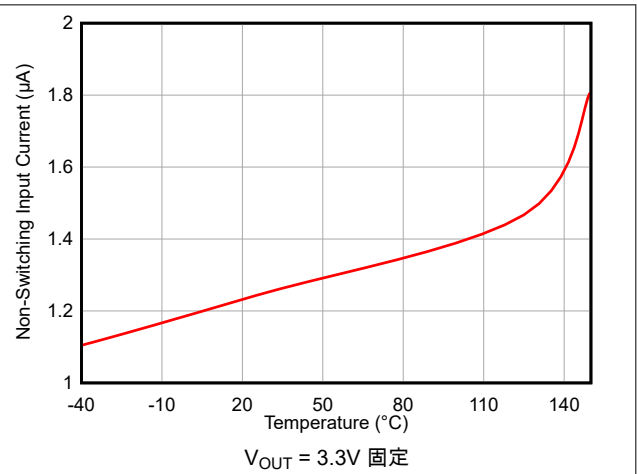
图 6-2. 非开关输入电流 ( I_{QVIN(nonsw)} ) 与温度间的关系
