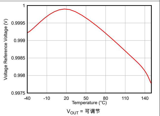
图 6-4. 反馈电压精度与温度间的关系
